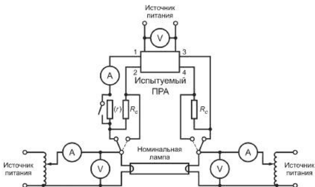
Рисунок А.8 — Схема измерений максимального тока в любом вводе электрода
