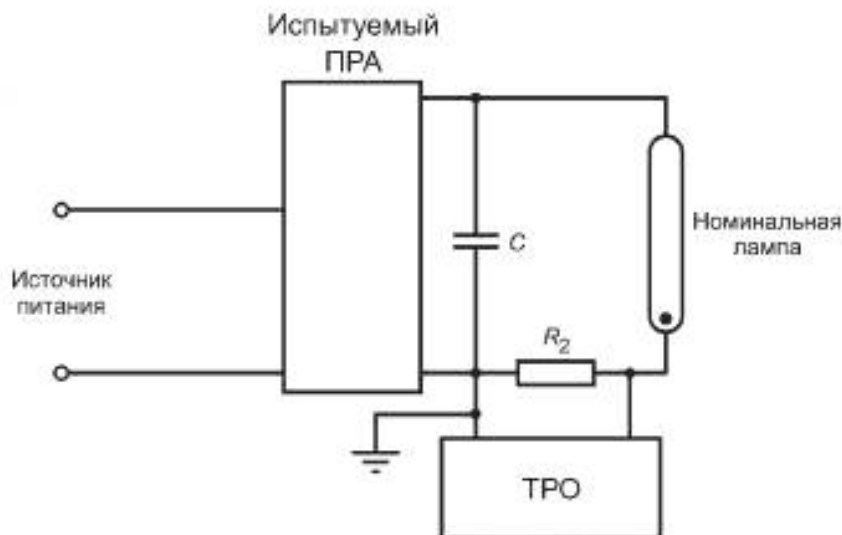
Рисунок А.9 — Схема измерений формы кривой тока
