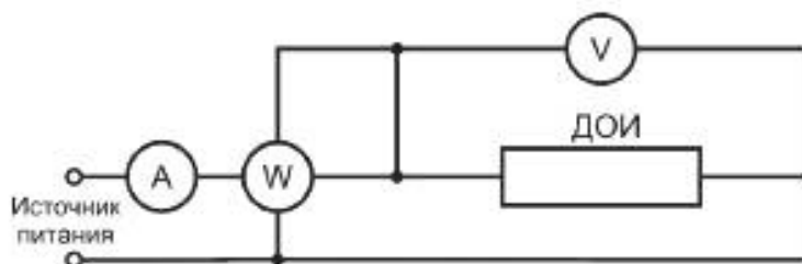
Рисунок А.2 — Схема для измерения коэффициента мощности
