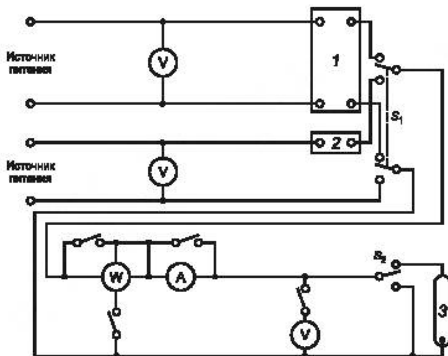
1 — испытуемый ПРА; 2 — ДОО; 3 — номинальная лампа
