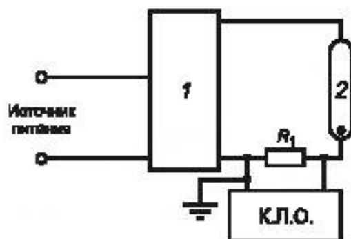
1 — испытуемый ПРА; 2 — номинальная лампа; К.Л.О. — осциллограф
