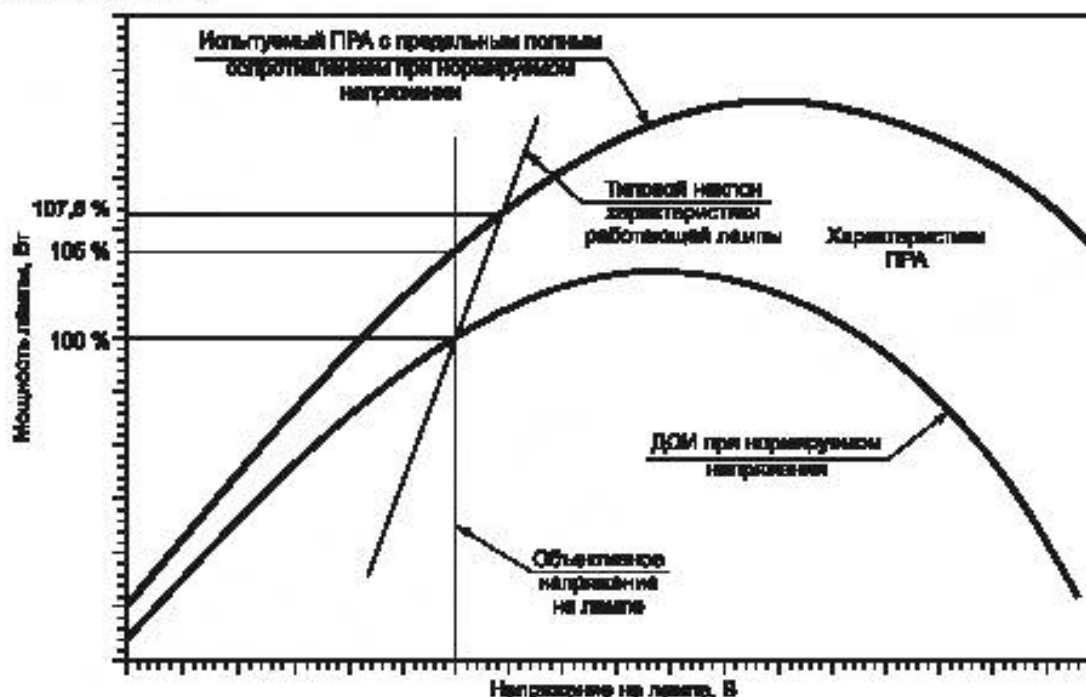
Рисунок D.1 — Характеристики соответствия настройки ПРА для натриевой лампы высокого давления, работающей с ДОО и испытуемым ПРА при номинальном напряжении питания
