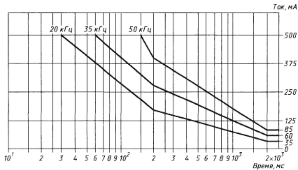
Рисунок 3 — Пределы емкостного тока утечки для трубочатой люминесцентной лампы, работающей на высокой частоте
