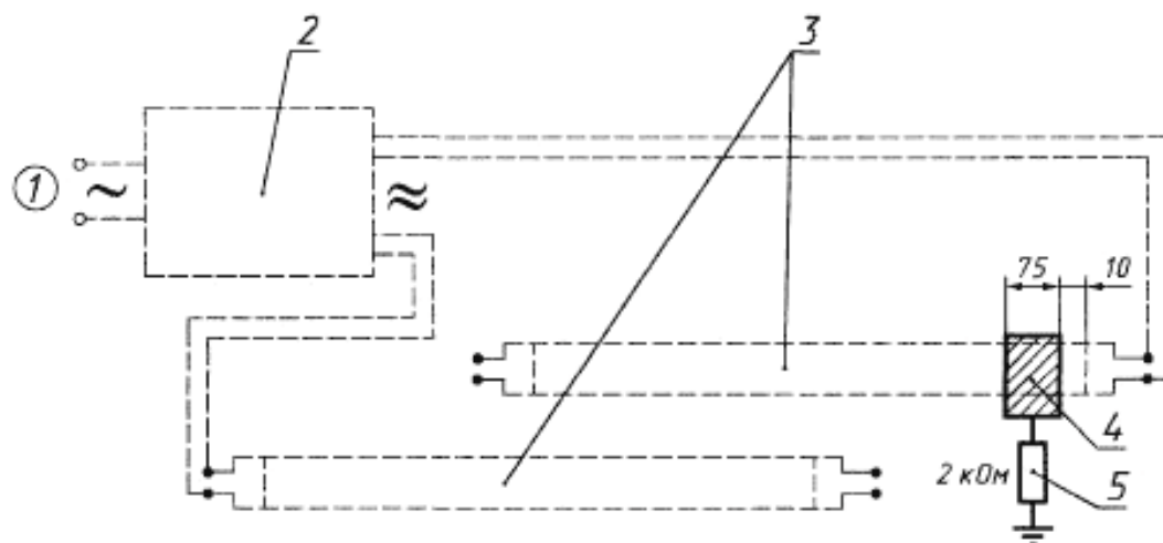
Рисунок 3 — Пределы емкостного тока утечки для трубочатой люминесцентной лампы, работающей на высокой частоте
