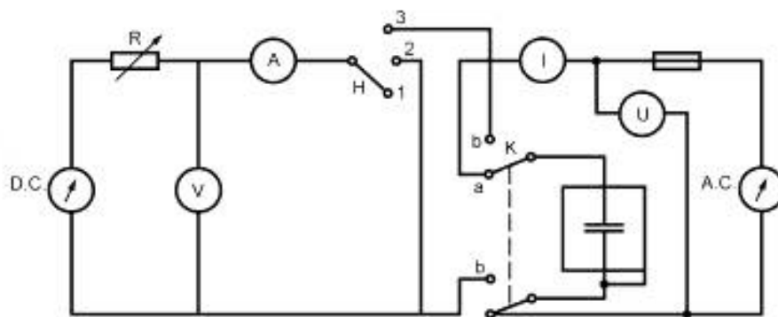
Рисунок 1 — Электрическая схема для выполнения испытания на разрушение
