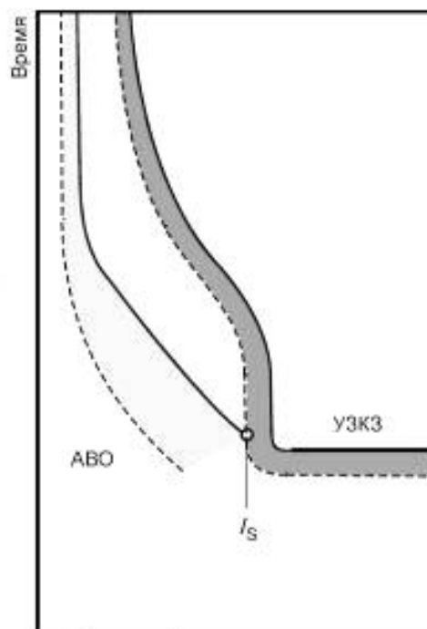
Ожидаемый ток короткого замыкания
