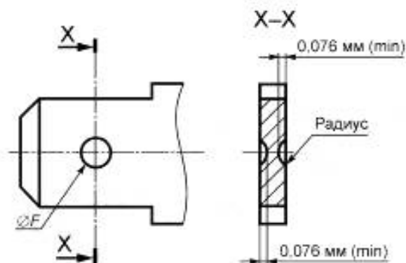
Рисунок Е.7 — Размеры круглых углублений фиксации (см. рисунок Е.6)
