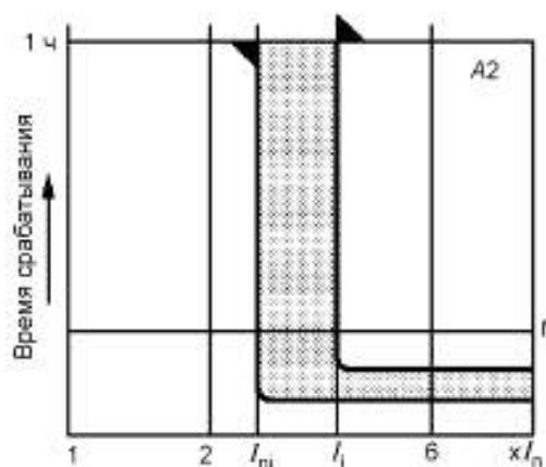
Рисунок А.2 — Характеристика только электромагнитной защиты
