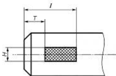
Рисунок E.10 — Размеры штыревого наконечника
