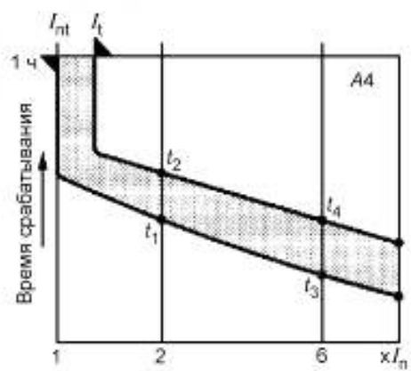
Рисунок А.4 — Характеристика гидравлическо-электромагнитной защиты
