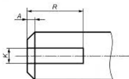
Рисунок E.12 — Размеры штыревого наконечника
