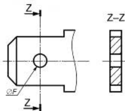
Рисунок Е.8 — Размеры прямоугольных элементов фиксации (см. рисунок Е.6)
