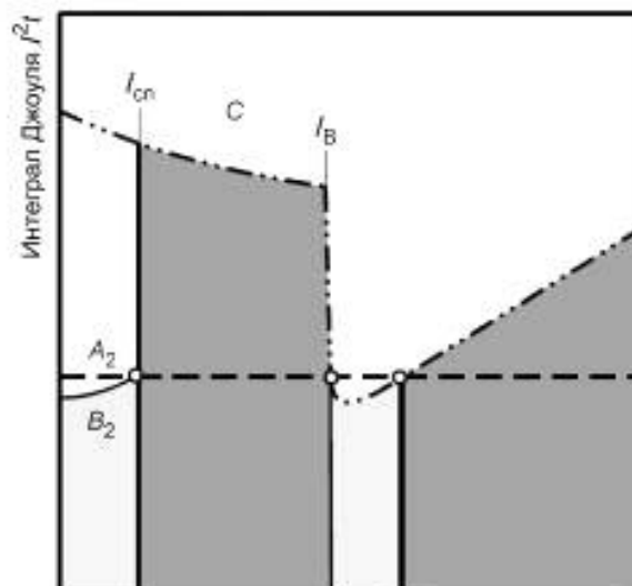
Рисунок F.8b — Ненадлежащая координация
