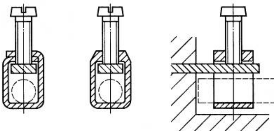
Выводы с хомутиком
