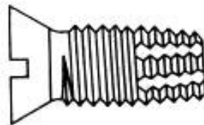
Рисунок 2 — Самонарезающий режущий винт
