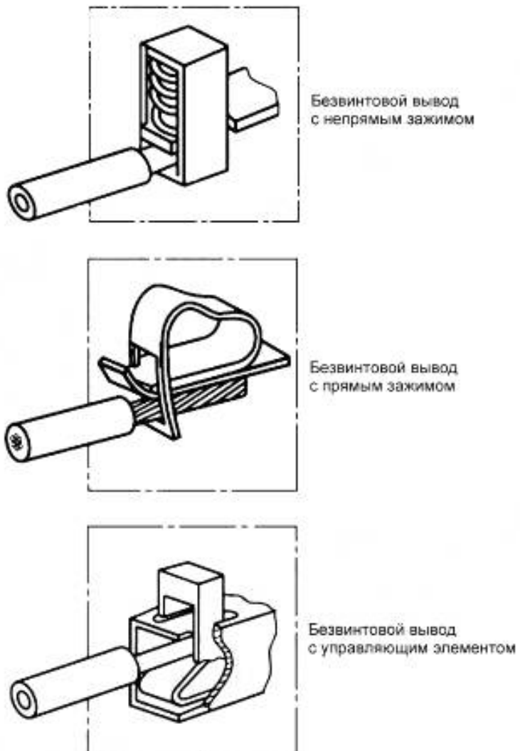
Рисунок Е.5 — Примеры безрезьбовых выводов
