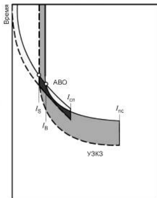
Ожидаемый ток короткого замыкания
