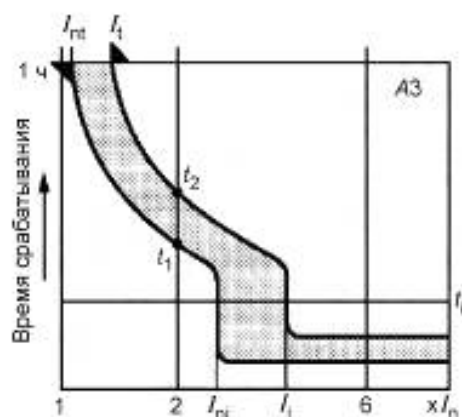
Рисунок А.3 — Характеристика тепловой и электромагнитной защиты
