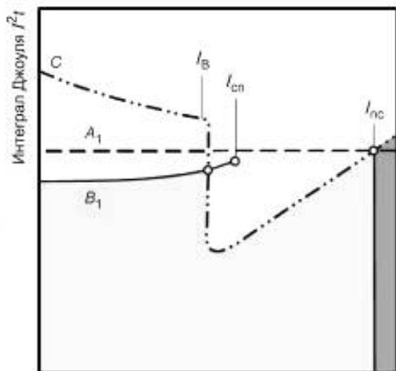
Рисунок F.8a — Надлежащая координация
