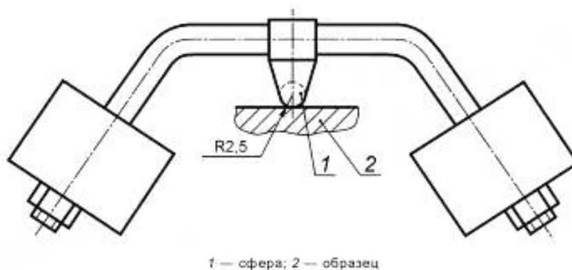
Рисунок 8 — Установка для испытаний давлением шарика
