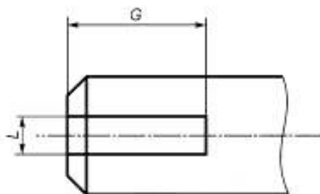
Рисунок E.11 — Размеры штыревого наконечника
