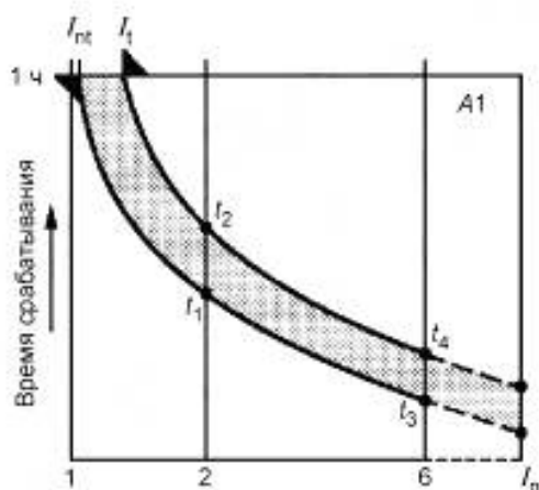
Рисунок А.1 — Характеристика только тепловой защиты
