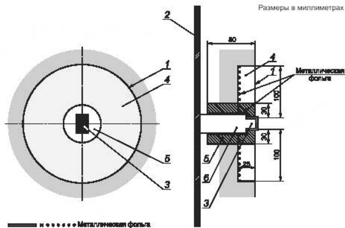
Рисунок R.1 — Механизм управления снаружи оболочки
