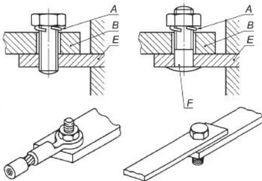
Рисунок D.4 — Зажимы со скобой
