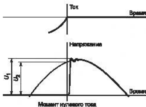
Рисунок 7 — Схема возвращающегося напряжения на контактах первой отключаемой фазы в идеальных условиях [см. 8.3.3.5.2, перечисление в)]
