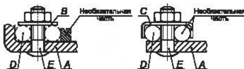
Рисунок D.2 — Зажимы с отверстиями
