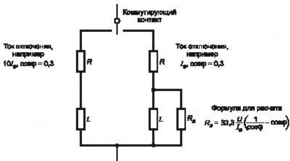
Рисунок 7 — Схема нагрузки L_2 для условий испытаний, требующих различных значений токов включения и отключения и (или) коэффициента мощности (постоянной времени)
