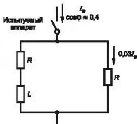
Рисунок С.2 — Упрощенная схема (см. С.3.2.1)
