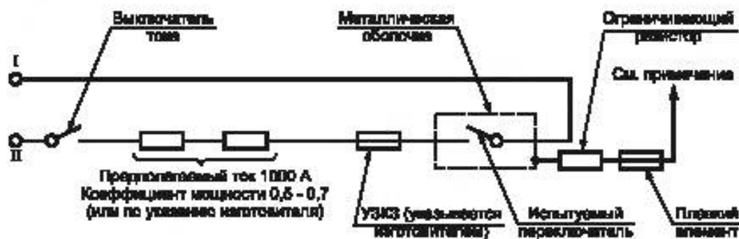
Рисунок 7 — Схема нагрузки L_2 для условий испытаний, требующих различных значений токов включения и отключения и (или) коэффициента мощности (постоянной времени)
