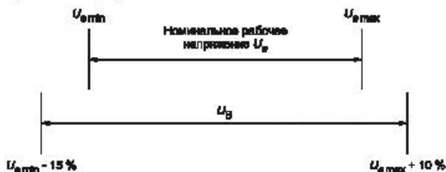
Рисунок Н.1 — Соотношение между U_n и U_B
