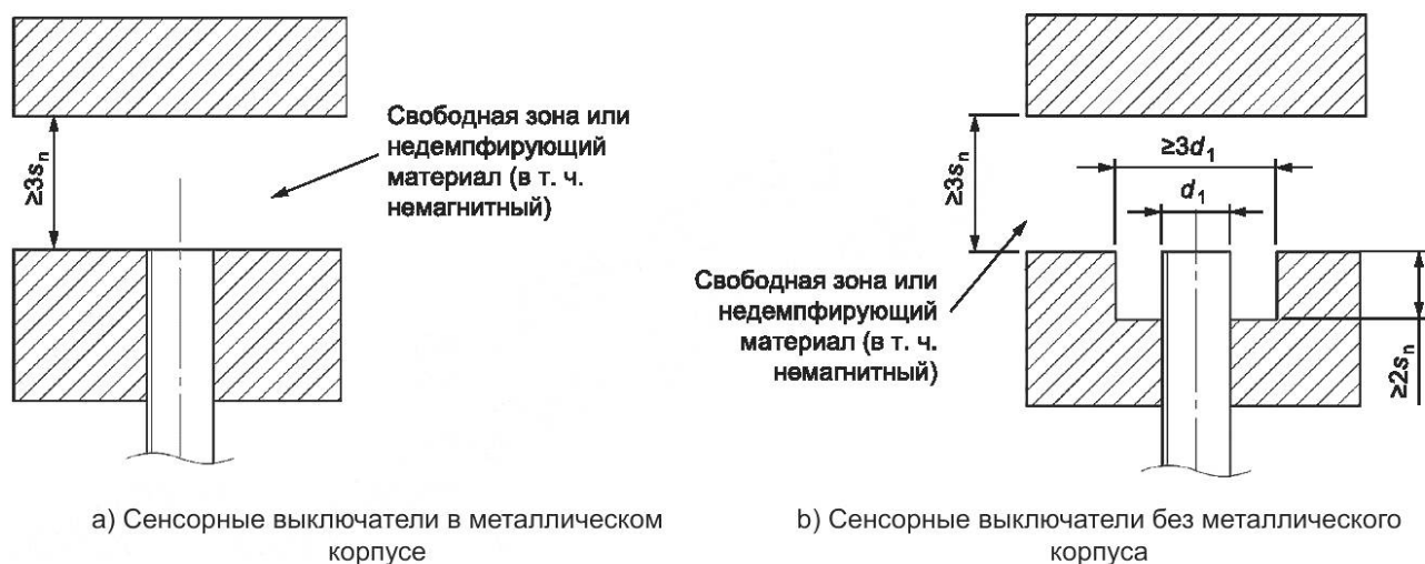
Рисунок А.6 — (IA, IB) Установка (монтаж) а
