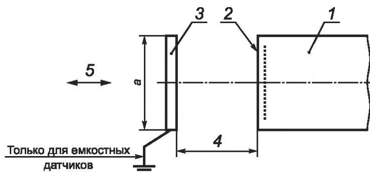
1 — сенсорный выключатель; 2 — чувствительная поверхность; 3 — цель; 4 — расстояние дальности действия; 5 — направление движения; a — длина стороны цели
