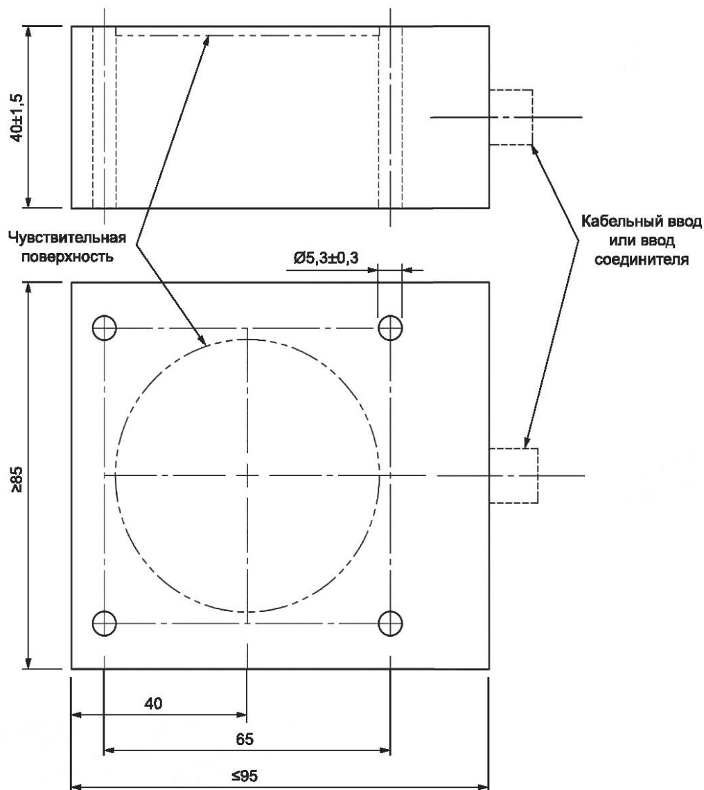
Рисунок А.13 — (IDC) Габаритные размеры
