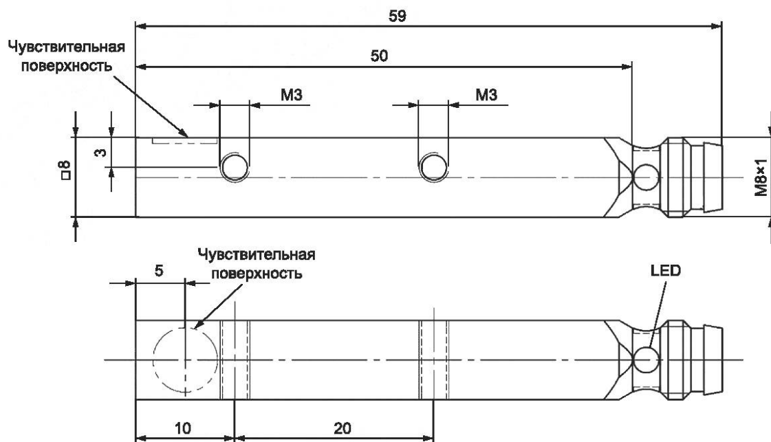
Рисунок А.20 — Сенсорные выключатели кубической формы размером 8 × 8 мм с соединителем M8
