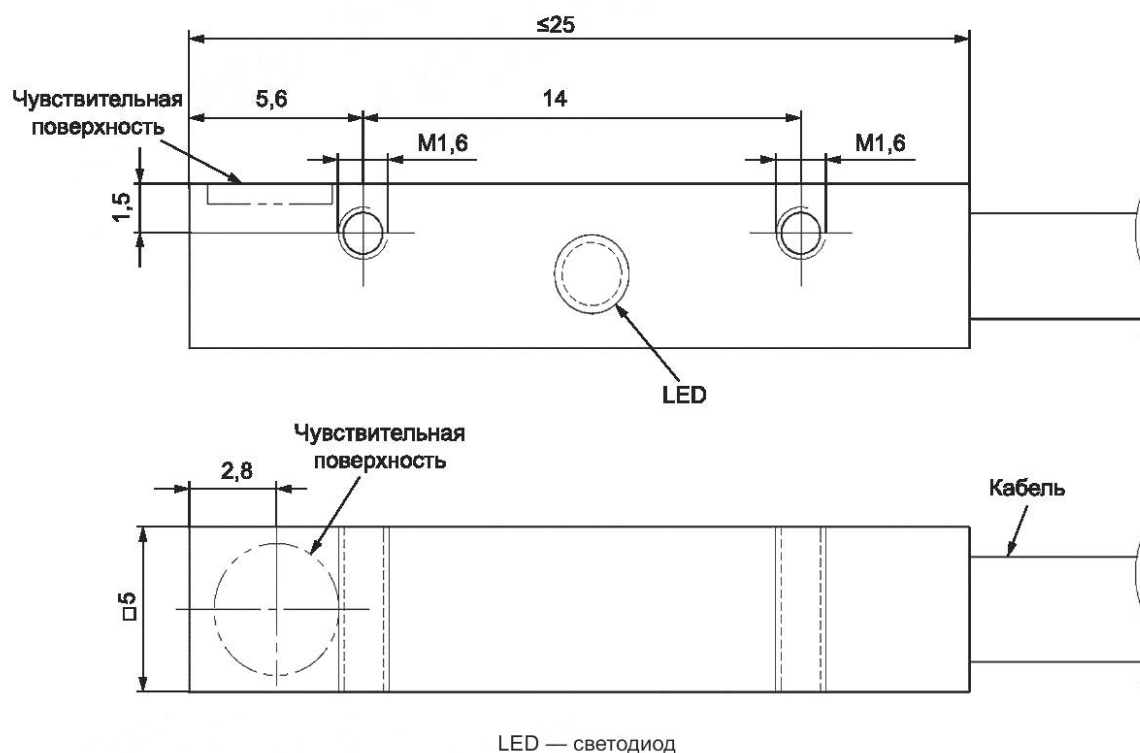
Рисунок А.18 — Сенсорные выключатели кубической формы размером 5 × 5 мм с кабелем
