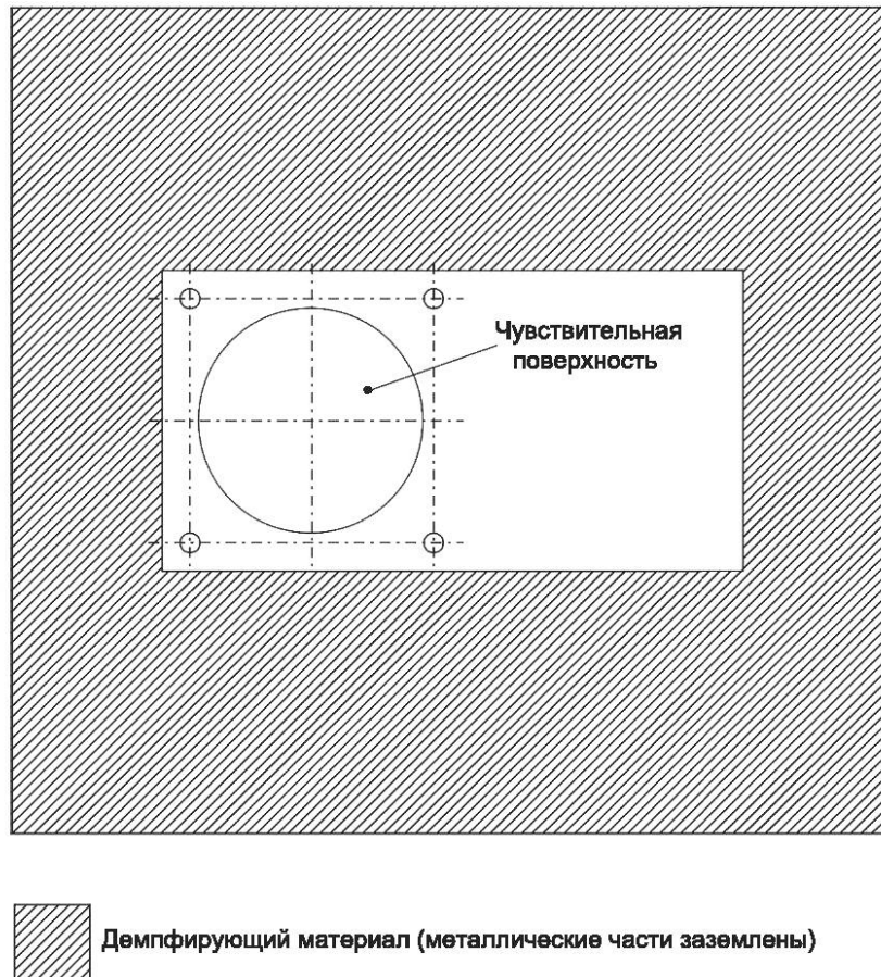
Рисунок А.26 — (CD) Установка (монтаж)
