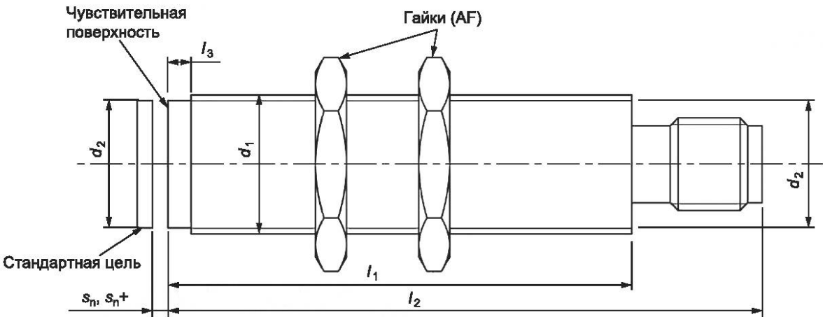
Рисунок А.3 — Габаритные размеры типа А — Корпус M5 × 0,5, M8 × 1, Ø 4, Ø 6,5 с соединителем M5/M8
