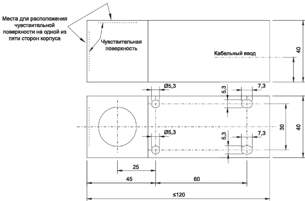
б) Габаритные размеры сенсорного выключателя типа С40
