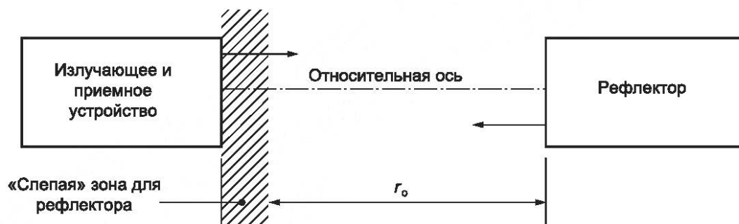
б) Тип R, прямо-излучающее устройство и рефлектор. Ретрорефлекторный фотоэлектрический сенсорный выключатель
