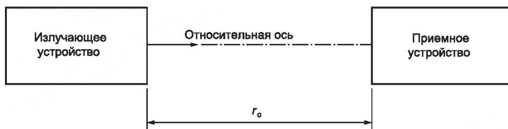
а) Тип Т, излучающее и приемное устройство. Барьерный фотоэлектрический сенсорный выключатель
