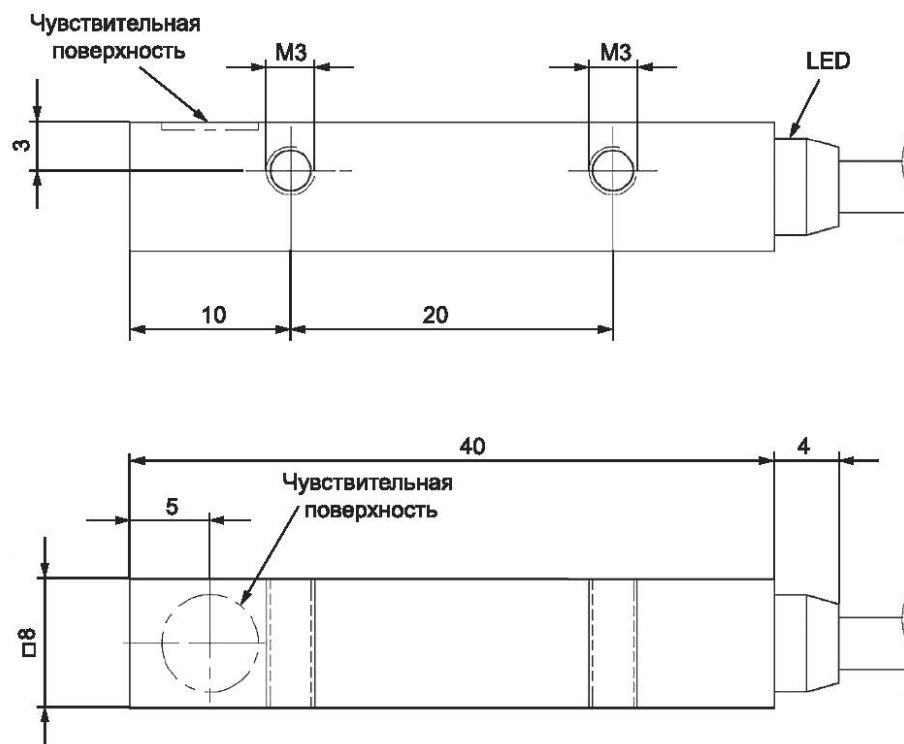
Рисунок А.19 — Сенсорные выключатели кубической формы размером 8 × 8 мм с кабелем
