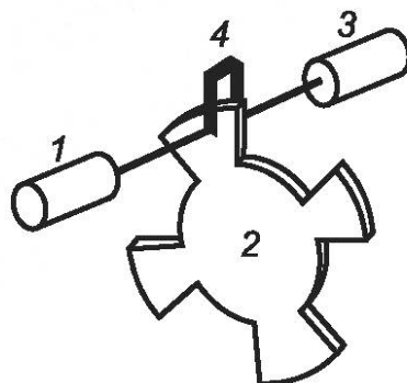
а) Сенсорный выключатель типа Т (сквозной луч)
