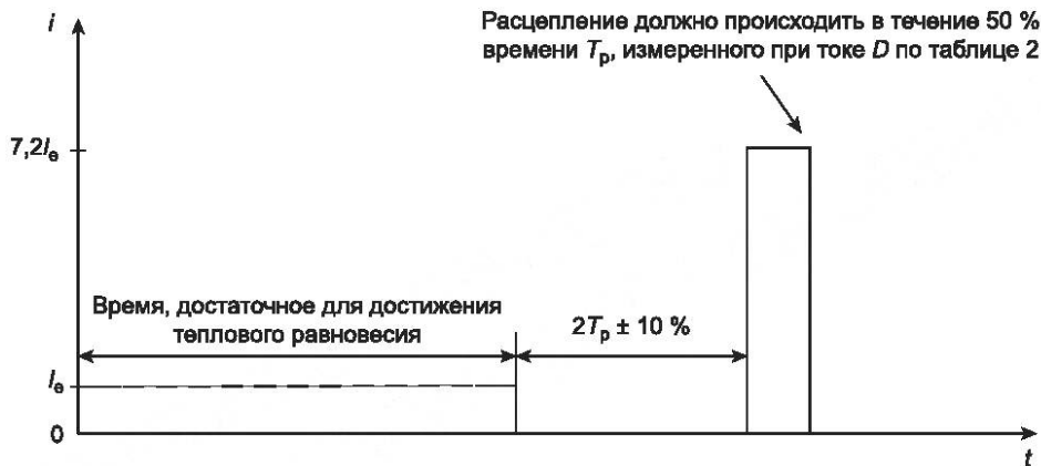
Рисунок 2 — Испытание тепловой памяти
