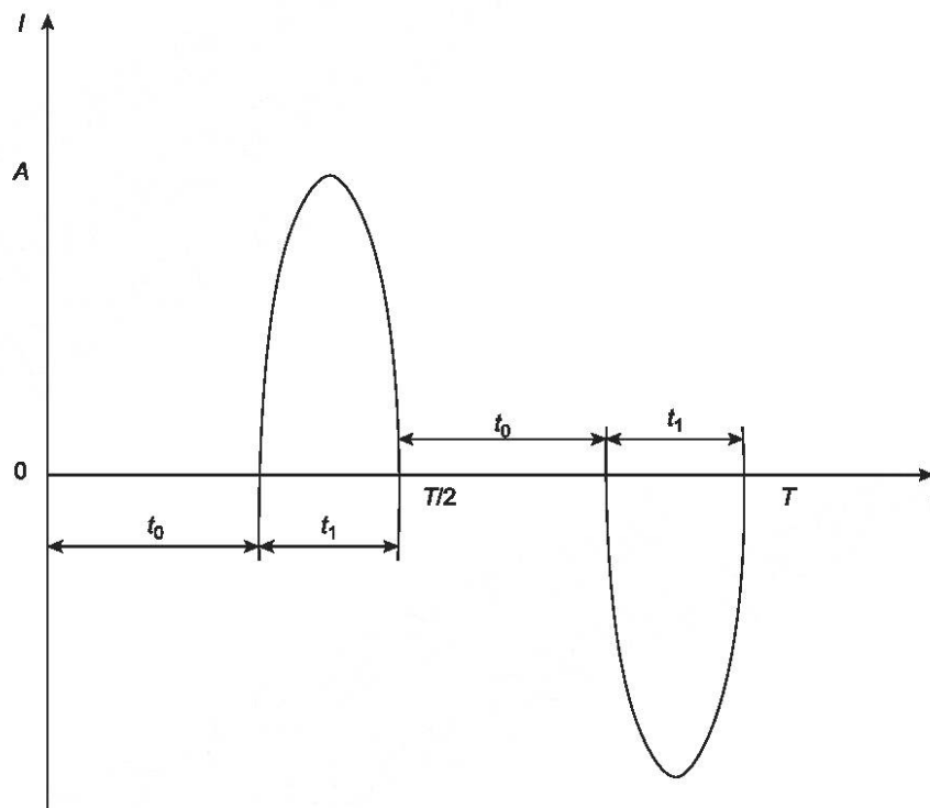
А — максимальный ток; Т — период; t_1 — продолжительность каждого полупериода; t_0 — время задержки
