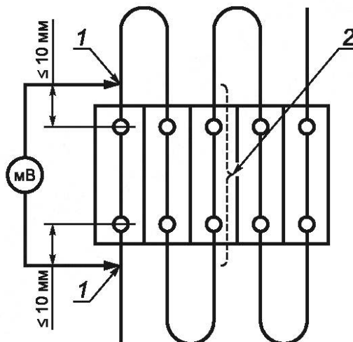
1 — места измерения падения напряжения; 2 — места измерения температуры
