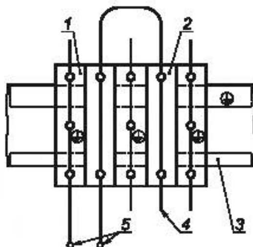
1 — клеммная колодка защитных проводников; 2 — клеммная колодка; 3 — рейка крепления; 4 — концы проводников; 5 — прикладываемое напряжение
