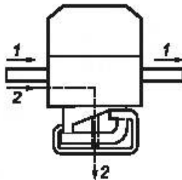
Рисунок 5 — Схема испытания на тепловой кратковременный ток
