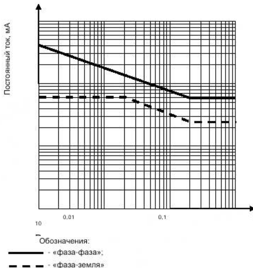
Рисунок 1 – Максимальный ток после единичной неисправности
