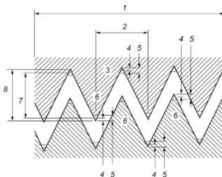
1 — внутренняя резьба; 2 — шаг; 3 — впадина; 4 — минимальный срез; 5 — максимальный срез; 6 — вершина; 7 — максимальная высота профиля резьбы; 8 — высота исходного треугольника резьбы
