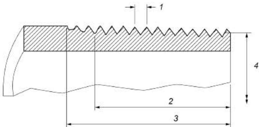
1 — шаг (p); 2 — эффективная длина резьбы; 3 — полная длина резьбы; 4 — средний диаметр на конце резьбы E_0
