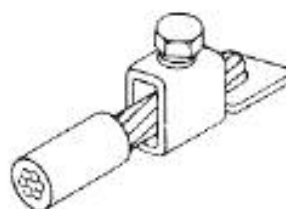
ф) винтовые зажимы с непосредственным давлением
