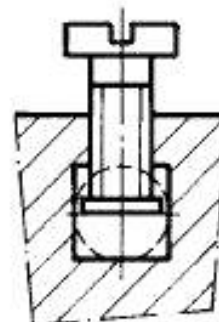
с) с прижимной пластиной
