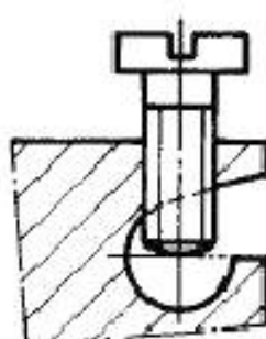
б) винтовой зажим с непосредственным давлением
