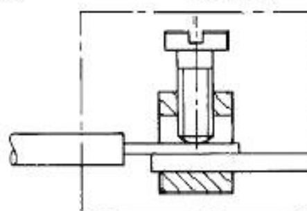
е) винтовой зажим с непосредственным давлением
