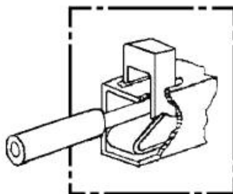
с) безвинтовой зажим с управляющим элементом
