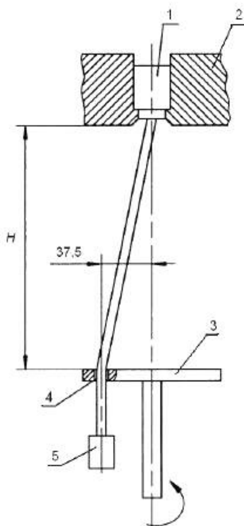
1 — испытуемый зажим; 2 — крепление; 3 — плата; 4 — втулка; 5 — груз
