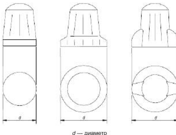
Рисунок 101 – Размер захвата
