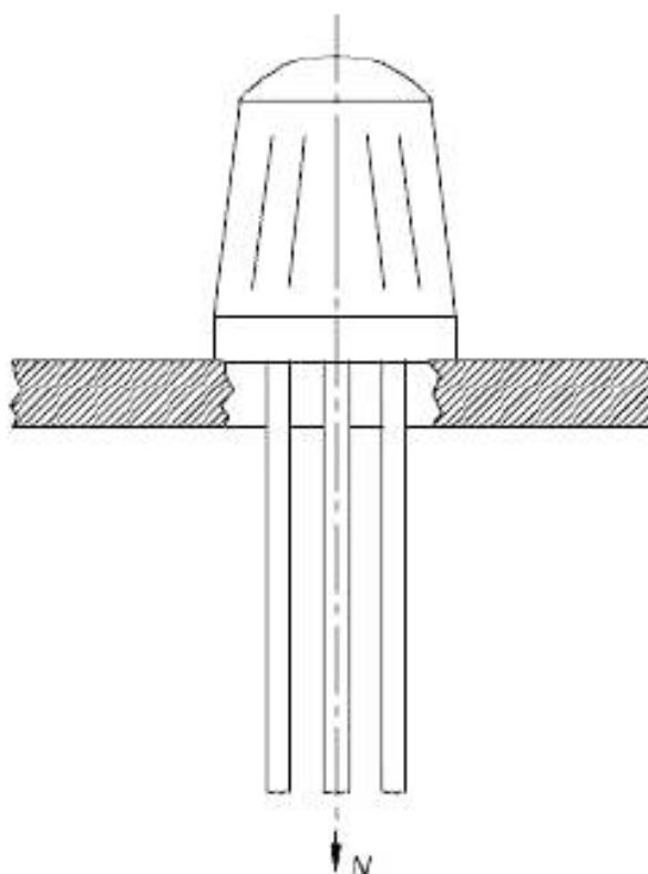
Рисунок 103 – Пример приложения тянущего усилия вдоль оси УСС
