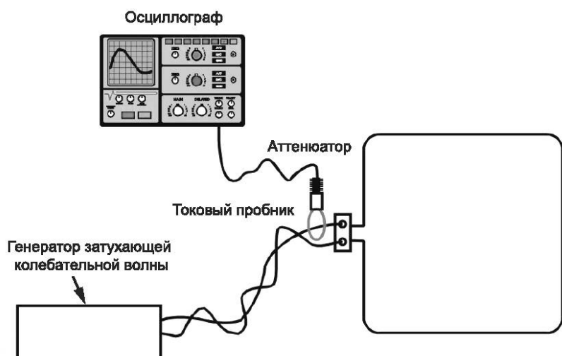
Рисунок 4 — Пример измерения тока стандартной индукционной катушки
