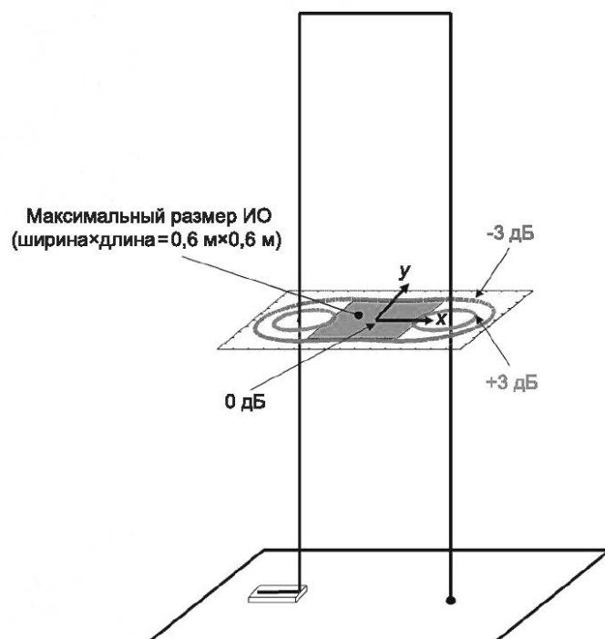
Рисунок А.5 — Изолинии +3 дБ и -3 дБ напряженности магнитного поля (предельные значения) в плоскости x — y для индукционной катушки размером 1 м \times 2,6 м с опорной пластиной заземления
