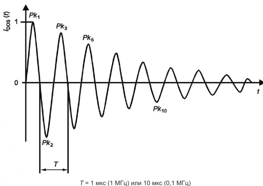
Рисунок 2 — Форма сигнала тока короткого замыкания в стандартных катушках
