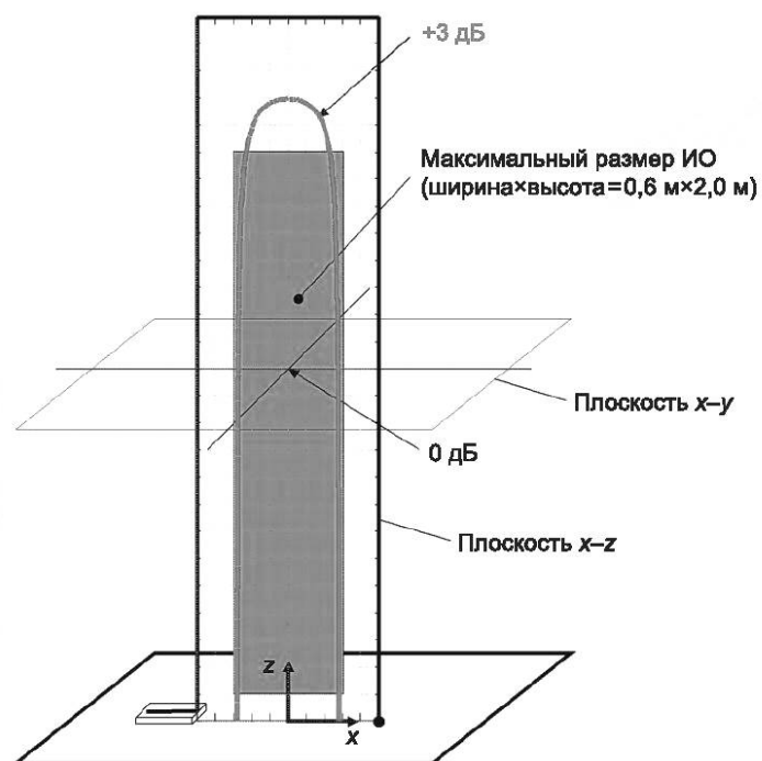
Рисунок А.4 — Изолиния +3 дБ напряженности магнитного поля (предельные значения) в плоскости x — z для индукционной катушки размером 1 м \times 2,6 м с опорной пластиной заземления
