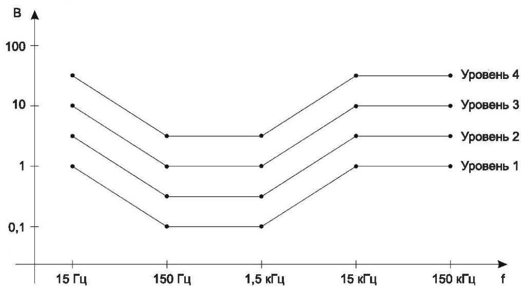
Рисунок 2 — Зависимость испытательного напряжения от частоты
