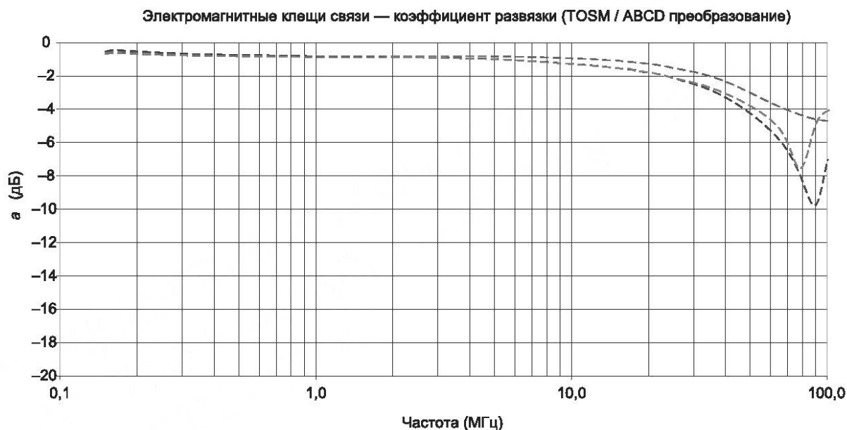
Рисунок А.8 — Типовые примеры коэффициентов развязки, три типовых представителя клещей связи
