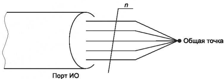
а) Определение общей точки при использовании неэкранированных кабелей
