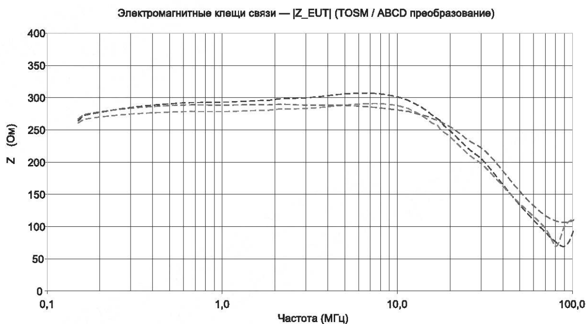
Рисунок А.7 — Типовые примеры полного сопротивления клещей связи, три типовых представителя клещей связи
