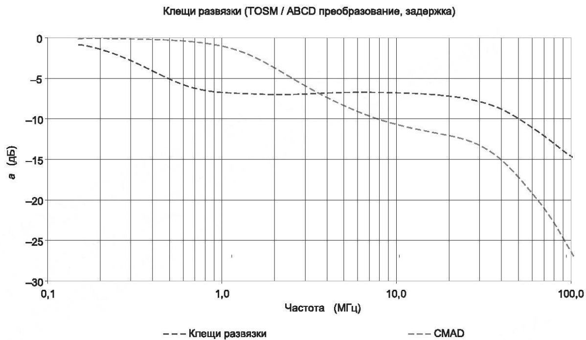
Рисунок А.14 — Типовые примеры коэффициентов развязки
