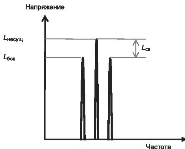
Рисунок J.4 — Спектр AM модулированного сигнала
