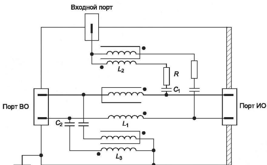
Рисунок D.3 — Пример упрощенной схемы УСП типа CDN-AF2, применяемого при вводе помехи в неэкранированные несимметричные линии (см. 6.2.2.4)
