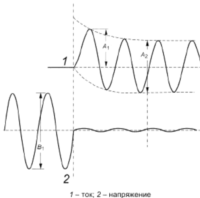
Рисунок 13 – Пример калибровочной записи для испытания в условиях короткого замыкания
