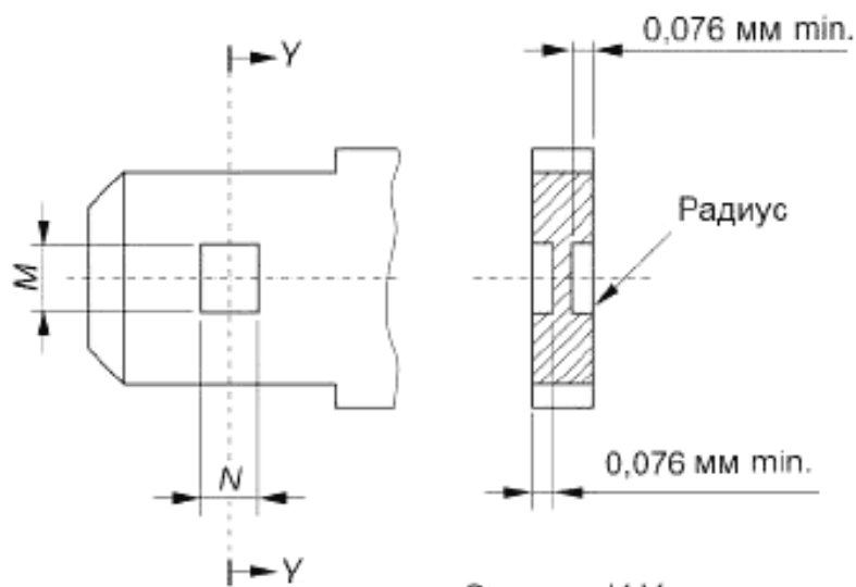
Сечение Y-Y
