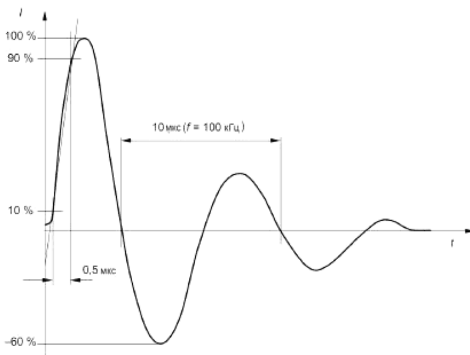
Рисунок 26 – Ток звенящей волны 0,5 мкс/100 кГц
