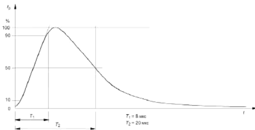
Рисунок 28 – Импульс тока 8/20 мкс
