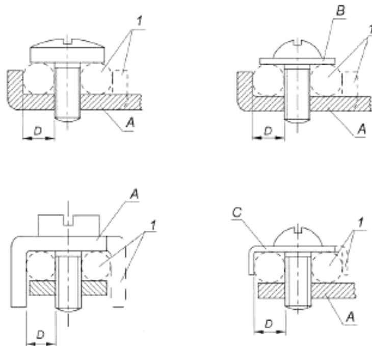
Рисунок IC.2а – Винтовые выводы
