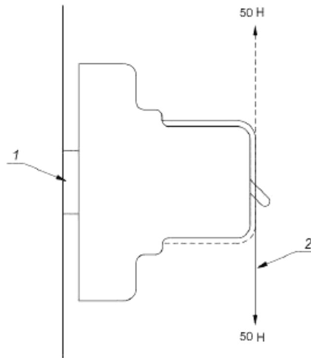
1 – рейка; 2 – шнур
