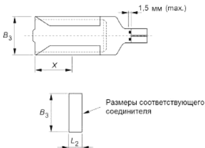
Рисунок К.5 – Размеры отверстий для фиксации
