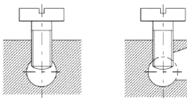
Рисунок IC.1b – Выводы без прижимных пластин
