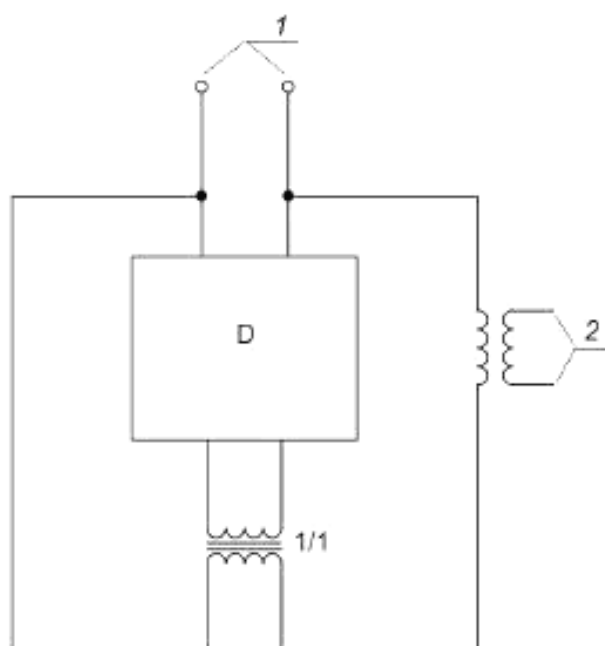
D – испытуемый АВДТ; 1 – источник напряжения 1,1U_{н} ; 2 – источник тока
