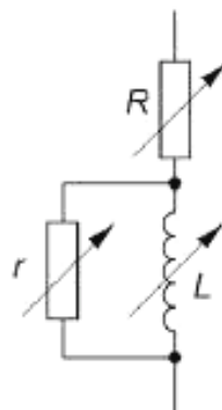
Рисунок 9 – Фрагмент полных сопротивлений Z , Z_1 и Z_2
