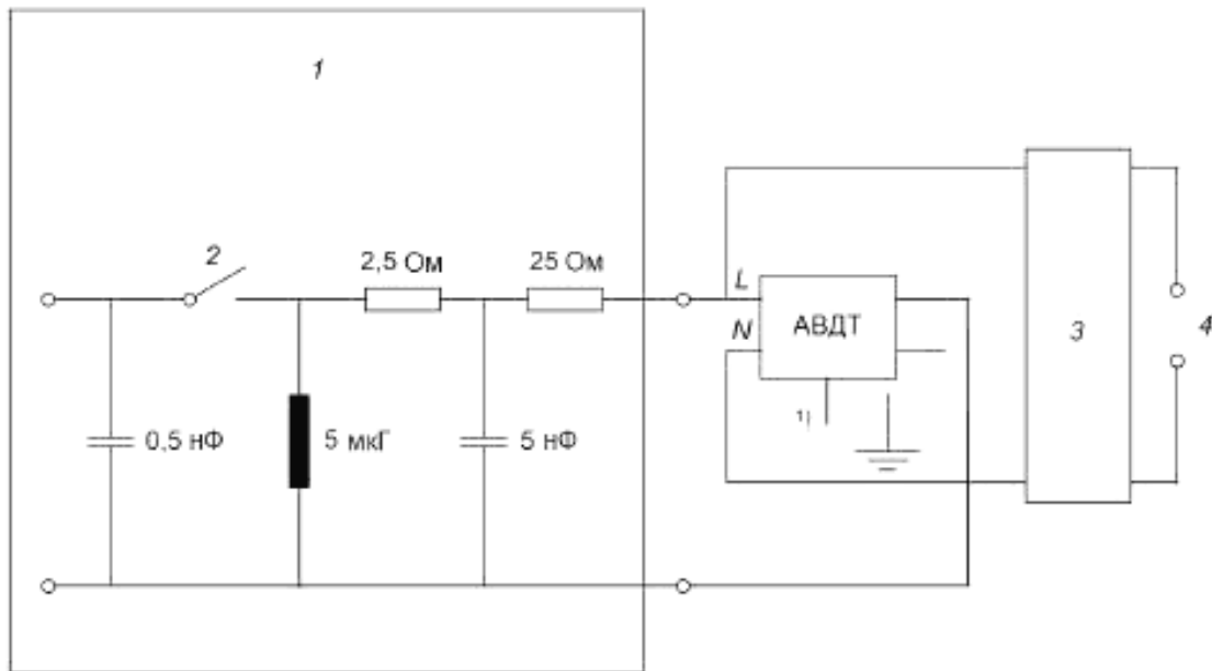
1 – генератор затухания колебаний волны 0,5 мкс/100 кГц; 2 – триггер; 3 – фильтр; 4 – источник питания
