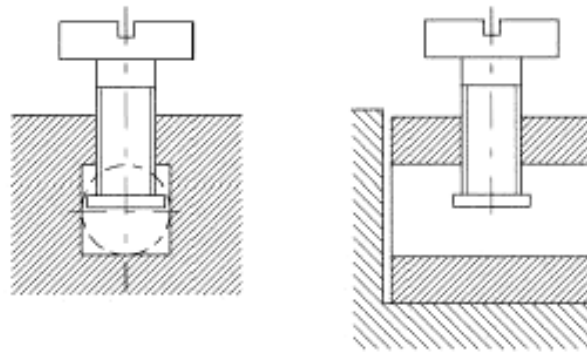
Рисунок IC.1с – Выводы с прижимными пластинами
