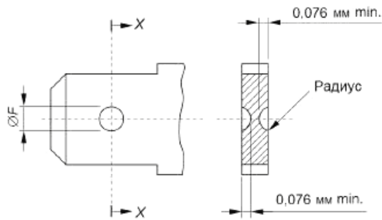
Сечение X-X
