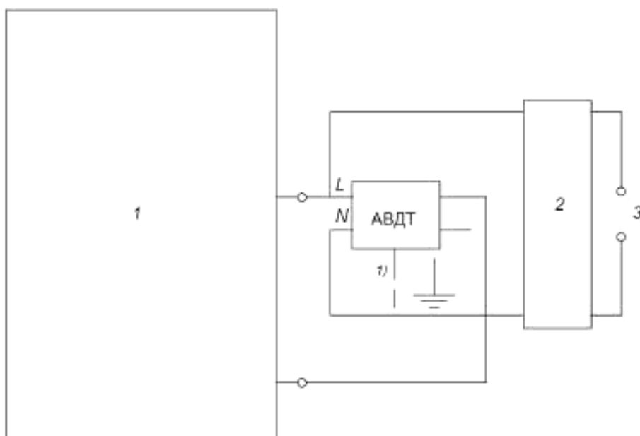
1 – генератор звенящей волны 8/20 мкс; 2 - фильтр; 3 – источник питания
