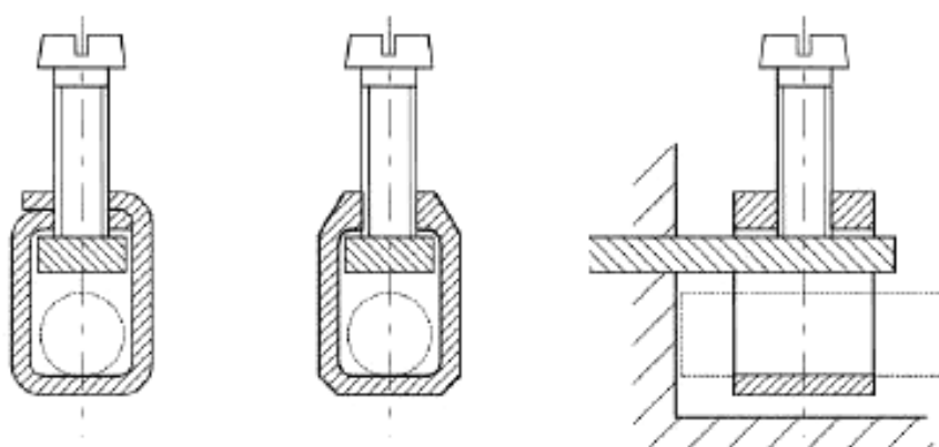
Рисунок IC.1a – Выводы с хомутиком
