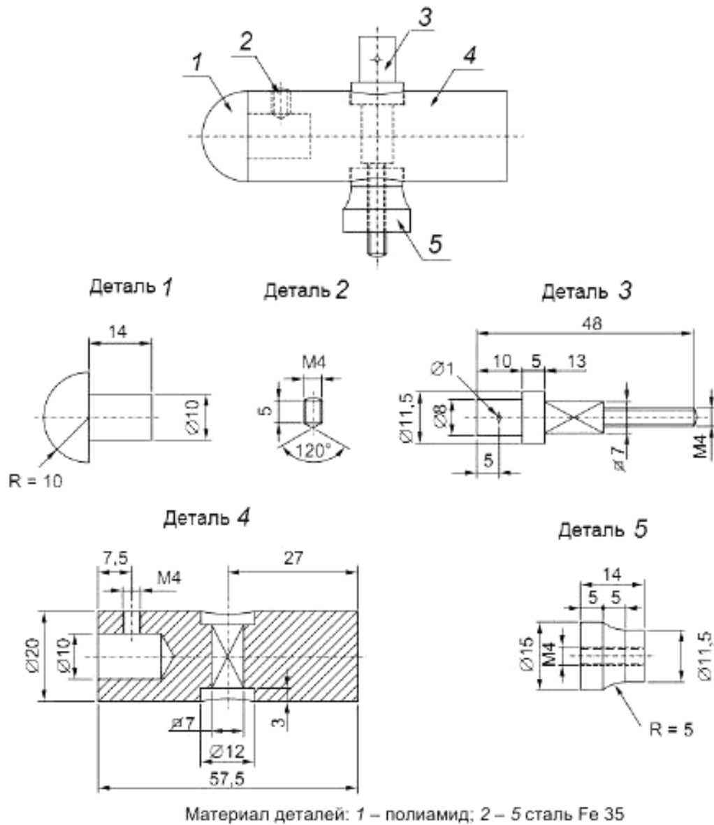
Рисунок 16 – Ударный элемент для маятникового устройства для испытаний на механический удар (см. 9.13.2.1)
