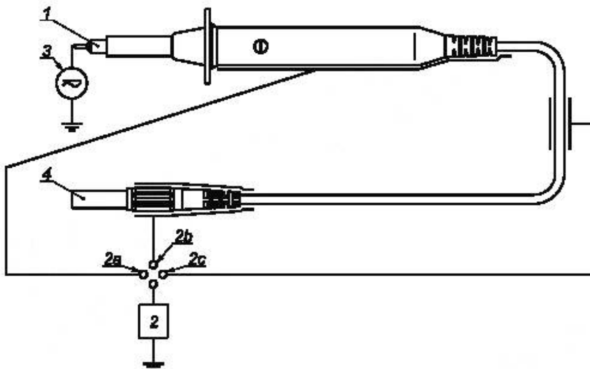
1 — НАКОНЕЧНИК ЩУПА; 2 — цель измерения ДОСТУПНОГО тока (см. приложение А); 2а — соединение с металлической фольгой, покрывающей части, которые управляются рукой или к которым прикасается рука; 2b — соединение с металлической фольгой, покрывающей соединитель; 2с — соединение с металлической фольгой, покрывающей кабель (см. 6.4.3); 3 — максимальное НОМИНАЛЬНОЕ напряжение; 4 — не подключено к оборудованию
