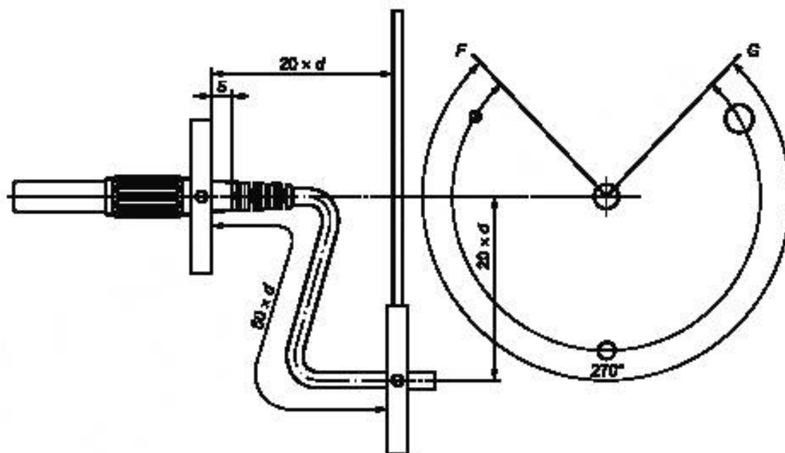
Рисунок 8 — Испытание кабеля ИЗМЕРИТЕЛЬНОГО ЩУПА на изгиб с вращением (см. 6.7.4)
