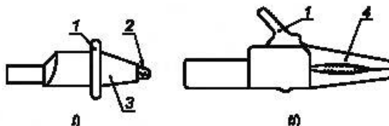
б) Защита посредством расстояния
