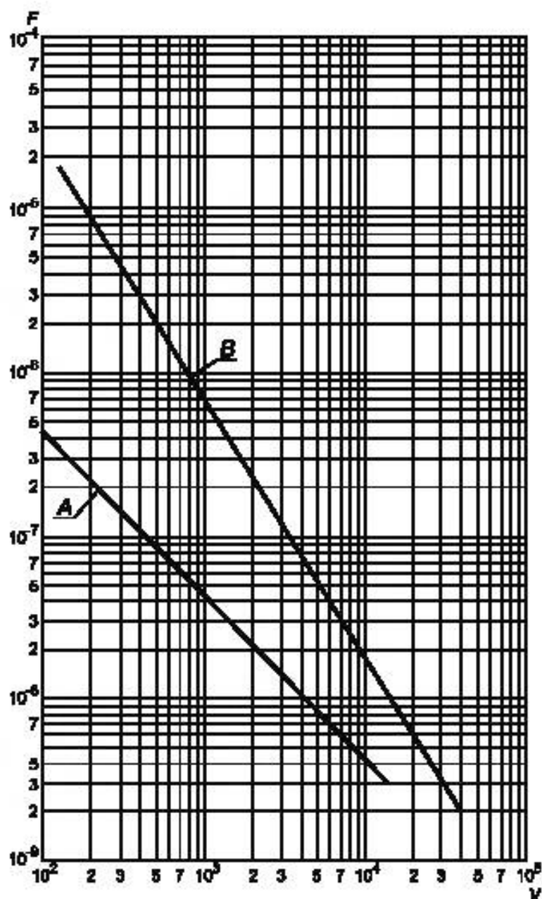
Рисунок 5 — Значения зарядных емкостей в НОРМАЛЬНЫХ УСЛОВИЯХ и при УСЛОВИИ ЕДИНИЧНОЙ НЕИСПРАВНОСТИ (см 6.3.1.3 и 6.3.2.3)
