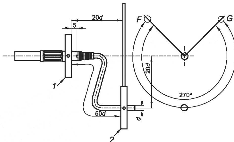
d — диаметр ПРОВОДА ЩУПА; F — начальная точка, конечная точка; G — средняя точка ( F + 270^\circ ); 1 — неподвижный зажим; 2 — вращающийся зажим
