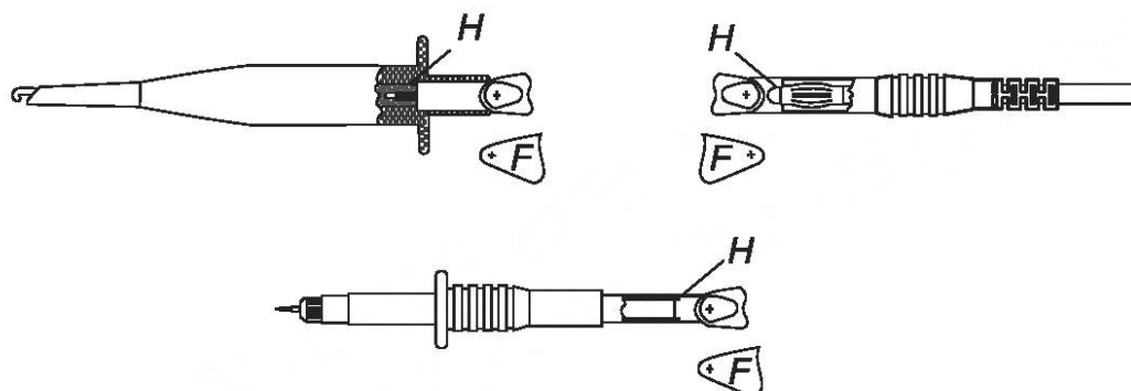
с) Частично сопряженная сборка щупов (см. 7.4.2.3)
