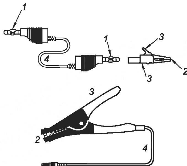
1 — СОЕДИНИТЕЛЬ; 2 — НАКОНЕЧНИК ЩУПА; 3 — область ПРУЖИННОГО ЗАЖИМА, удерживаемая рукой; 4 — ПРОВОД ЩУПА
