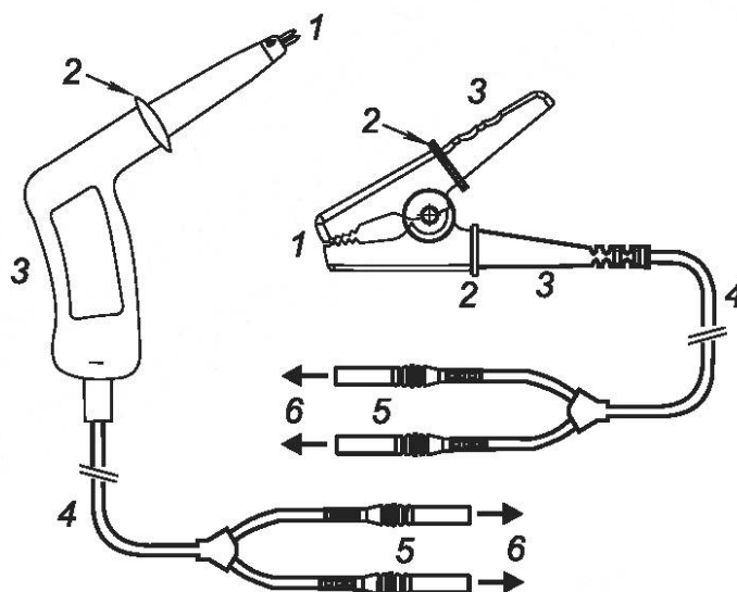
1 — НАКОНЕЧНИК ЩУПА; 2 — ЗАЩИТНЫЙ ПРЕДОХРАНИТЕЛЬ ПАЛЬЦЕВ; 3 — область корпуса сборки щупа, удерживаемая рукой; 4 — ПРОВОД ЩУПА; 5 — СОЕДИНИТЕЛЬ; 6 — подключение к оборудованию
