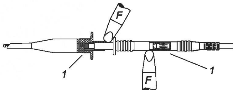
а) Части сборки щупов
