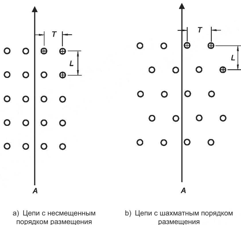
Рисунок D.1 — Конфигурация бисерной цепи (если применимо)
