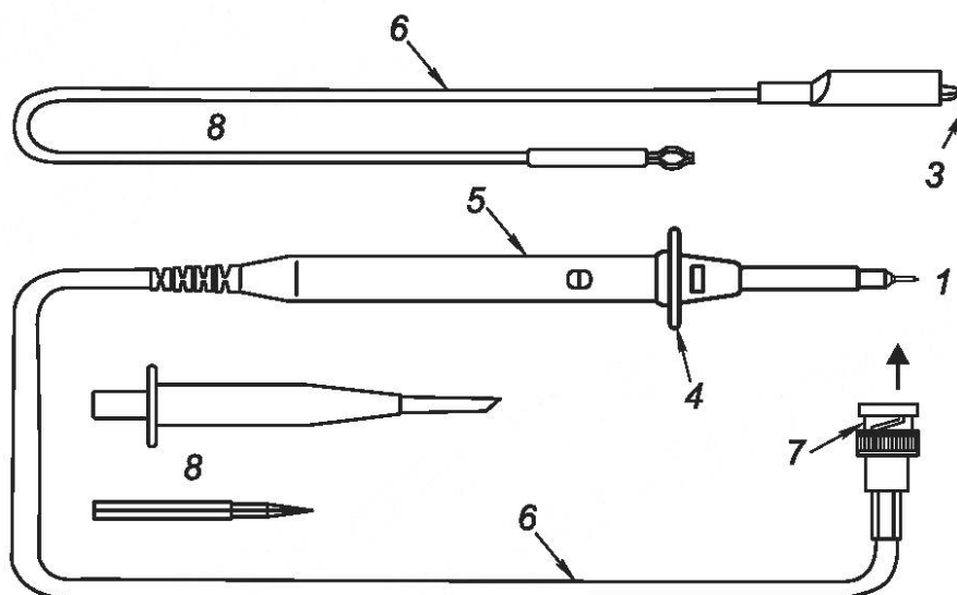
а) Сборка щупов типа В для высоковольтной сети
