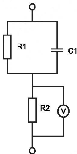
Рисунок А.3 — Схема измерения тока, вызывающего электрический ожог
