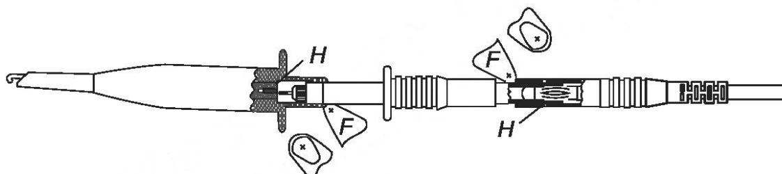
б) Полностью сопряженная сборка щупов (см. 7.4.2.2)
