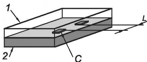
1 — первый слой; 2 — второй слой; C — проводник; L — расстояние между проводниками
