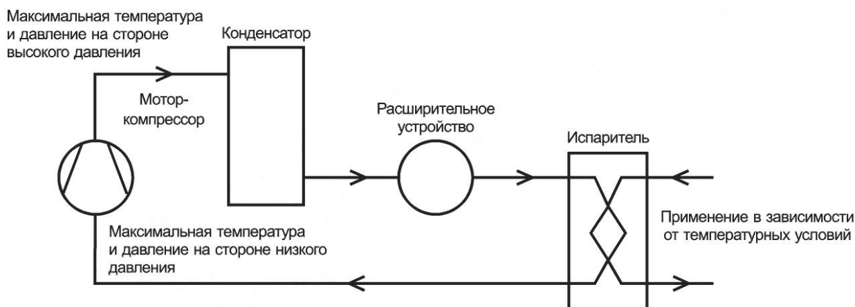
Рисунок 101 — Схема системы охлаждения со встроенным конденсатором
