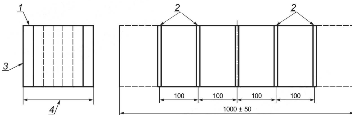
1 — меньшая ось кабеля; 2 — проволочный бандаж; 3 — большая ось кабеля; 4 — n -е количество испытуемых отрезков Рисунок 3 — Способ формирования плоского горизонтального блока из некруглых кабелей
