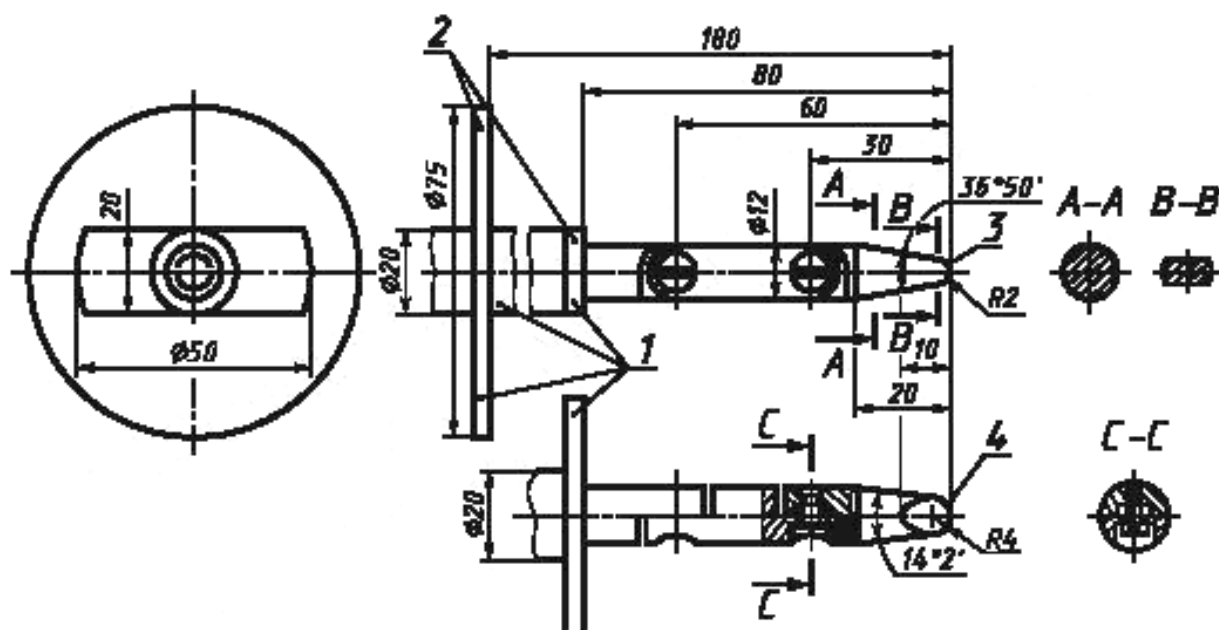
1 — изоляционный материал; 2 — стопорная плата; 3 — цилиндр; 4 — сфера
