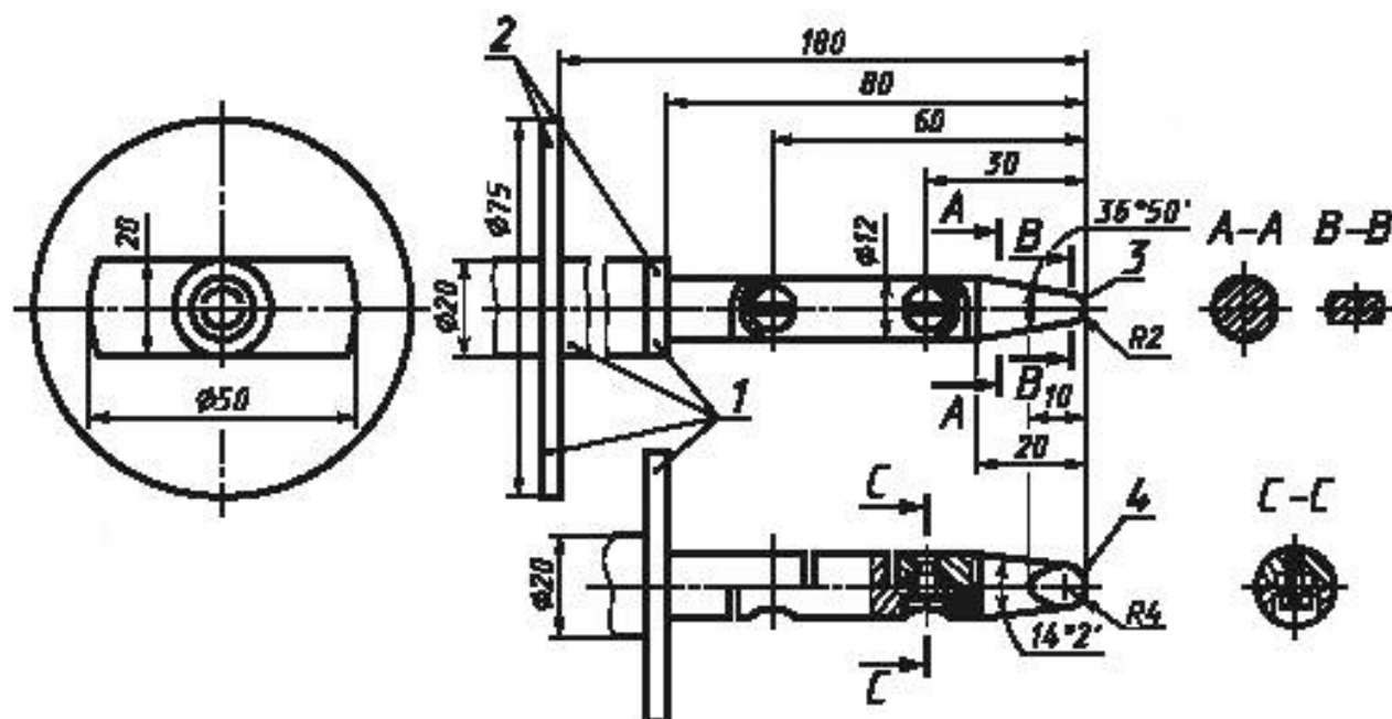
1 — изоляционный материал; 2 — опорная плата; 3 — цилиндр; 4 — сфера
