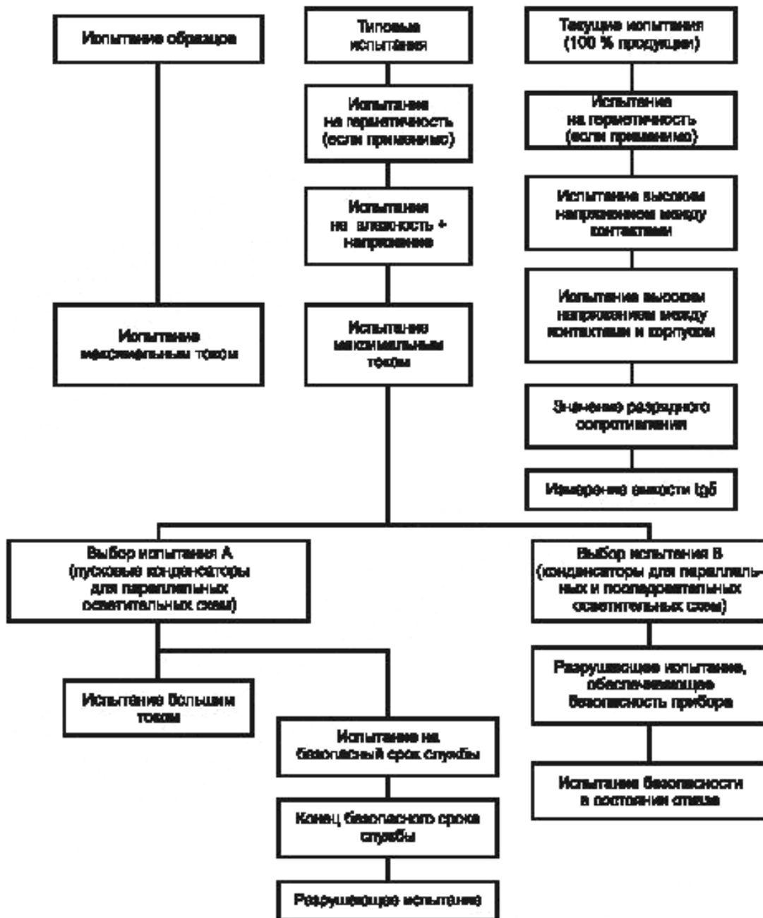
Рисунок 4 — Схема процедуры испытаний
