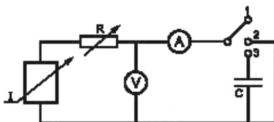
Рисунок 2 — Схема выдержки на постоянном напряжении
