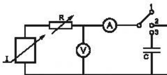
Рисунок 2 — Схема выдержки на постоянном напряжении
