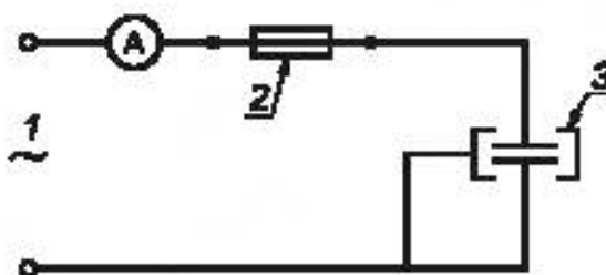
1 — источник переменного напряжения; 2 — плавкий предохранитель; 3 — конденсатор
