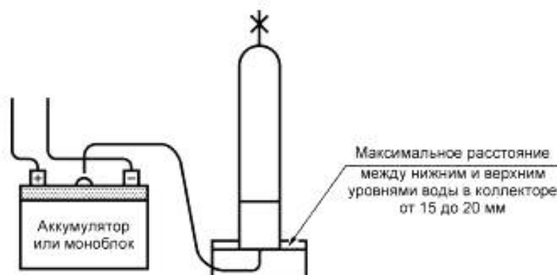
Рисунок 1 — Пример приспособления для сбора газа
