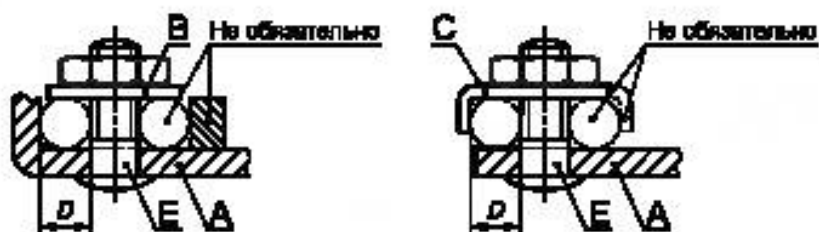
Рисунок 2б — Шпильчные зажимы
