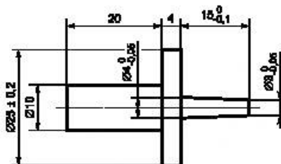
Рисунок 13 — Испытательный стержень
