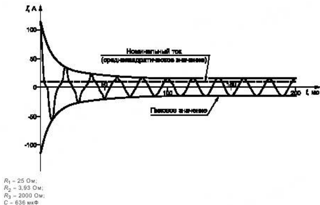
Рисунок 10 — Характеристики испытательной цепи с емкостной нагрузкой для испытания выключателей с номинальными параметрами 10/100 А 250 В —
