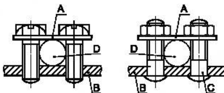
Рисунок 2 — Примеры винтовых и шпильчных зажимов
