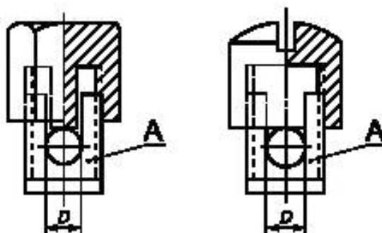
Рисунок 4 — Примеры зажимов под наконечник
