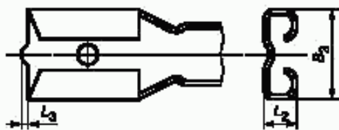
Рисунок 7 — Вставки плоских втычных соединителей
