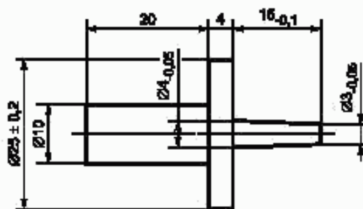
Рисунок 13 — Испытательный стержень
