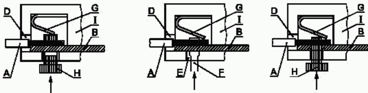
б) Безвинтовой зажим-вывод с зажимающими средствами прямого действия, ослабляемыми с помощью инструмента.
