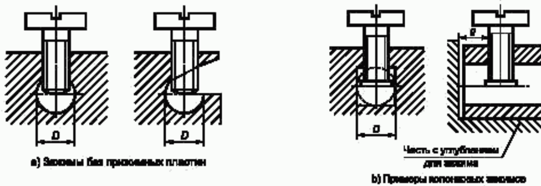
Рисунок 1 — Примеры колонковых зажимов
