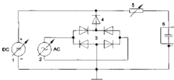
Рисунок 2 — Источник постоянного тока N — Тип 1
