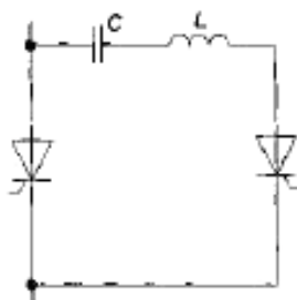
Рисунок А.1б — Пример контура коммутации
