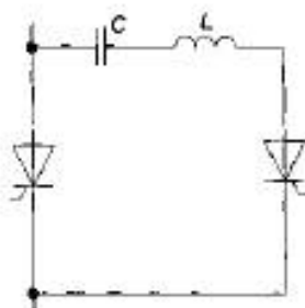
Рисунок А.1b — Пример контура коммутации
