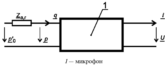
Рисунок 1 — Эквивалентная схема микрофона-приемника в свободном поле
