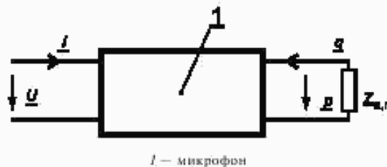
Рисунок 2 — Эквивалентная схема микрофона-излучателя в свободном звуковом поле
