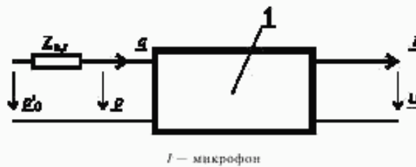
Рисунок 1 — Эквивалентная схема микрофона-приемника в свободном поле
