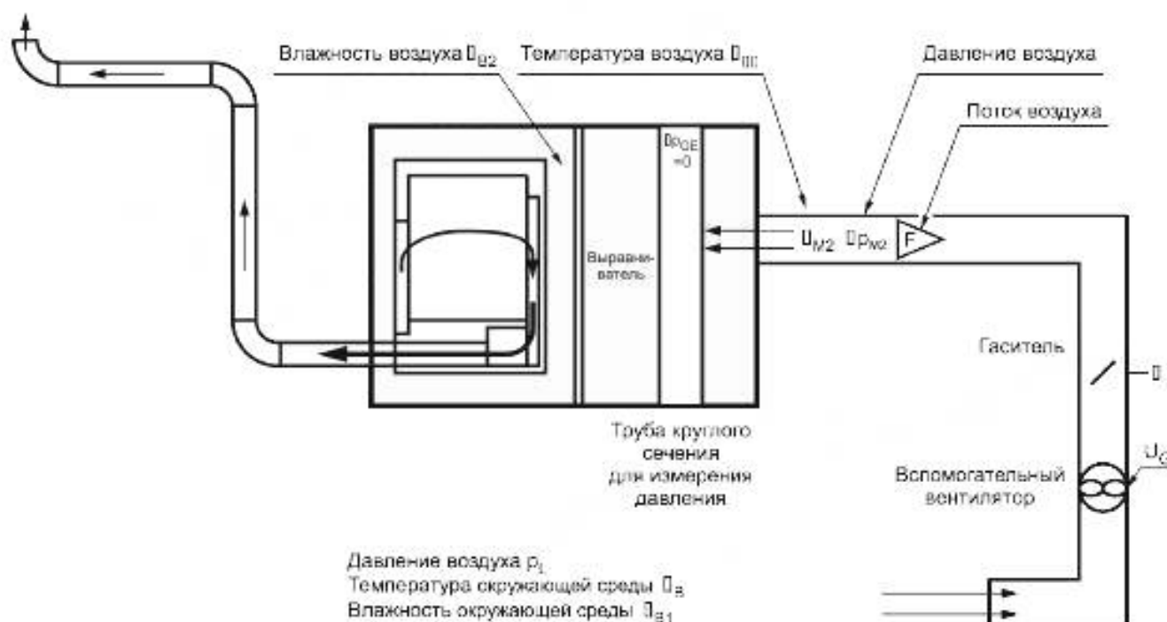
Рисунок Н.1 — Компоновка приемной камеры
