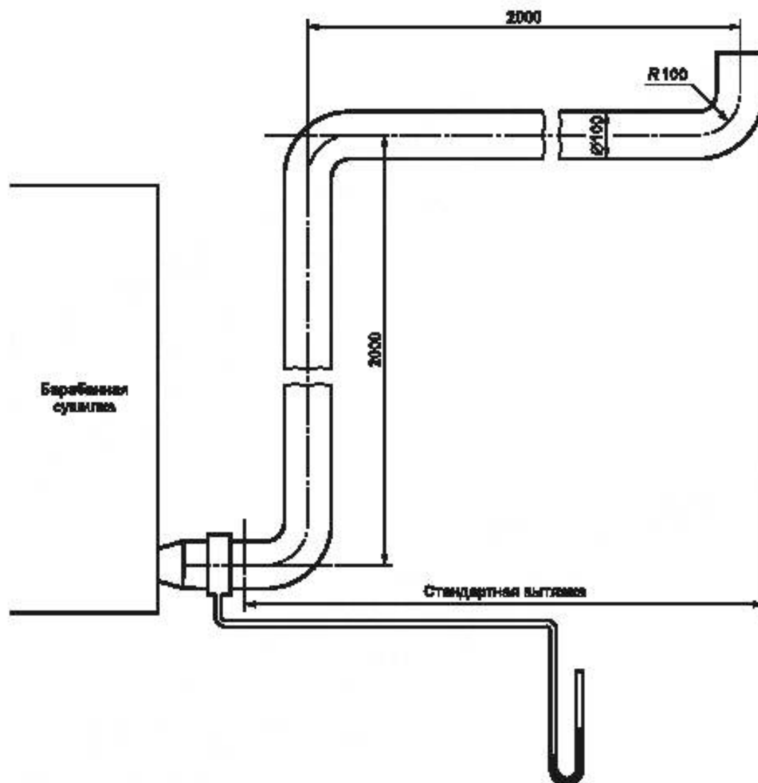
Рисунок В.2 — Стандартный вытяжной воздуховод
