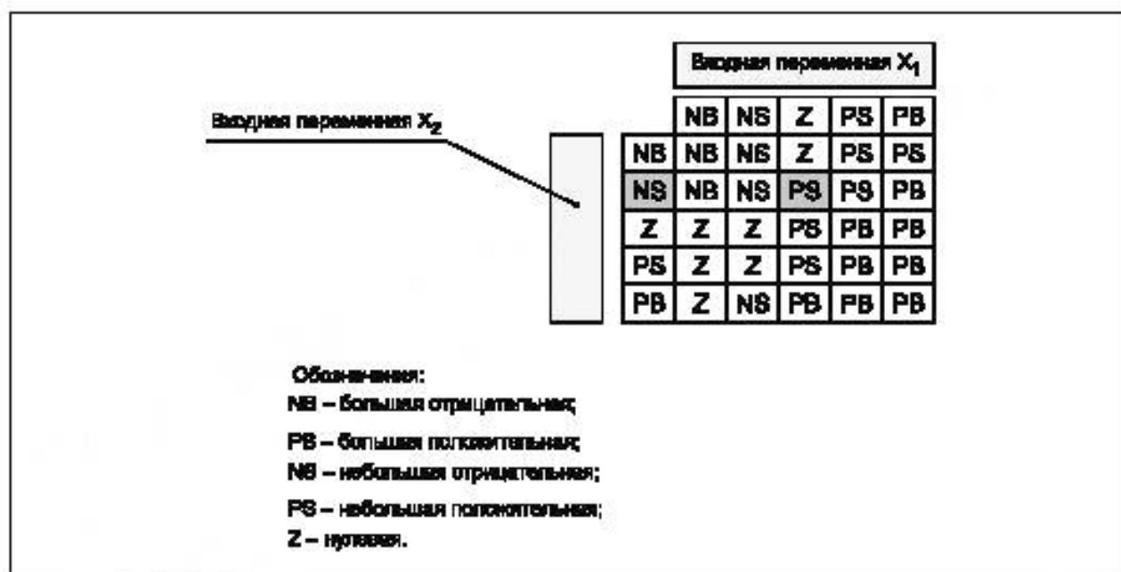
Рисунок A.8 — Матричное представление двух переменных
