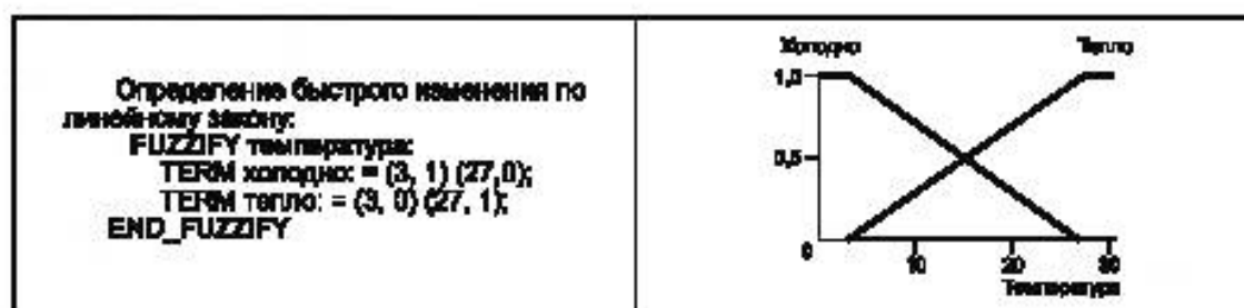
Рисунок 4 — Пример термов быстрого изменения по линейному закону
