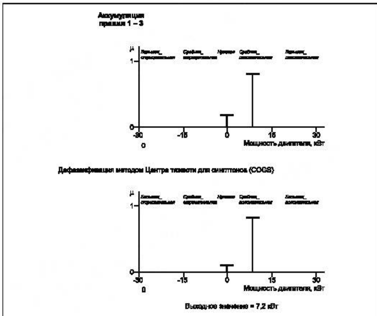
Рисунок С.15 — Дефазификация
