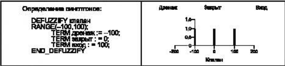
Рисунок 6 — Примеры термов синглтонов
