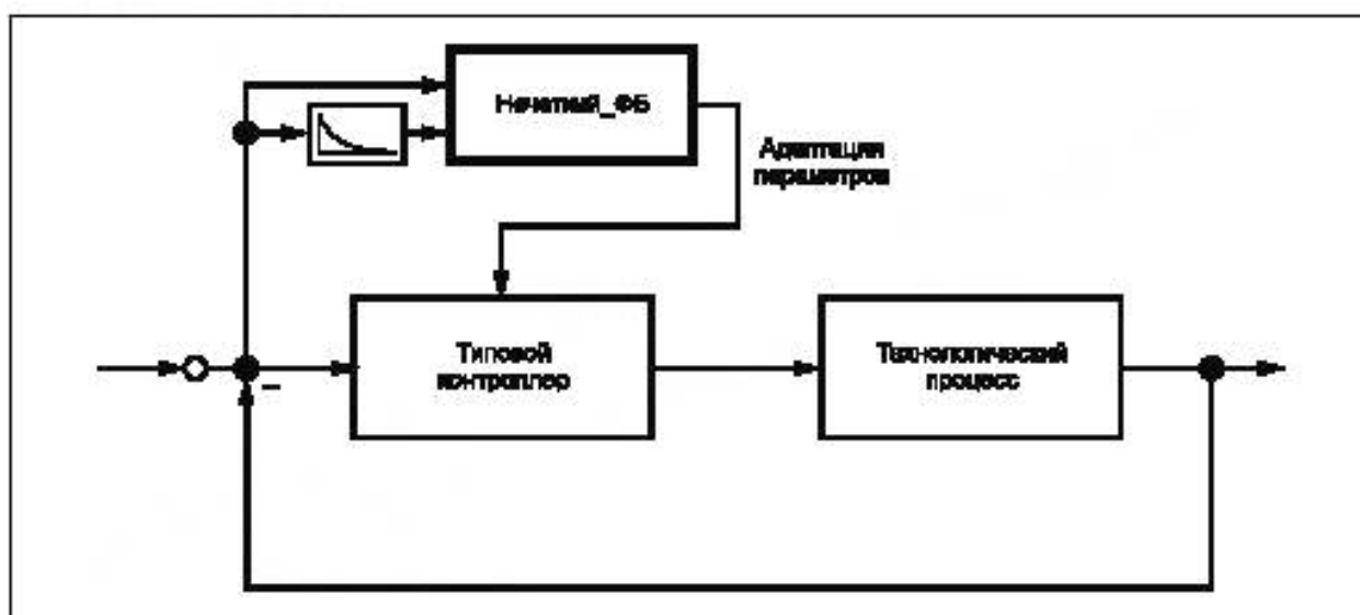
Рисунок В.2 — Пример адаптации параметров
