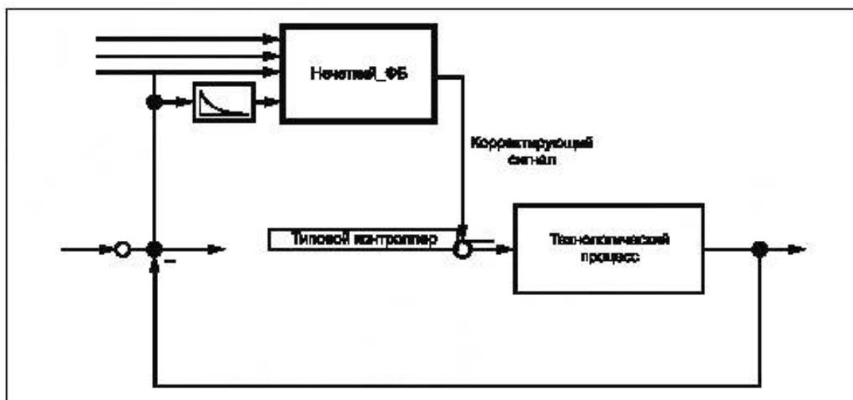
Рисунок В.1 — Пример предварительного регулирования
