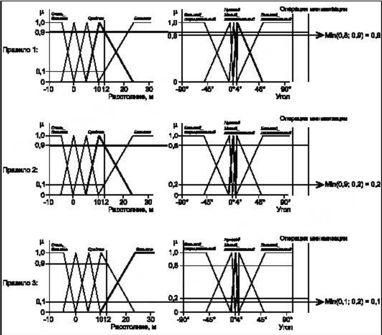
Рисунок С.10 — Принципы агрегирования
