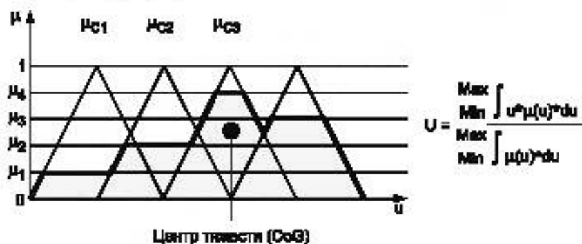
Рисунок А.11а — Методы дефазификации
