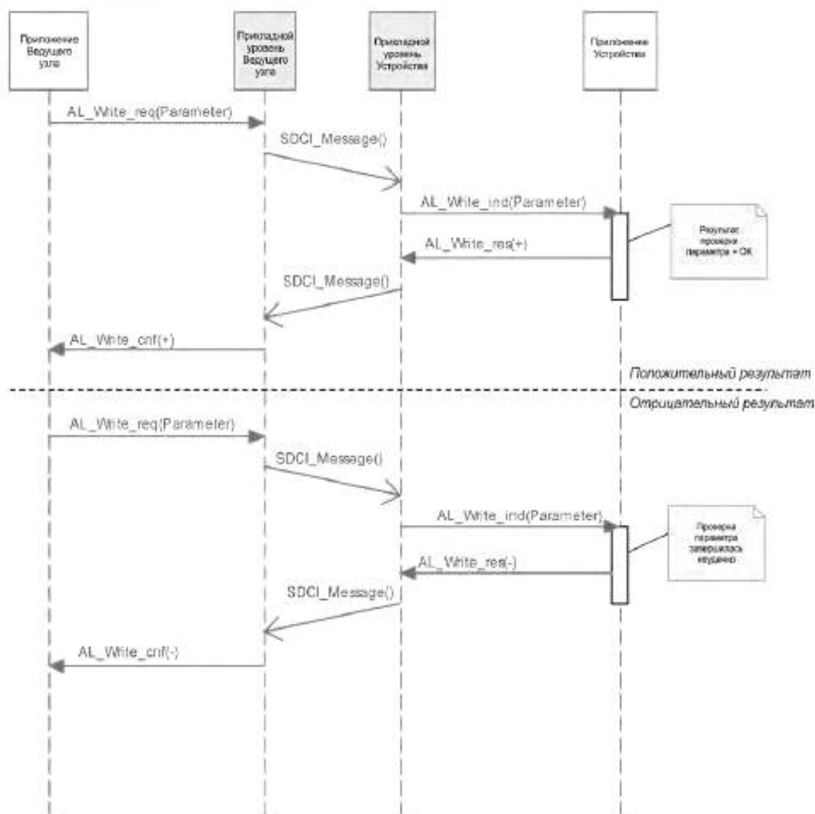
Рисунок 85 — Положительный и отрицательный результаты проверки параметра
