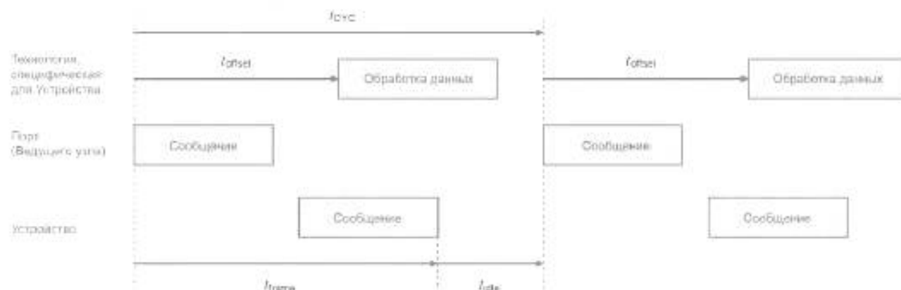
Рисунок 90 — Временная диаграмма цикла
