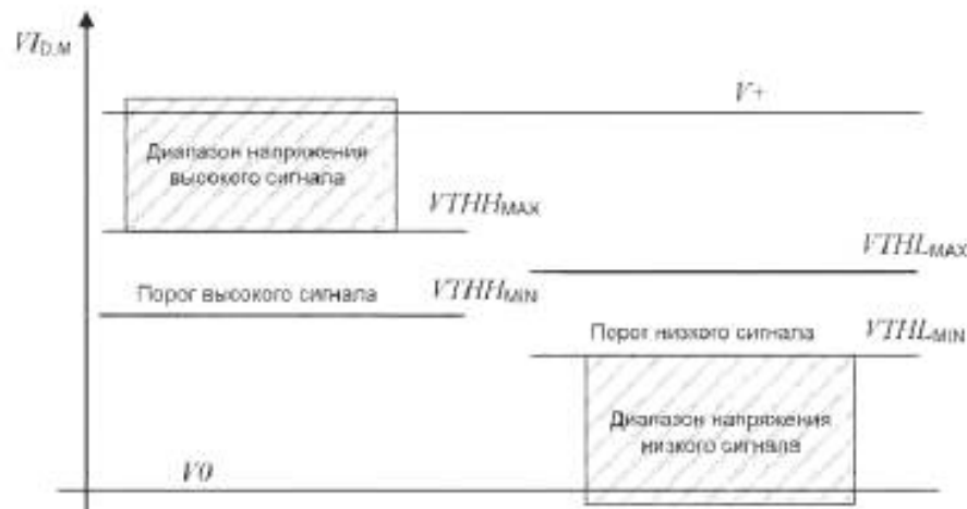
Рисунок 17 — Пороги переключения
