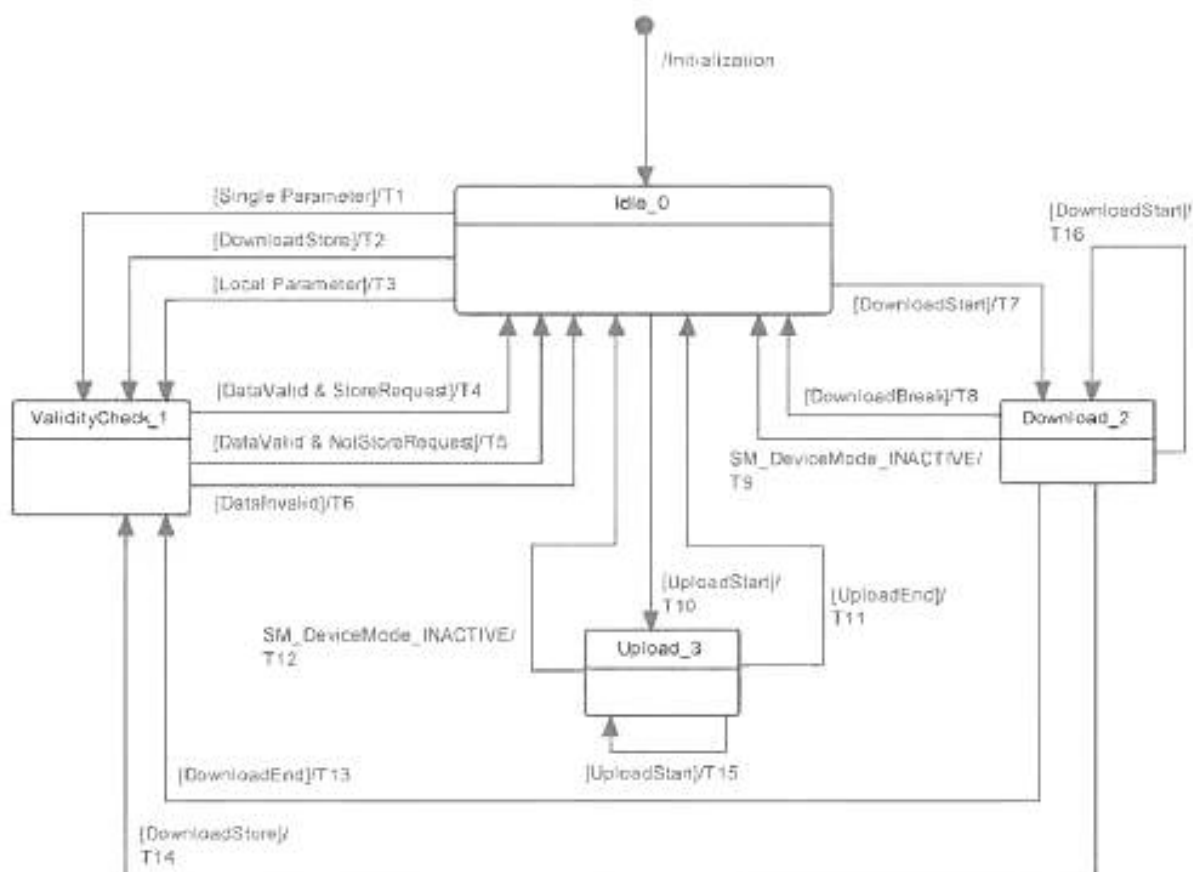
Рисунок 84 — Конечная машина PM
