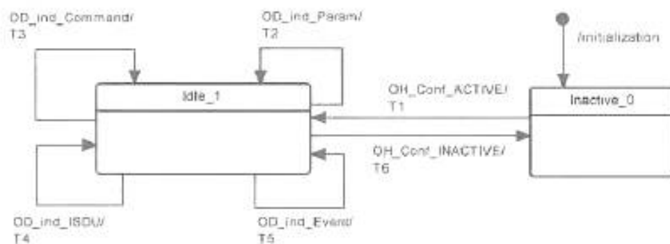
Рисунок 47 — Конечная машина обработчика OD на Устройстве
