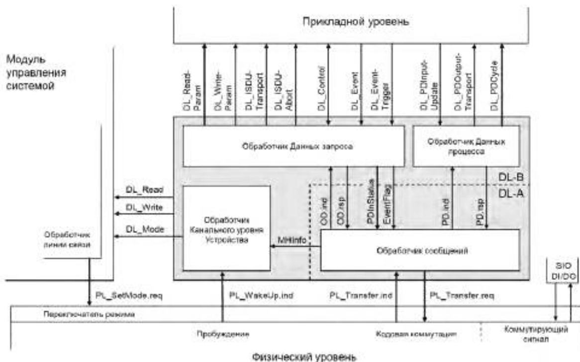
Рисунок 27 — Структура и услуги DL (Устройства)
