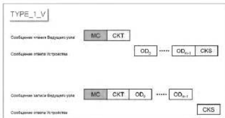
Рисунок A.8 — M-последовательность типа TYPE_1_V
