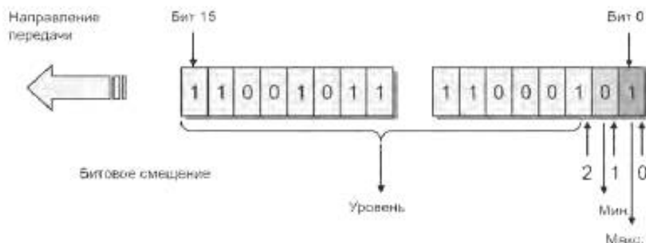
Рисунок Е.7 — Пример 2 структуры типа данных RecordT
