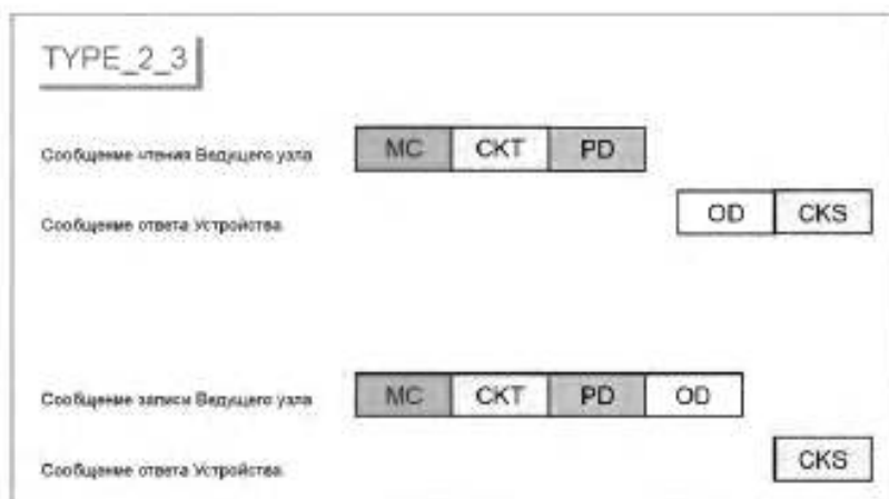
Рисунок А.11 — М-последовательность типа TYPE_2_3
