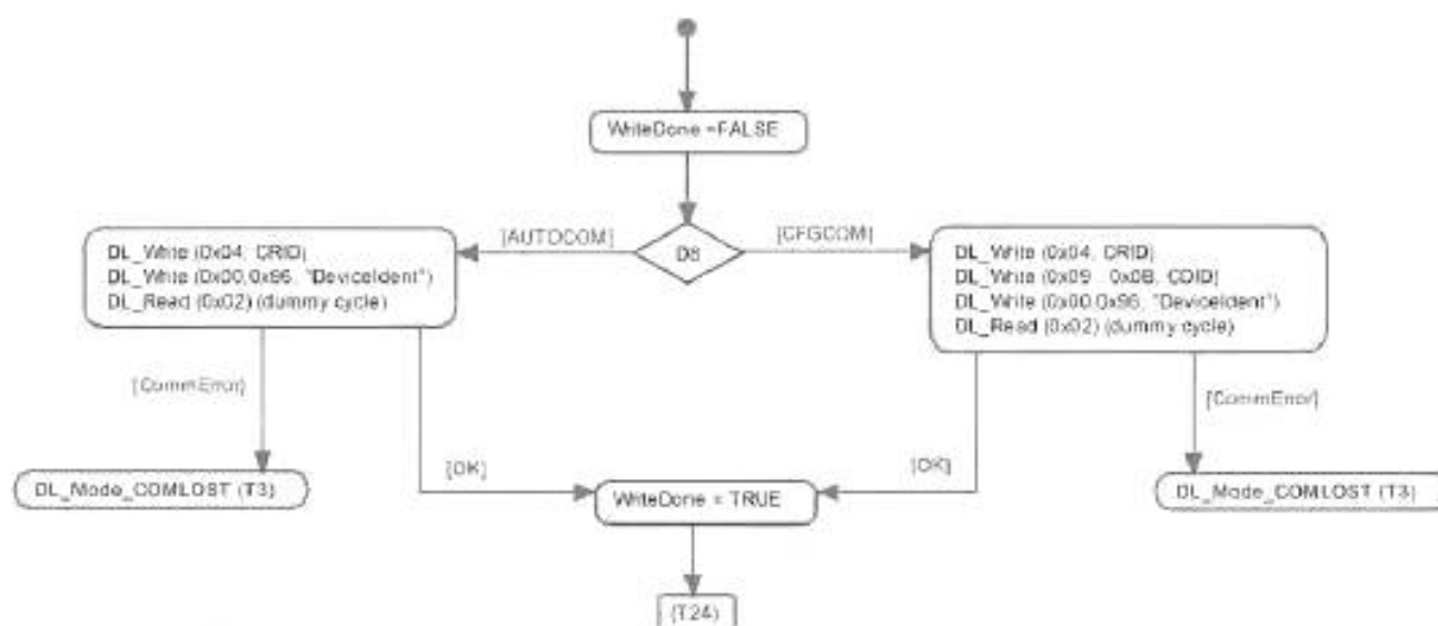
Рисунок 74 — Действия (запись параметра) в состоянии RestartDevice
