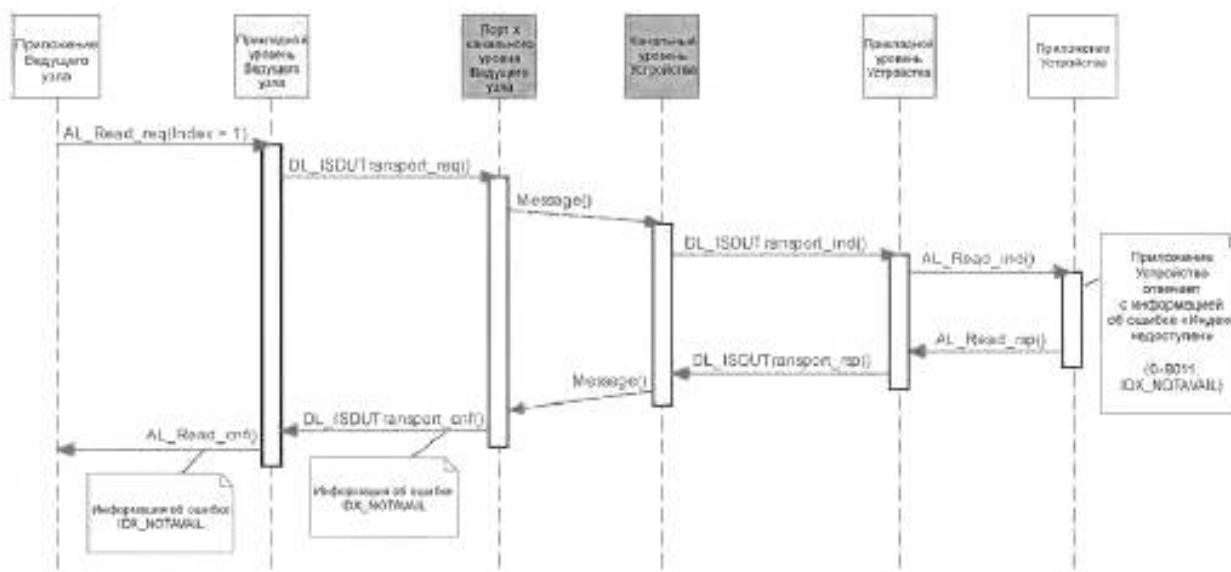
Рисунок 60 — Диаграмма последовательностей для OD в случае ошибок
