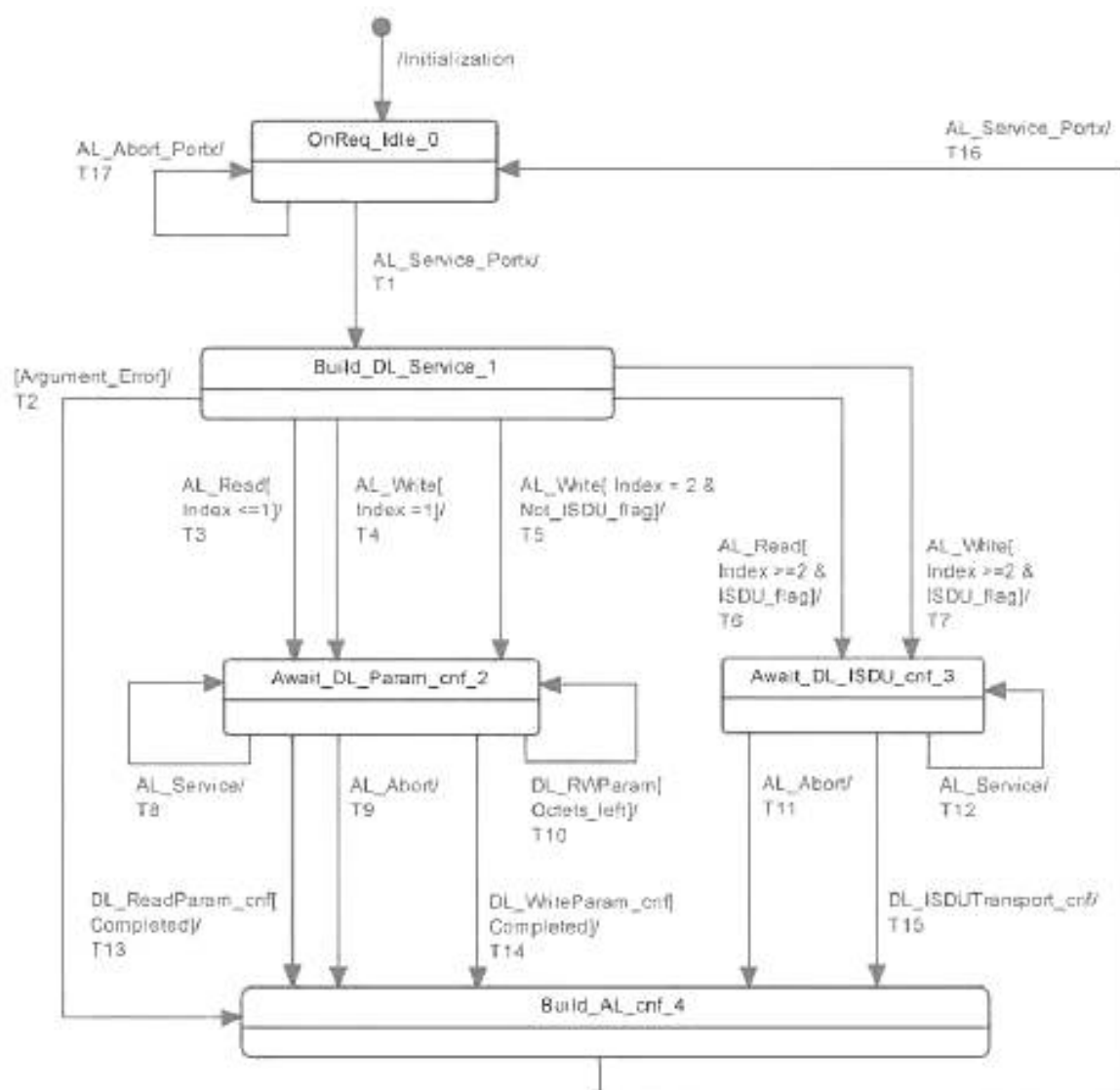
Рисунок 57 — Конечная машина OD AL Ведущего узла
