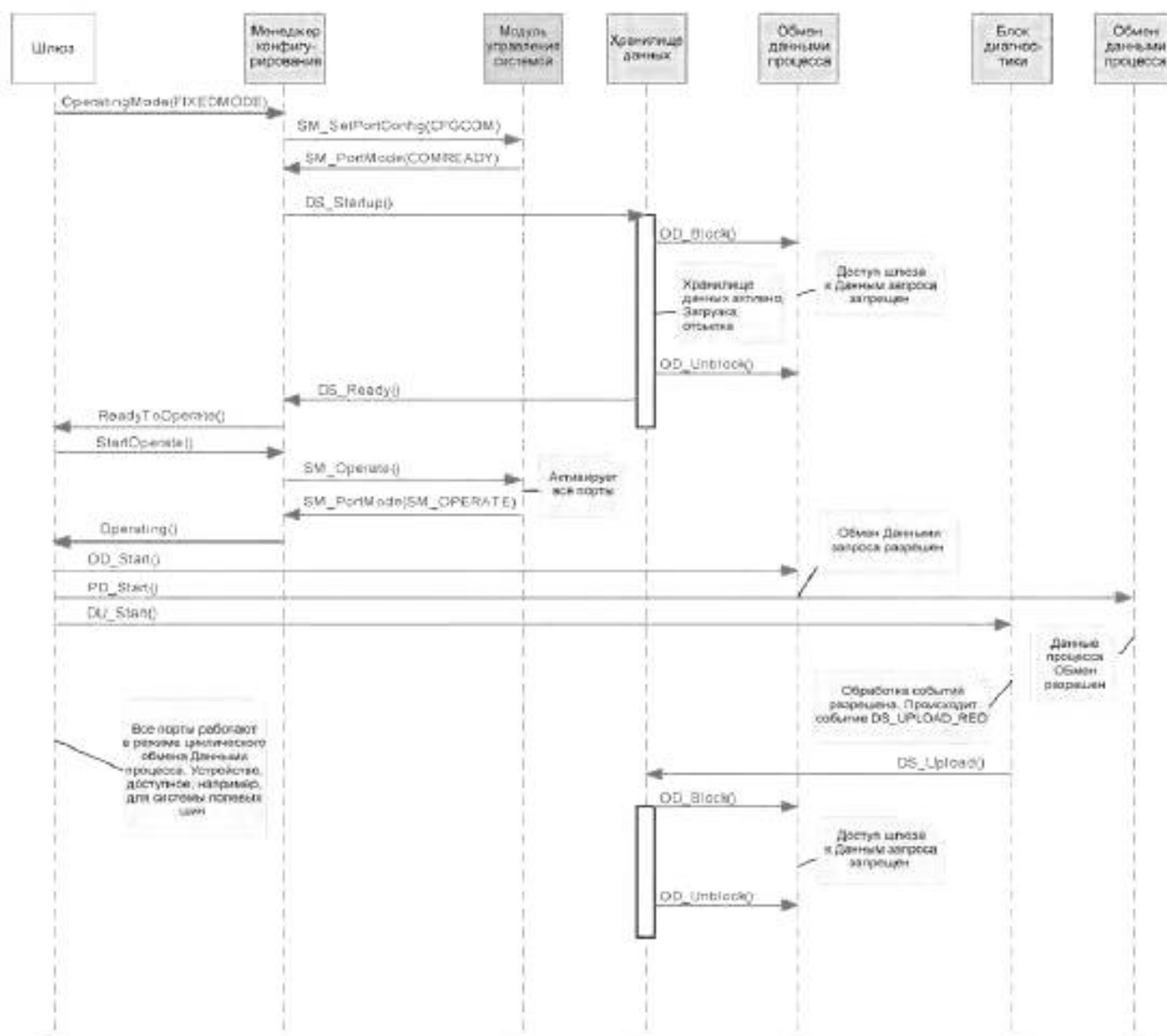
Рисунок 96 — Диаграмма последовательности действий CM
