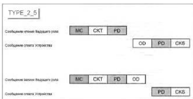
Рисунок А.13 — М-последовательность типа TYPE_2_5
