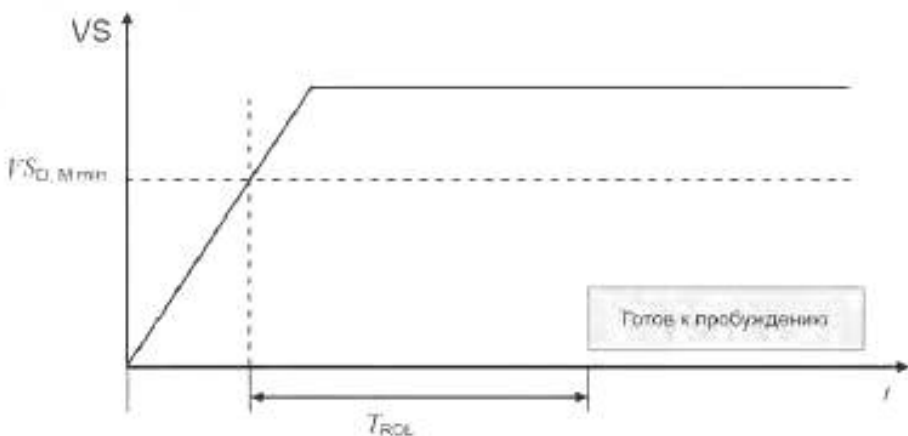
Рисунок 22 — Регламент подачи питания для источника Питания 1
