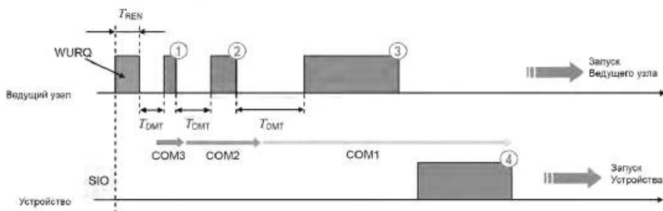
Рисунок 29 — Пример попытки установления связи
