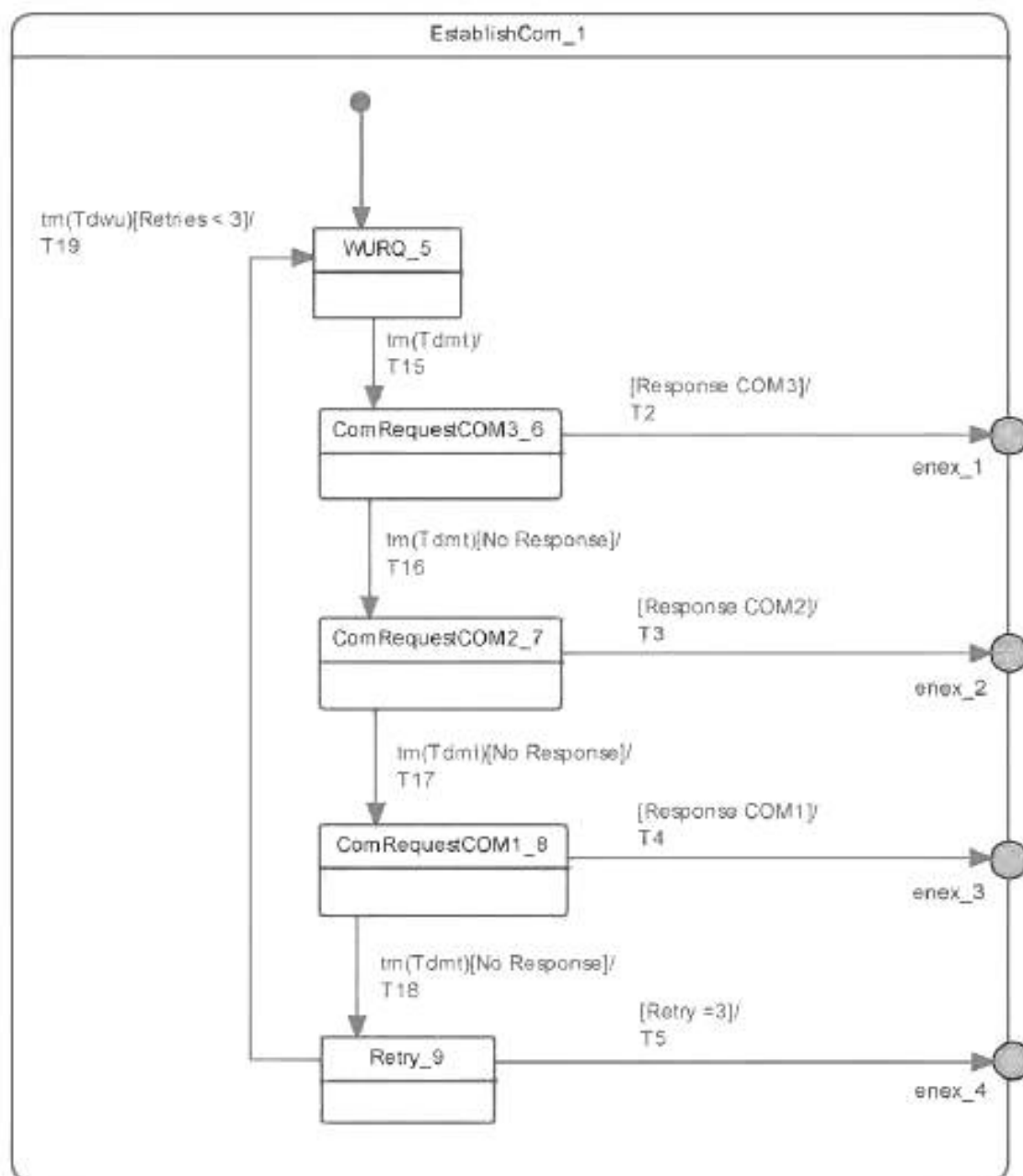
Рисунок 34 — Функциональный узел 1 для установки связи
