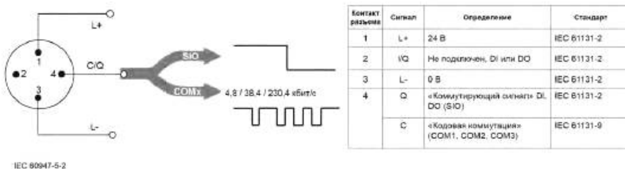
Рисунок 3 — Совместимость SDCI с МЭК 61131-2
