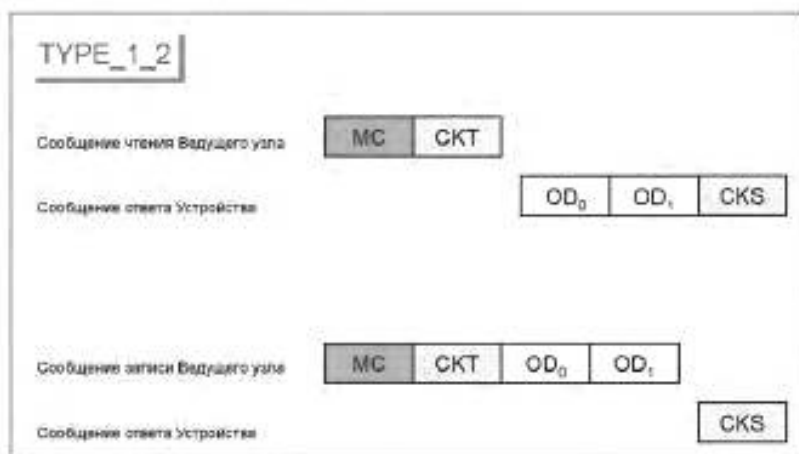
Рисунок А.7 — М-последовательность типа TYPE_1_2
