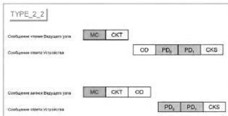
Рисунок A.10 — M-последовательность типа TYPE_2_2
