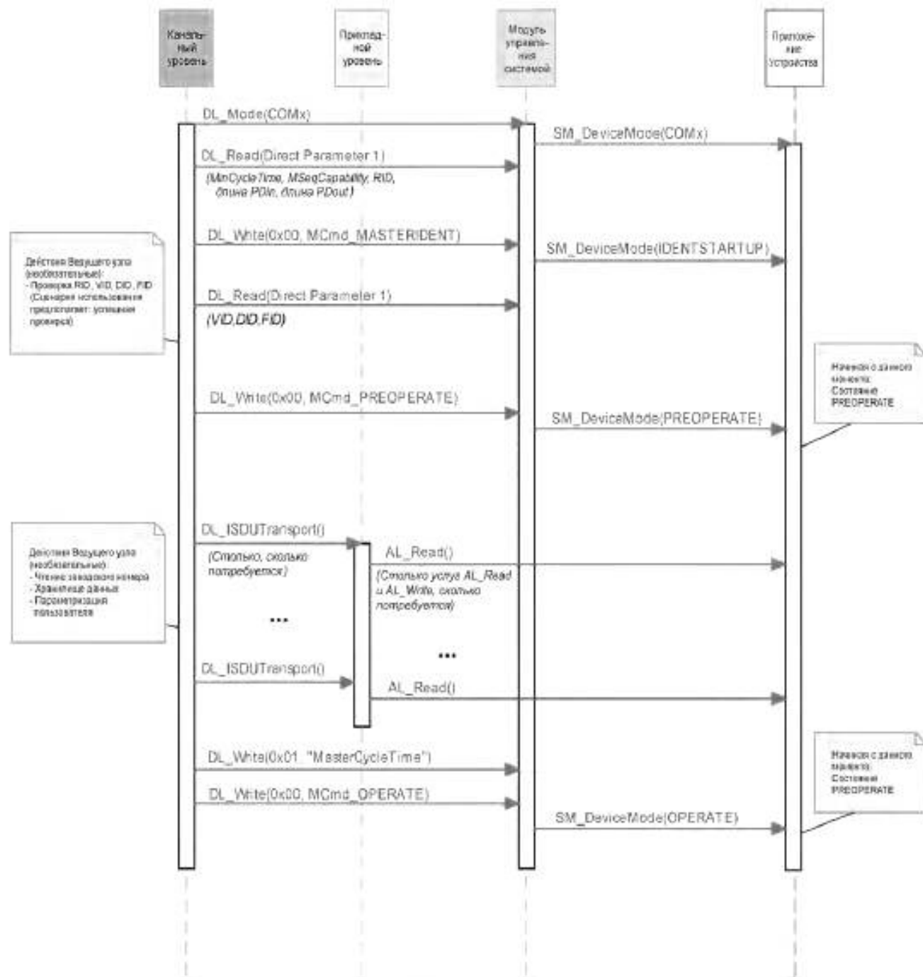
Рисунок 80 — Диаграмма последовательностей нормального запуска Устройства
