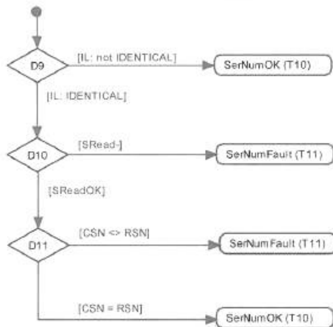
Рисунок 76 — Действия (проверка заводского номера) для состояния CheckSerNum_3
