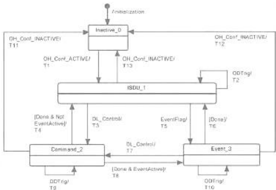
Рисунок 46 — Конечная машина обработчика OD Ведущего узла
