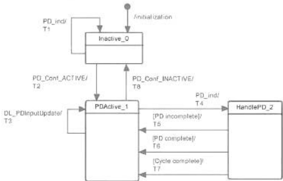
Рисунок 45 — Конечная машина обработчика PD Устройства
