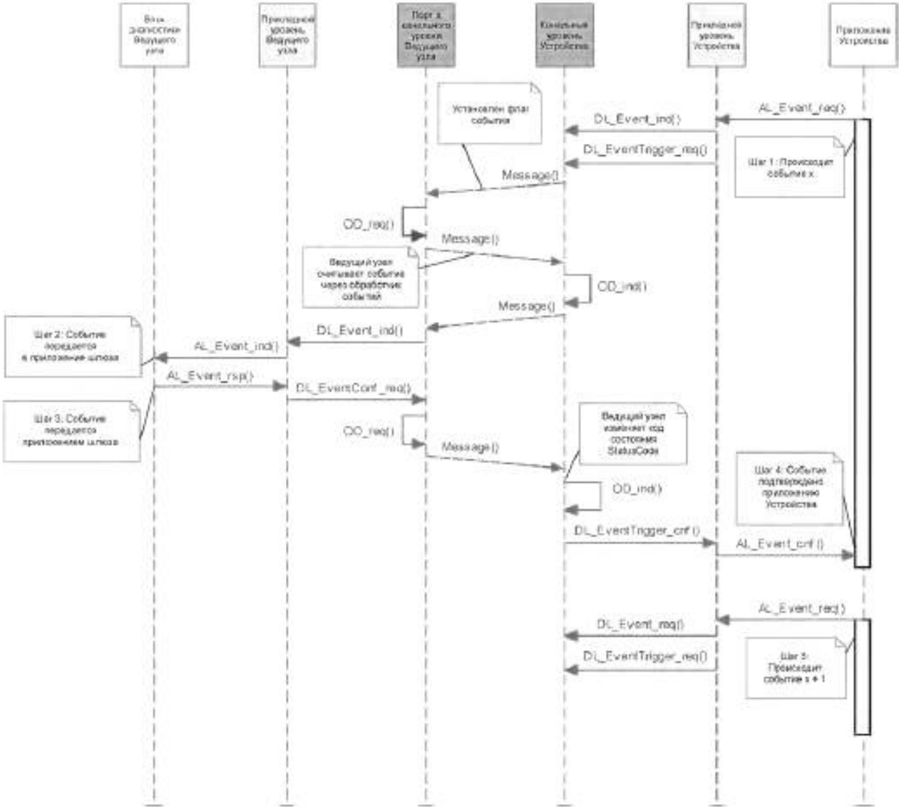
Рисунок 64 — График одиночного События
