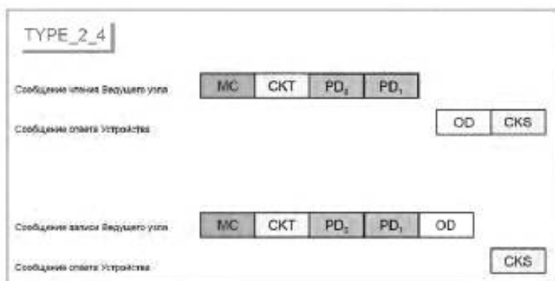
Рисунок А.12 — М-последовательность типа TYPE_2_4
