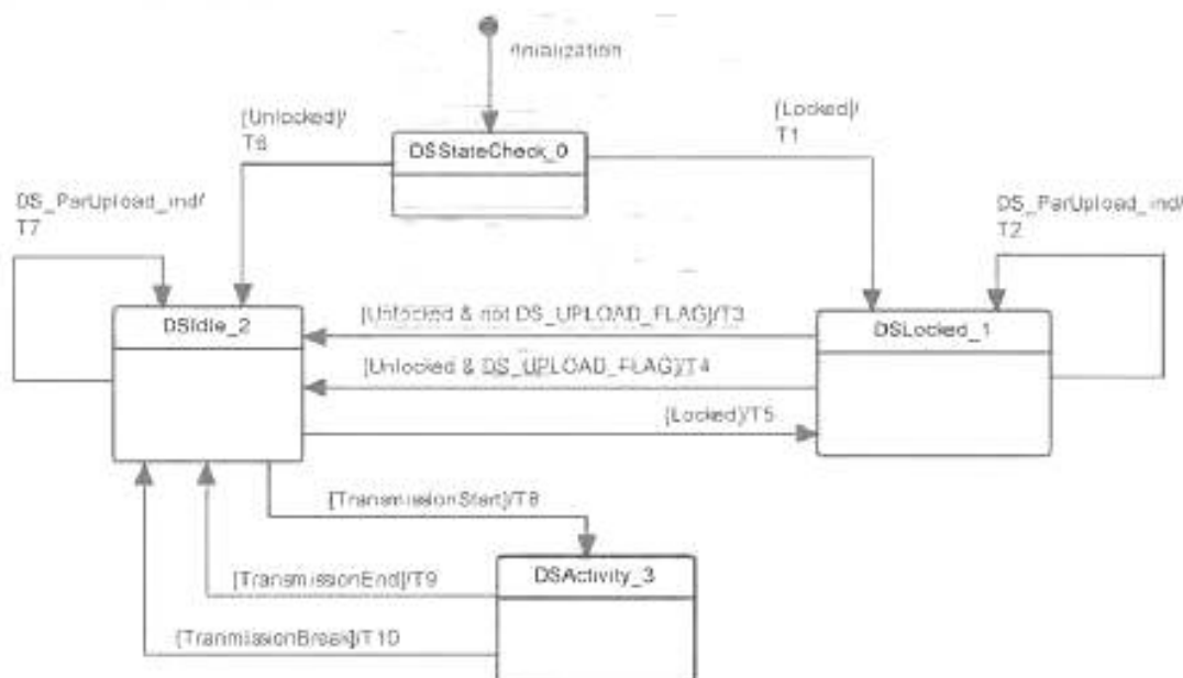
Рисунок 88 — Конечная машина DS
