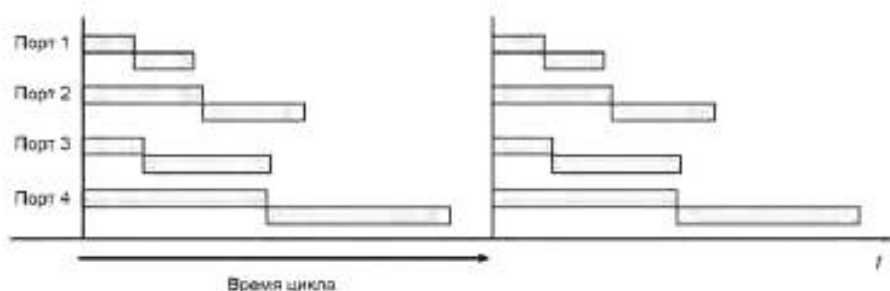
Рисунок 97 — Порты в режиме синхронизации сообщений MessageSync
