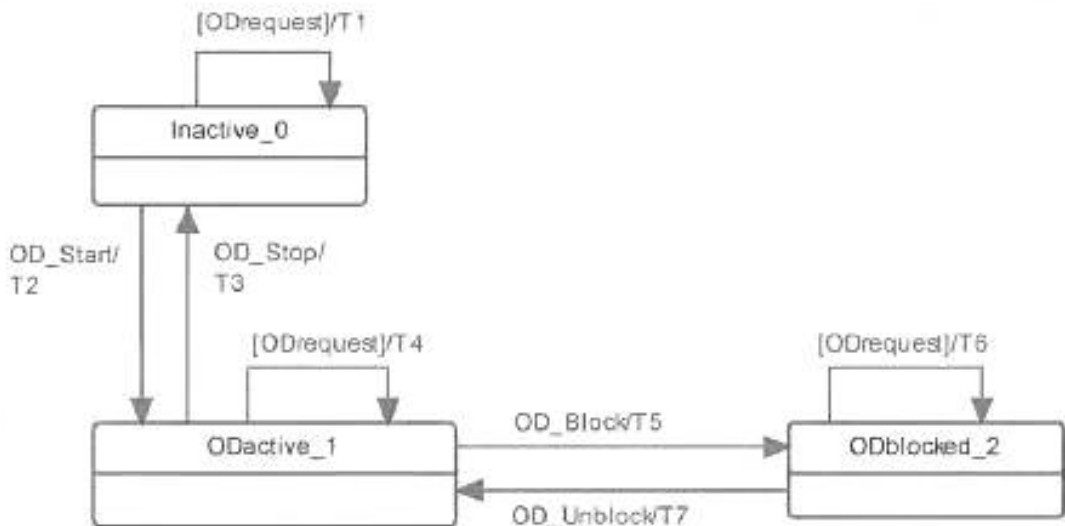
Рисунок 105 — Конечная машина Обмена OD
