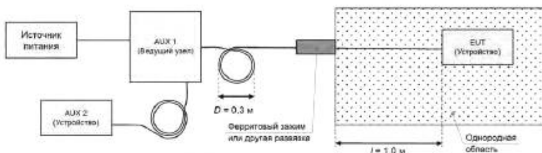
Рисунок G.6 — Установка для испытаний на устойчивость к радиочастотному электромагнитному полю (Устройство)
