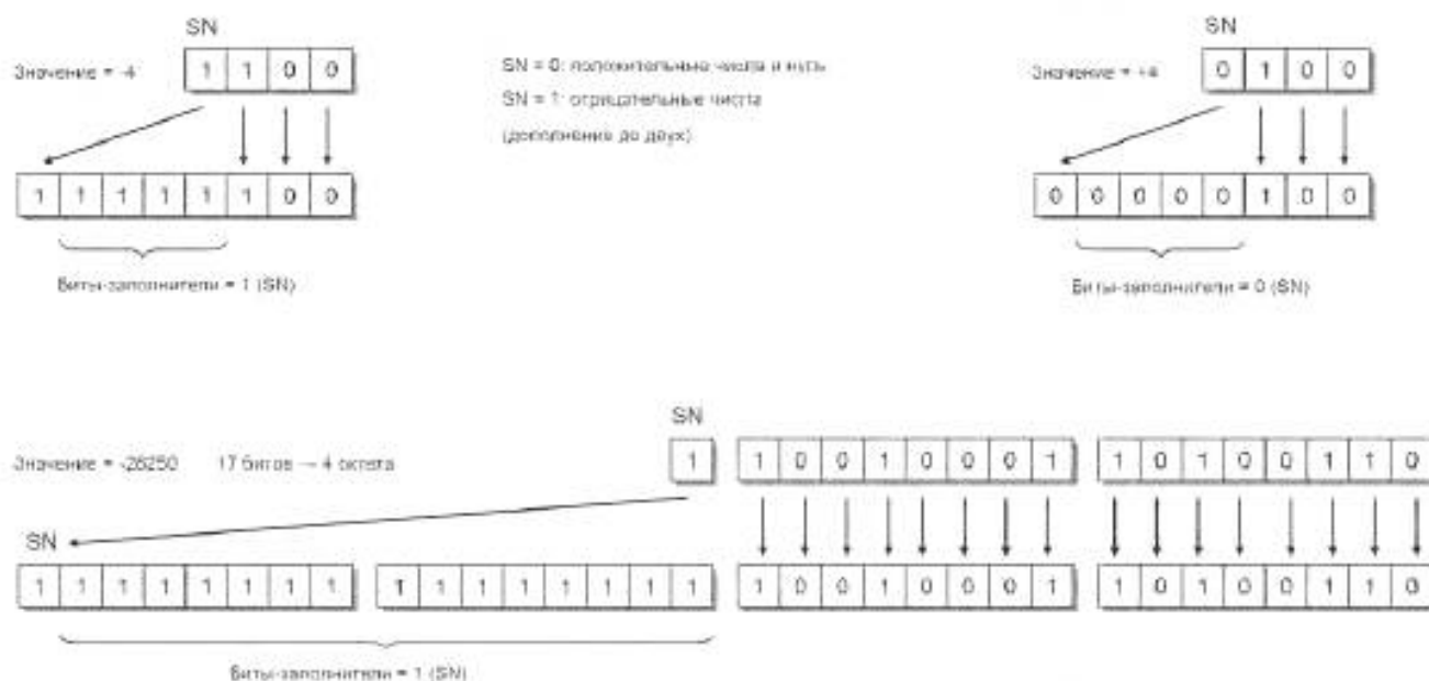
Рисунок E.2 — Примеры кодирования типа данных IntegerT
