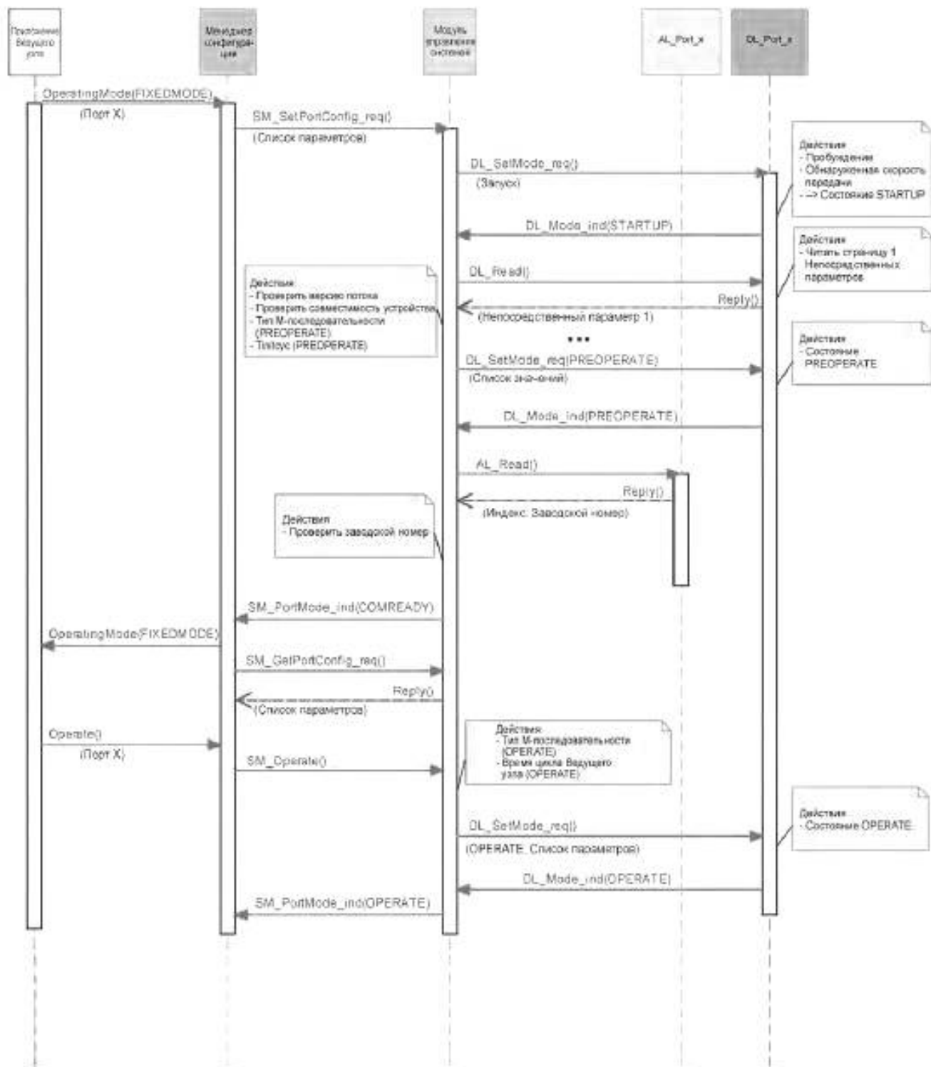
Рисунок 68 — Схема последовательности сценария использования «Настройка порта»
