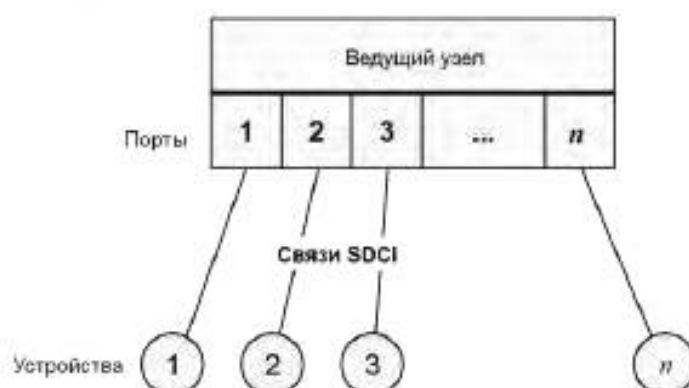
Рисунок 10 — Топология SDCI
