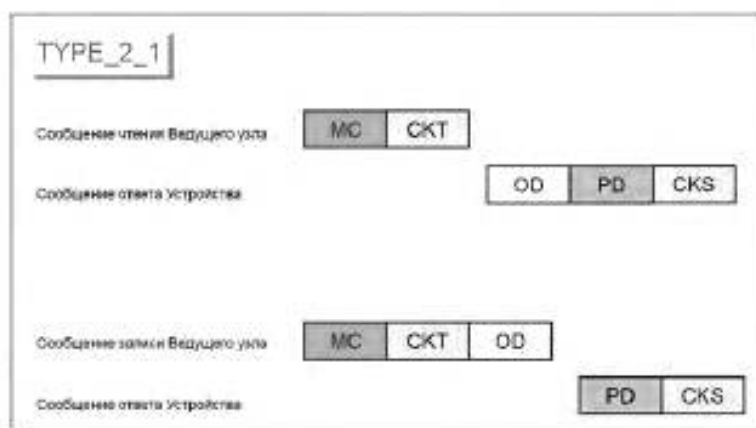
Рисунок A.9 — M-последовательность типа TYPE_2_1
