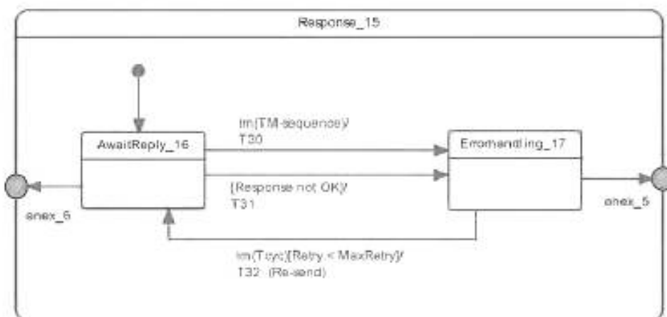
Рисунок 41 — Функциональный блок «Response 15» обработчика прерываний
