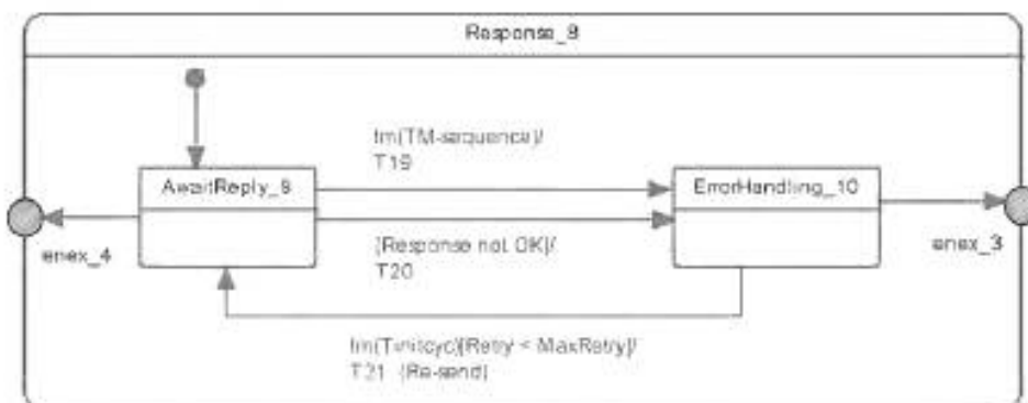
Рисунок 40 — Функциональный блок «Response 8» обработчика прерываний
