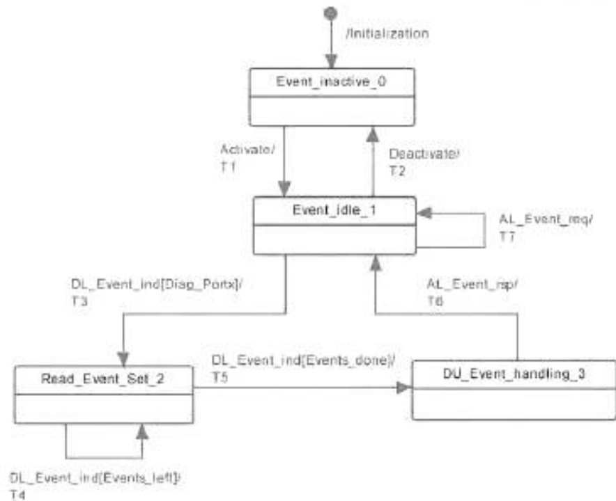
Рисунок 62 — Конечная машина Событий AL на Ведущем узле
