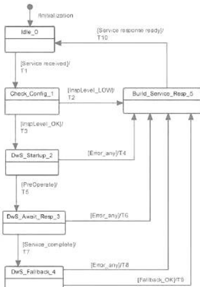
Рисунок 112 — Режим DIwithSDCI виртуального порта
