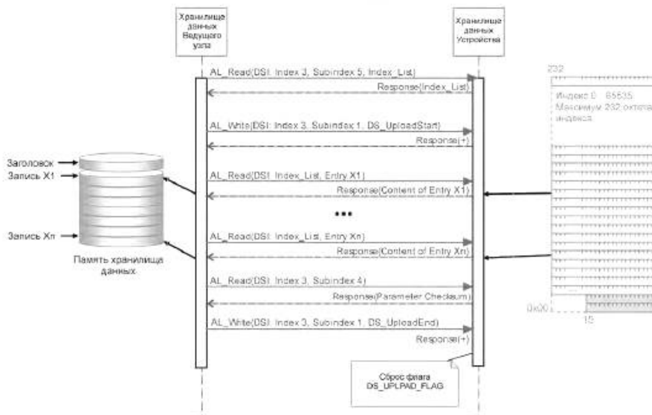
Рисунок 102 — Диаграмма последовательности подкачки в DS
