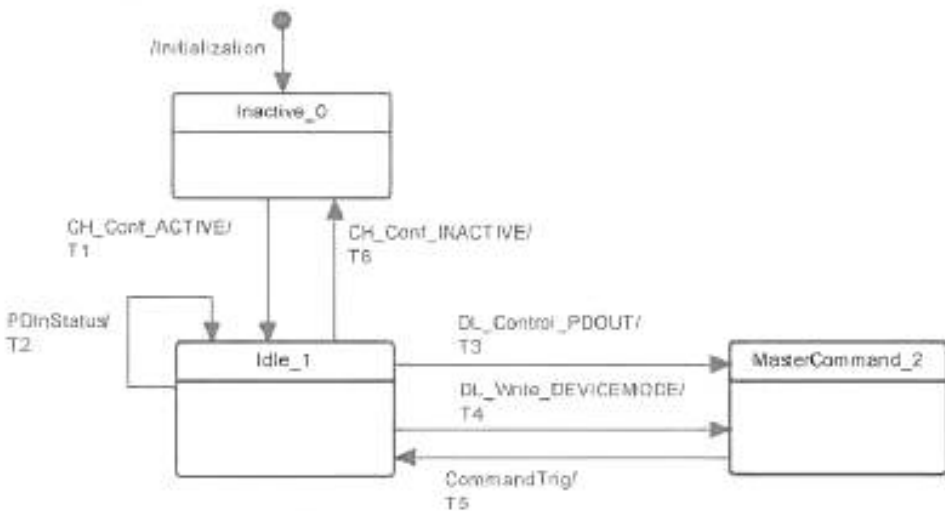
Рисунок 51 — Конечная машина обработчика команд на Ведущем узле
