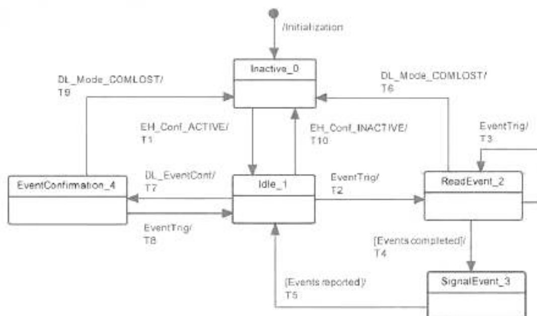
Рисунок 53 — Конечная машина обработчика Событий на Ведущем узле
