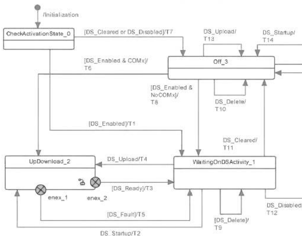
Рисунок 99 — Основная конечная машина механизма DS
