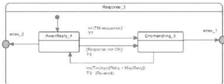
Рисунок 39 — Функциональный блок «Response 3» обработчика прерываний
