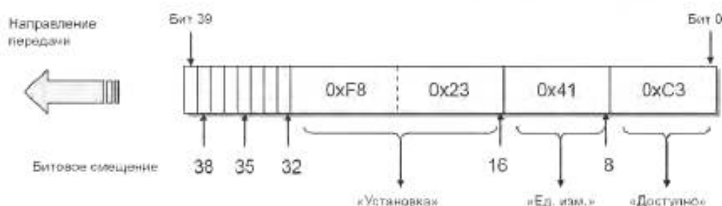
Рисунок Е.8 — Пример 3 структуры типа данных RecordT
