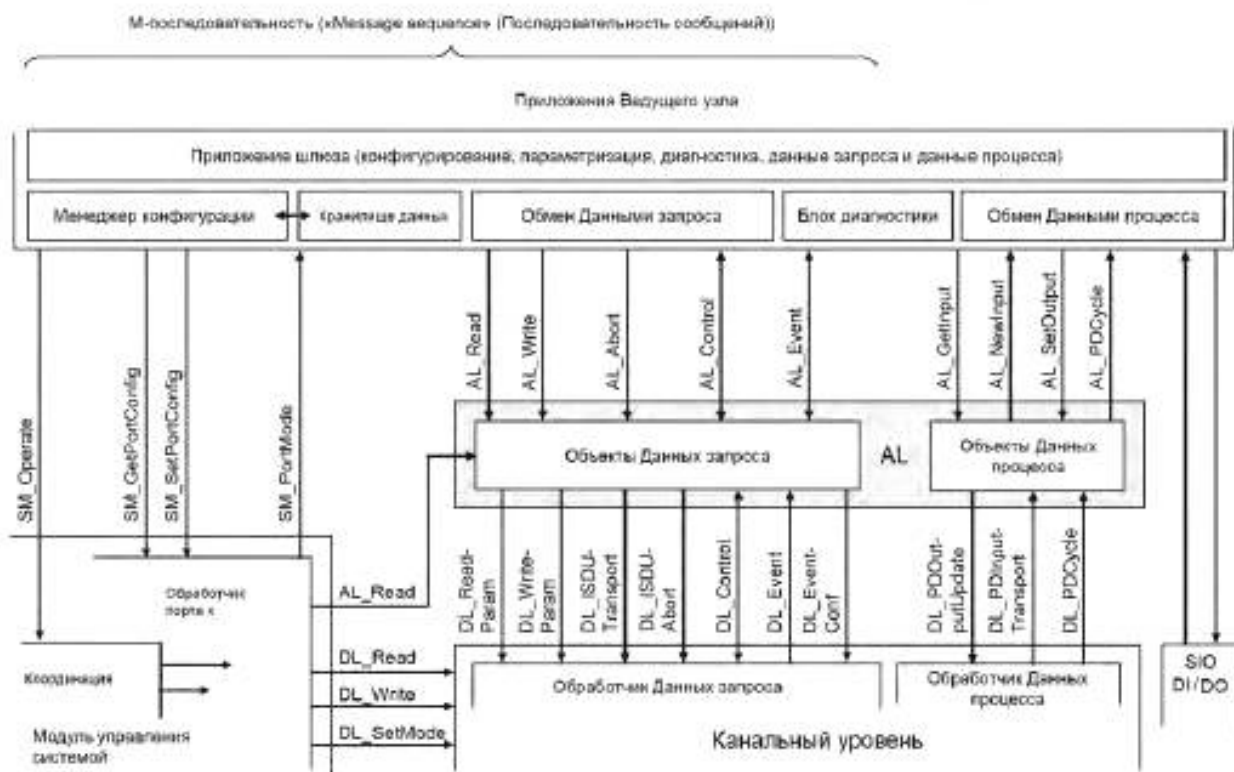
Рисунок 55 — Структура и услуги AL (Ведущий узел)
