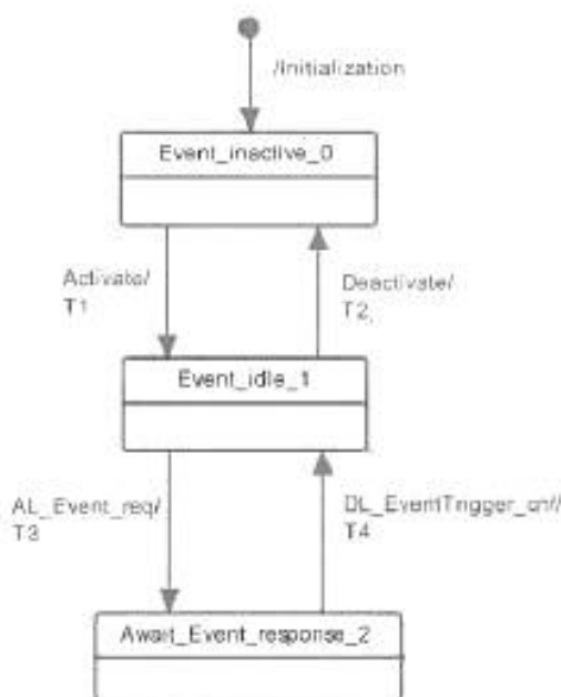
Рисунок 63 — Конечная машина Событий прикладного уровня на Устройстве
