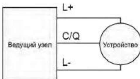
Рисунок 9 — Система 3-проводного соединения
