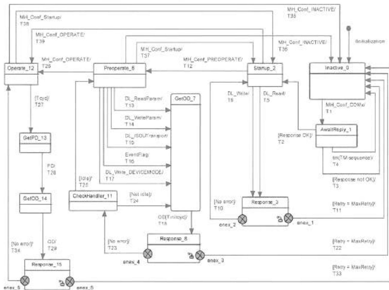
Рисунок 38 — Конечная машина обработчика сообщений Ведущего узла
