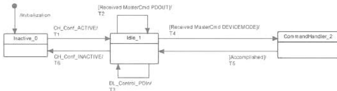
Рисунок 52 — Конечная машина обработчика команд на Устройстве
