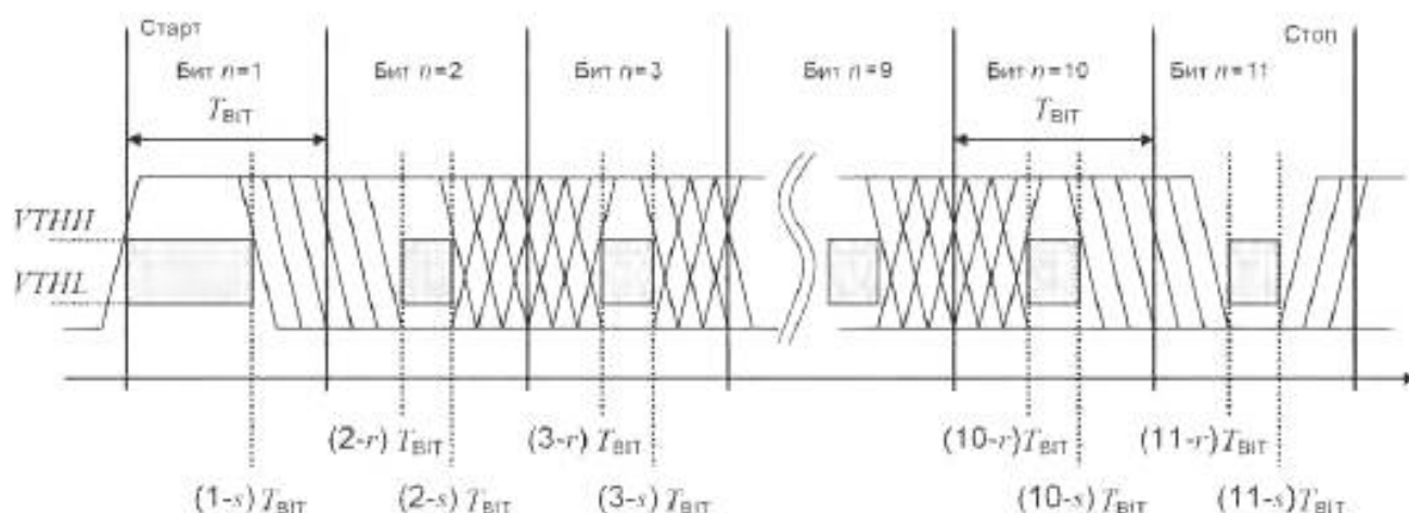
Рисунок 20 — Глазковая диаграмма для правильного обнаружения фрейма UART
