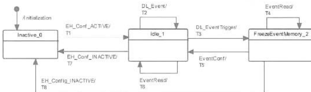
Рисунок 54 — Конечная машина обработчика Событий на Устройстве
