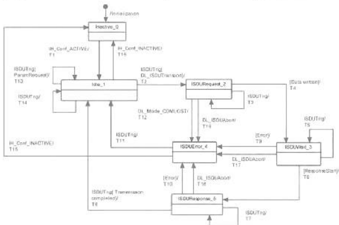
Рисунок 49 — Конечная машина обработчика ISDU на Ведущем узле
