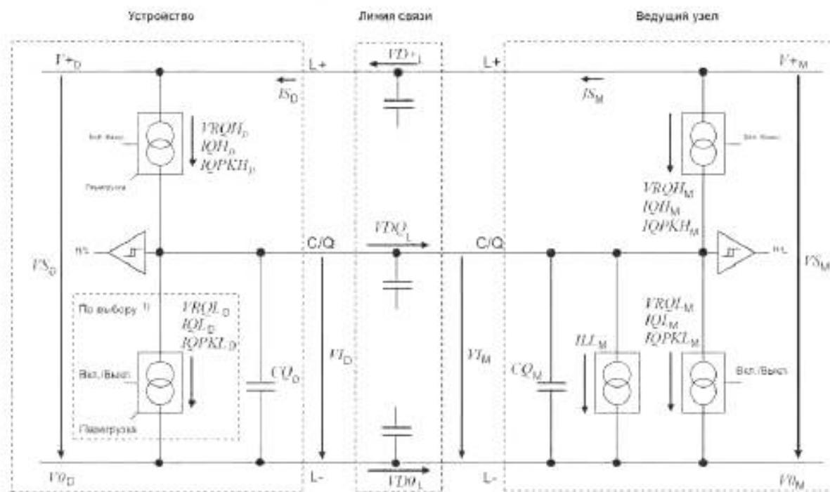
Рисунок 15 — Эталонная схема системы 3-проводного присоединения SDCI
