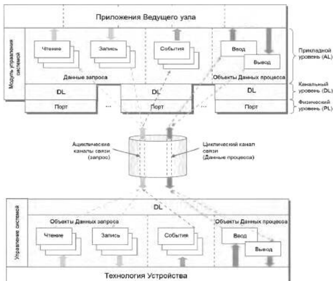
Рисунок 7 — Передача объекта данных на AL
