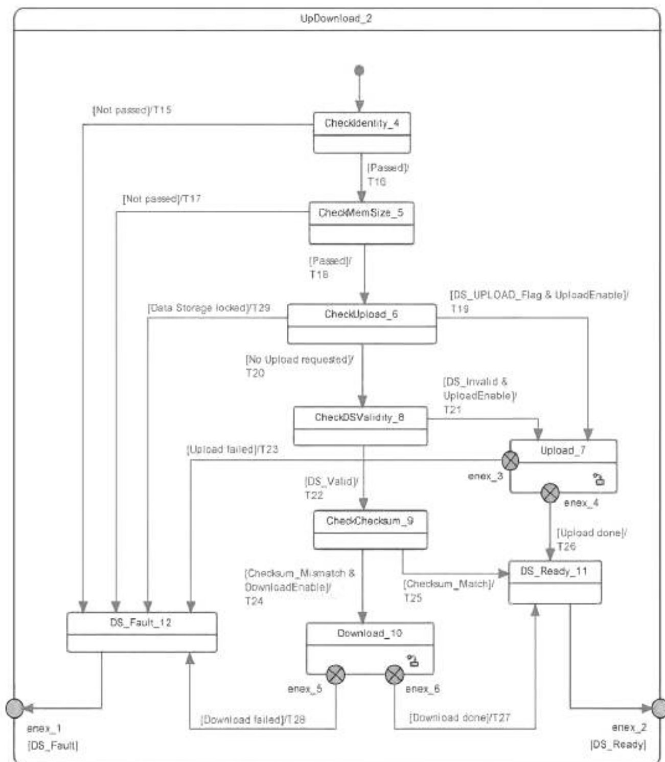
Рисунок 100 — Функциональный блок UpDownload_2 механизма DS
