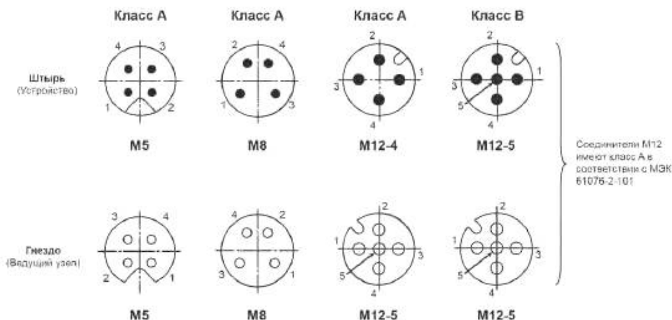
Рисунок 23 — Расположение контактов (вид спереди)
