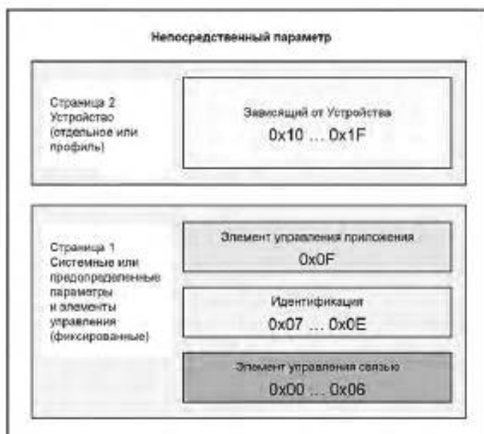
Рисунок В.1 — Классификация и отображение Непосредственных параметров
