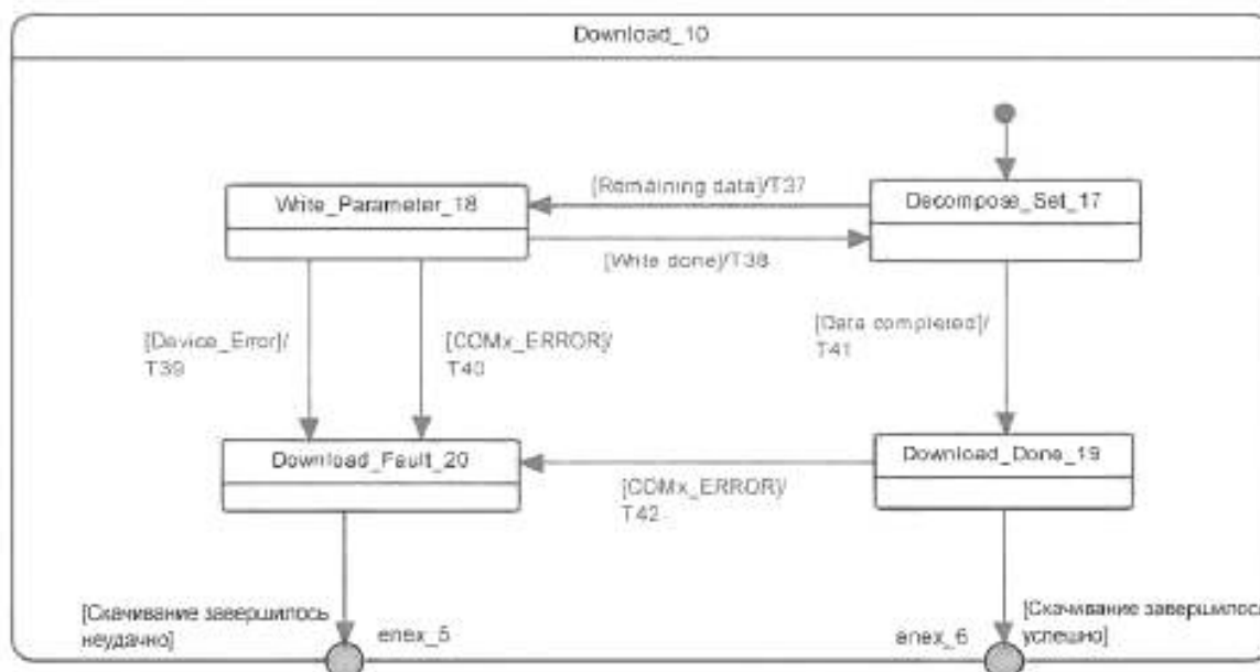
Рисунок 103 — Функциональный блок Download_10 DS
