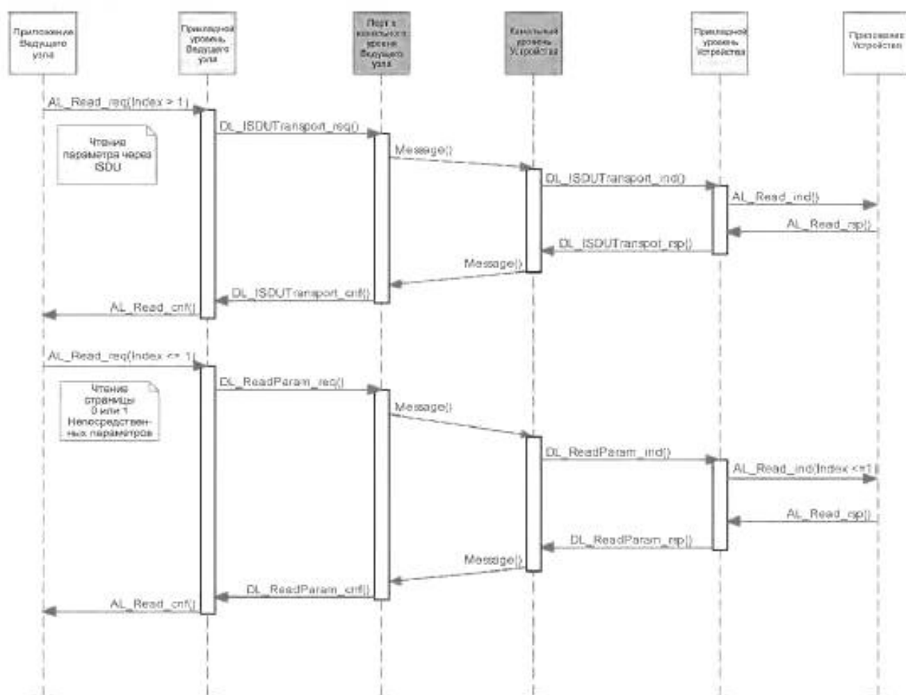
Рисунок 59 — Диаграмма последовательностей при передаче OD
