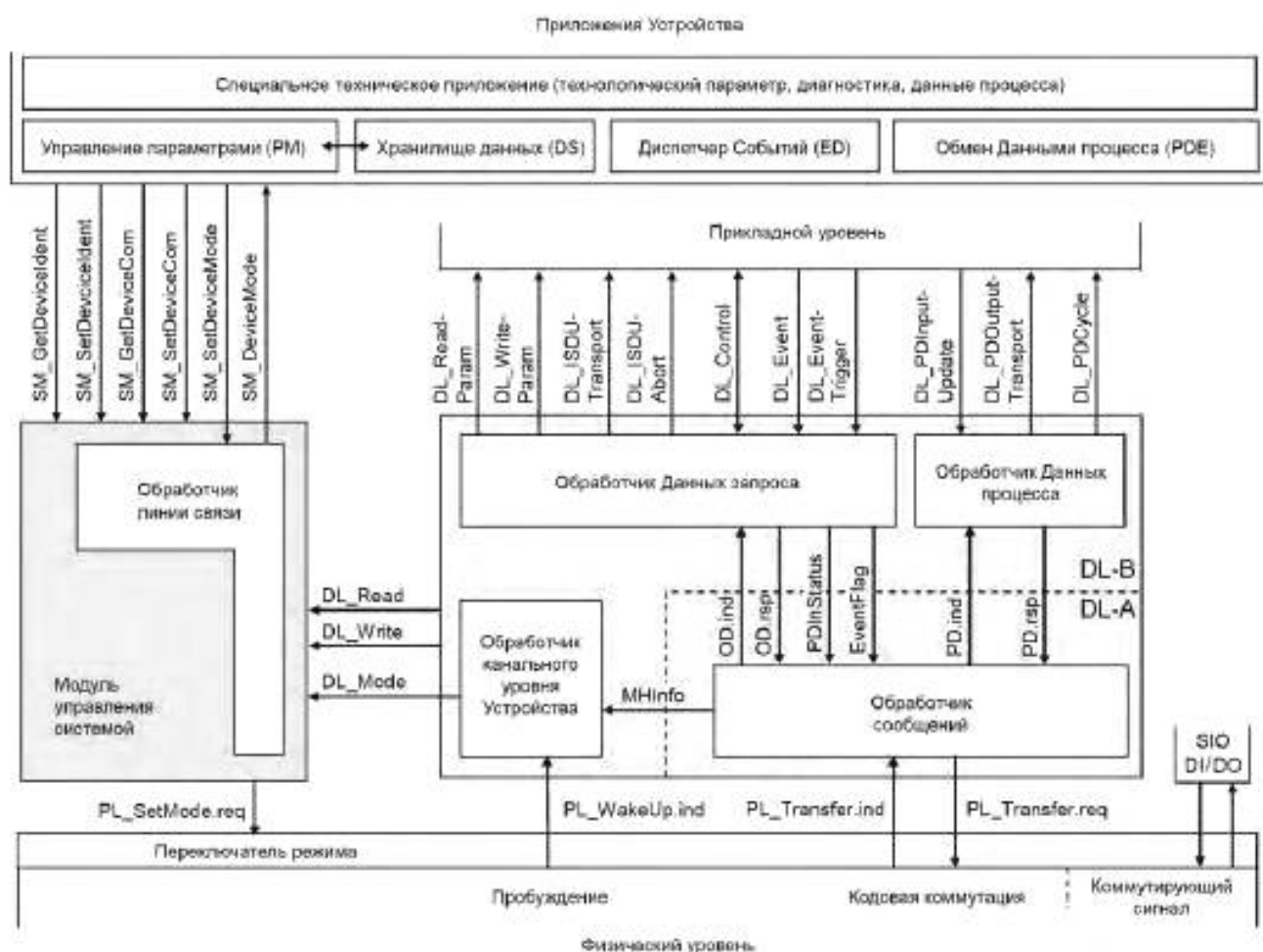
Рисунок 77 — Структура и услуги SM на Устройстве
