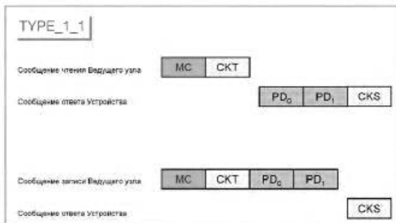
Рисунок А.6 — М-последовательность типа TYPE_1_1
