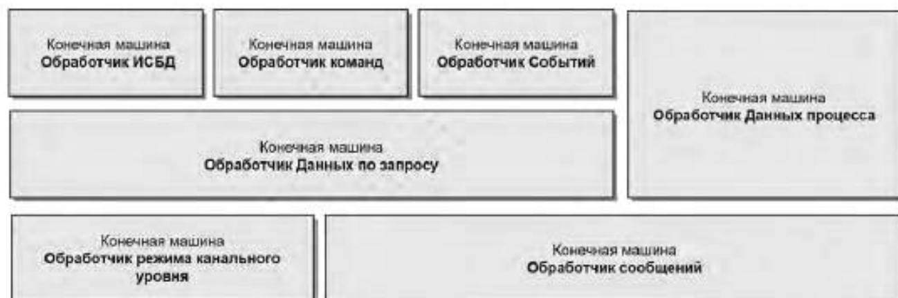
Рисунок 28 — Конечные машины канального уровня
