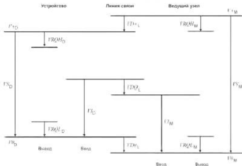
Рисунок 16 — Определения уровня напряжения
