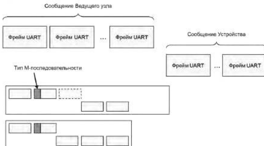
Рисунок 36 — Последовательности сообщений SDCI
