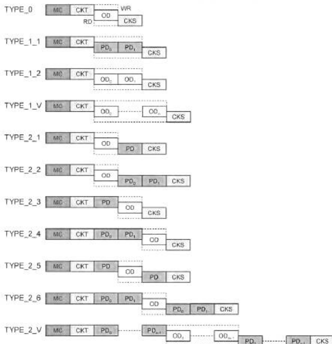
Рисунок 37 — Обзор типов М-последовательностей
