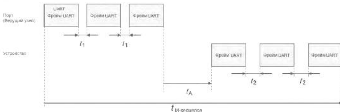
Рисунок А.16 — Временные соотношения М-последовательности
