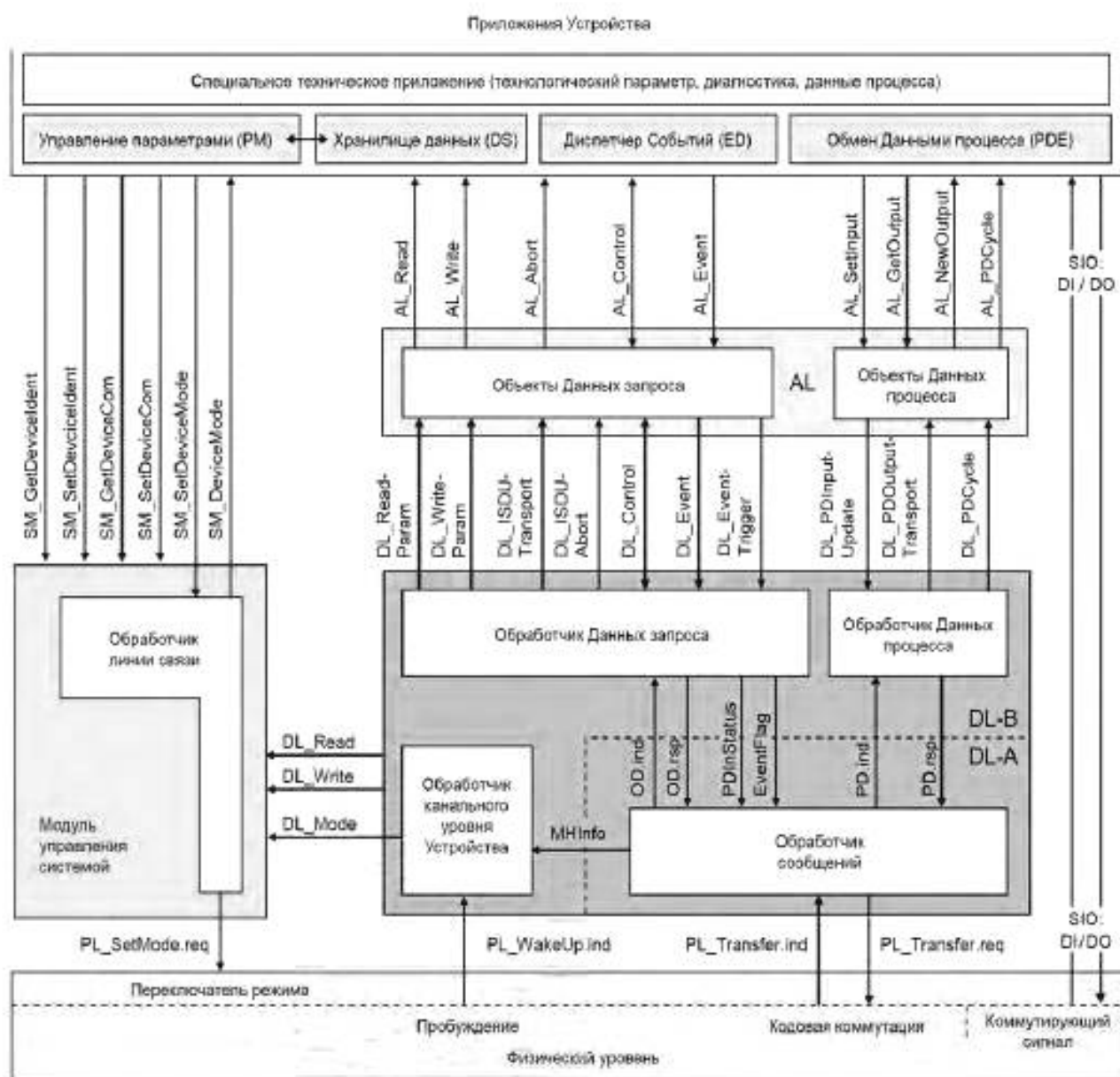
Рисунок 83 — Структура и услуги устройства
