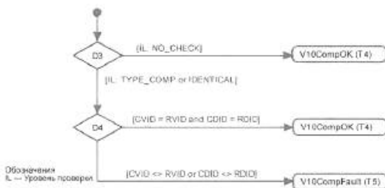
Рисунок 72 — Действия для состояния CheckV10
