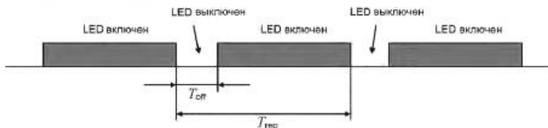
Рисунок 92 — Временные интервалы LED-индикатора Устройства
