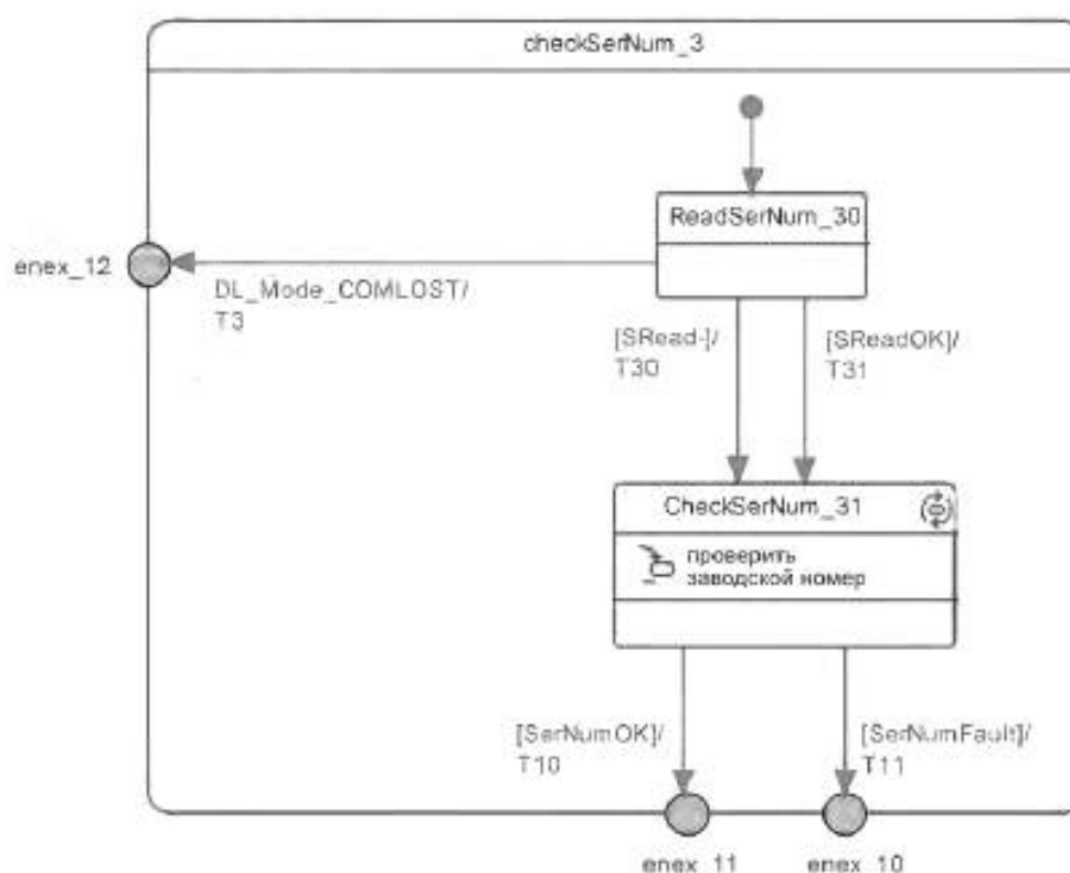
Рисунок 75 — Функциональный блок CheckSerNum_3 SM на Ведущем узле
