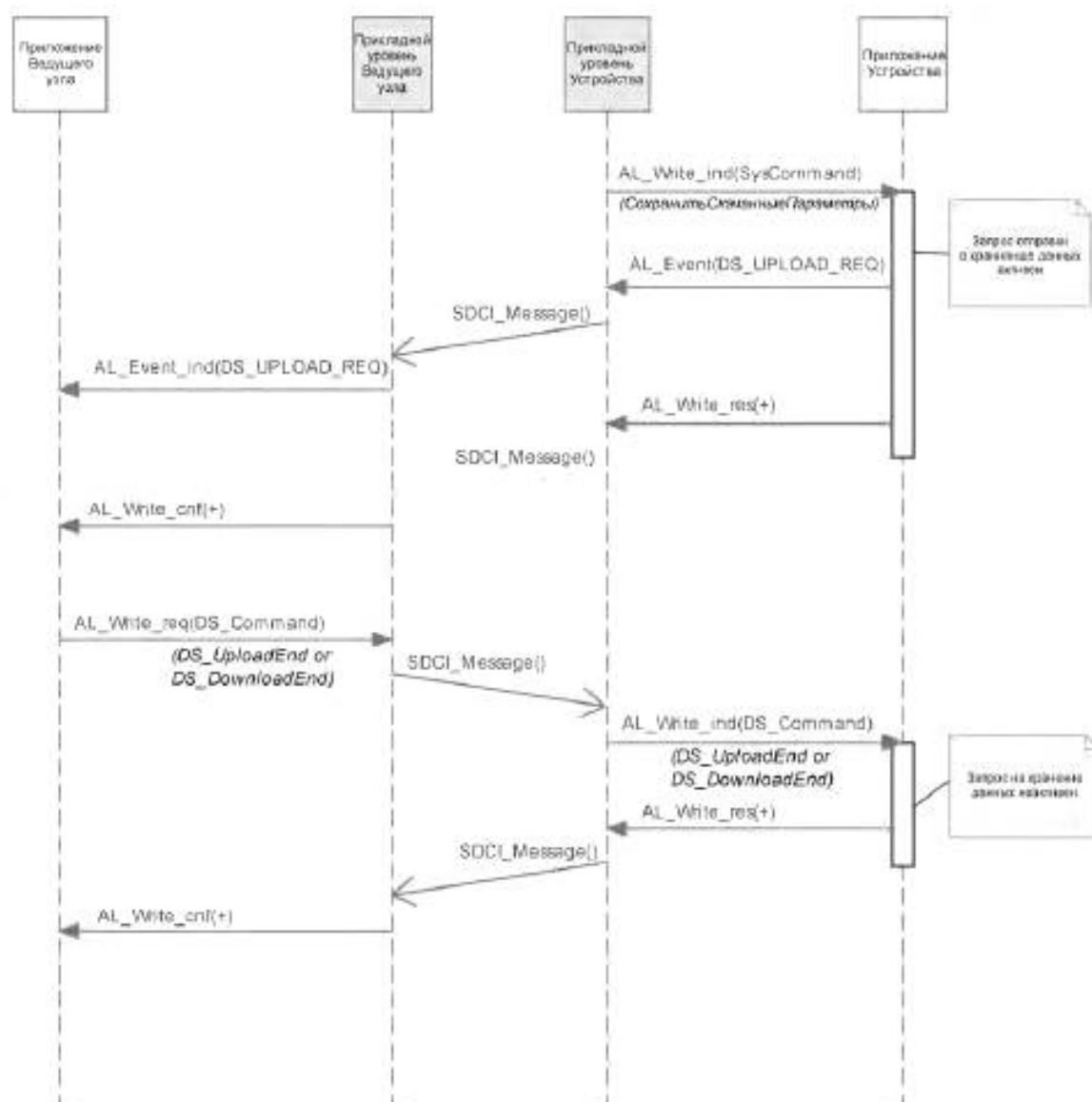
Рисунок 89 — Последовательность сообщений запроса DS
