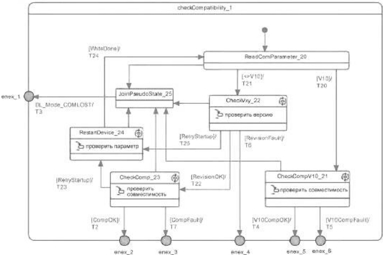
Рисунок 70 — Функциональный блок CheckCompatibility_1 на Ведущем узле
