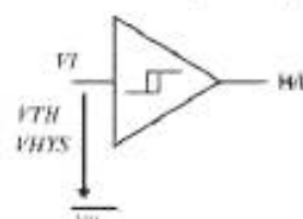
Рисунок 14 — Эталонная схема приемника
