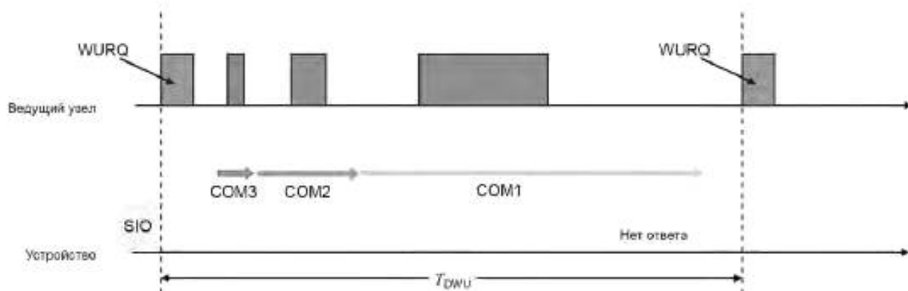
Рисунок 30 — Неудачная попытка установления связи
