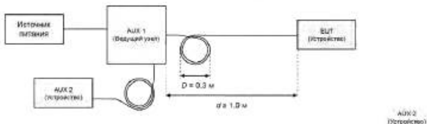
Рисунок G.5 — Установка для испытаний на устойчивость к электростатическим разрядам (Устройство)
