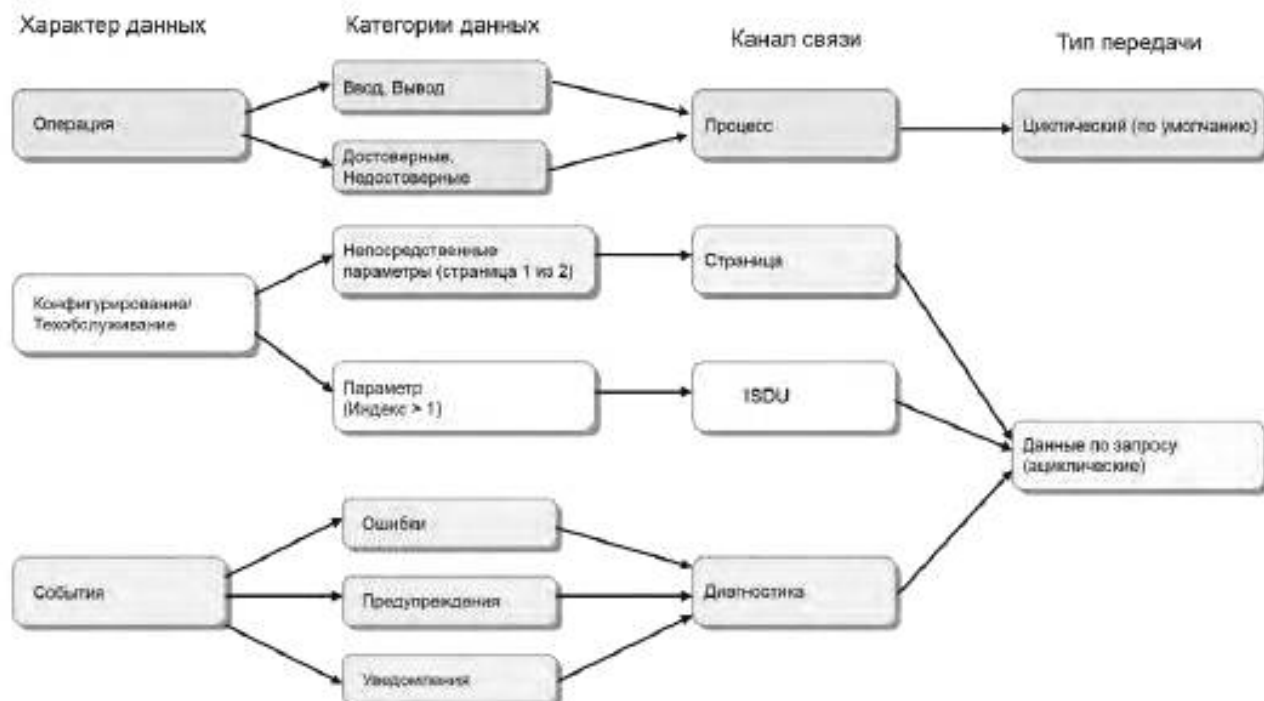
Рисунок 6 — Отношения между характеристиками данных и типами передачи
