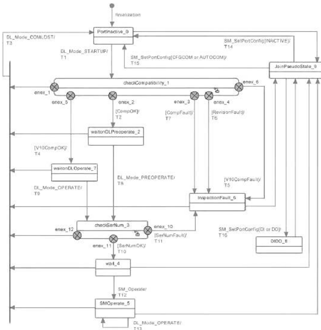
Рисунок 69 — Структура и услуги SM на Ведущем узле
