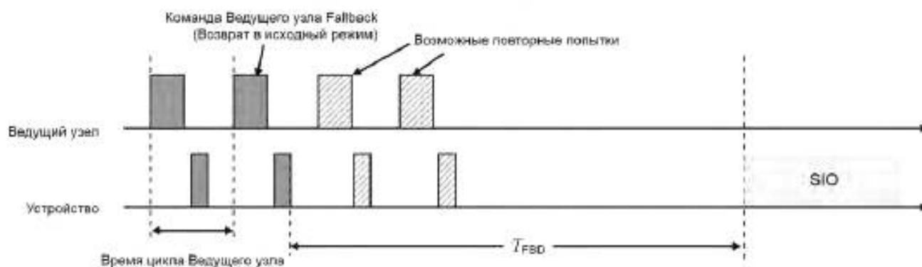
Рисунок 32 — Процедура возврата в исходный режим
