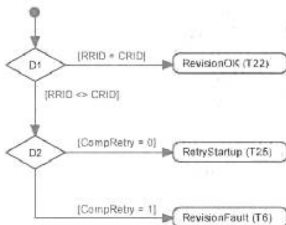
Рисунок 71 — Действия для состояния CheckVxy
