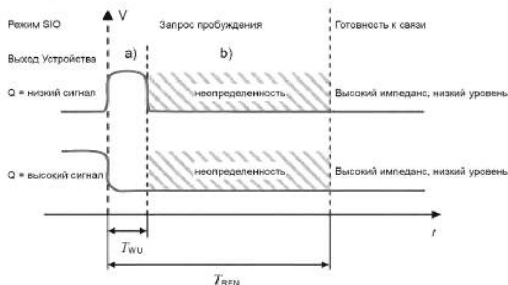
Рисунок 21 — Запрос пробуждения
