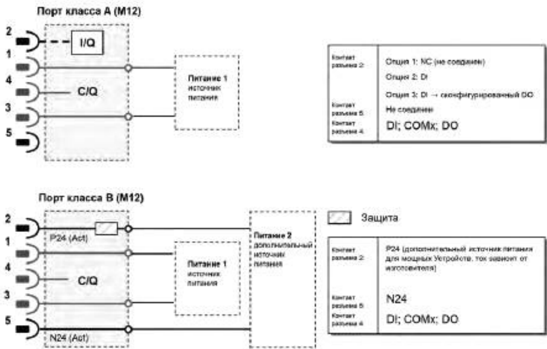
Рисунок 24 — Определения портов классов А и В
