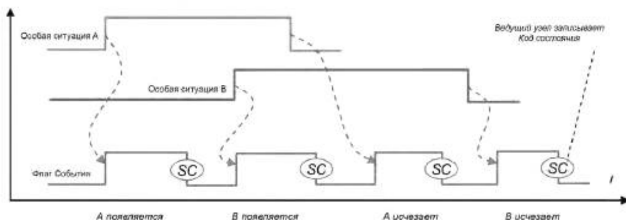
Рисунок 91 — Поток ошибок в случае последовательных ошибок
