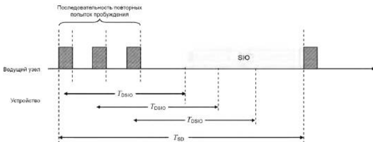
Рисунок 31 — Стратегия повторных попыток установления связи
