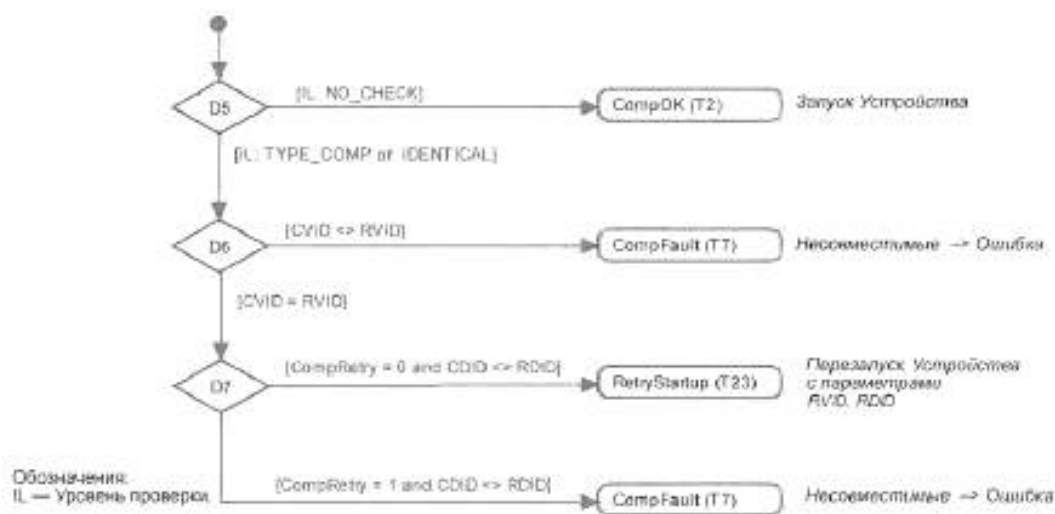
Рисунок 73 — Действия для состояния CheckComp
