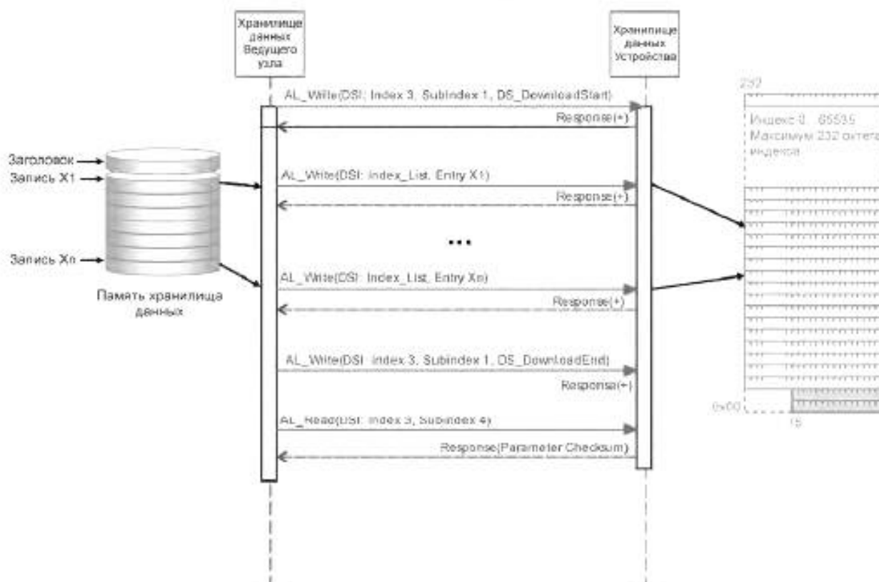
Рисунок 104 — Диаграмма последовательности скачивания из DS
