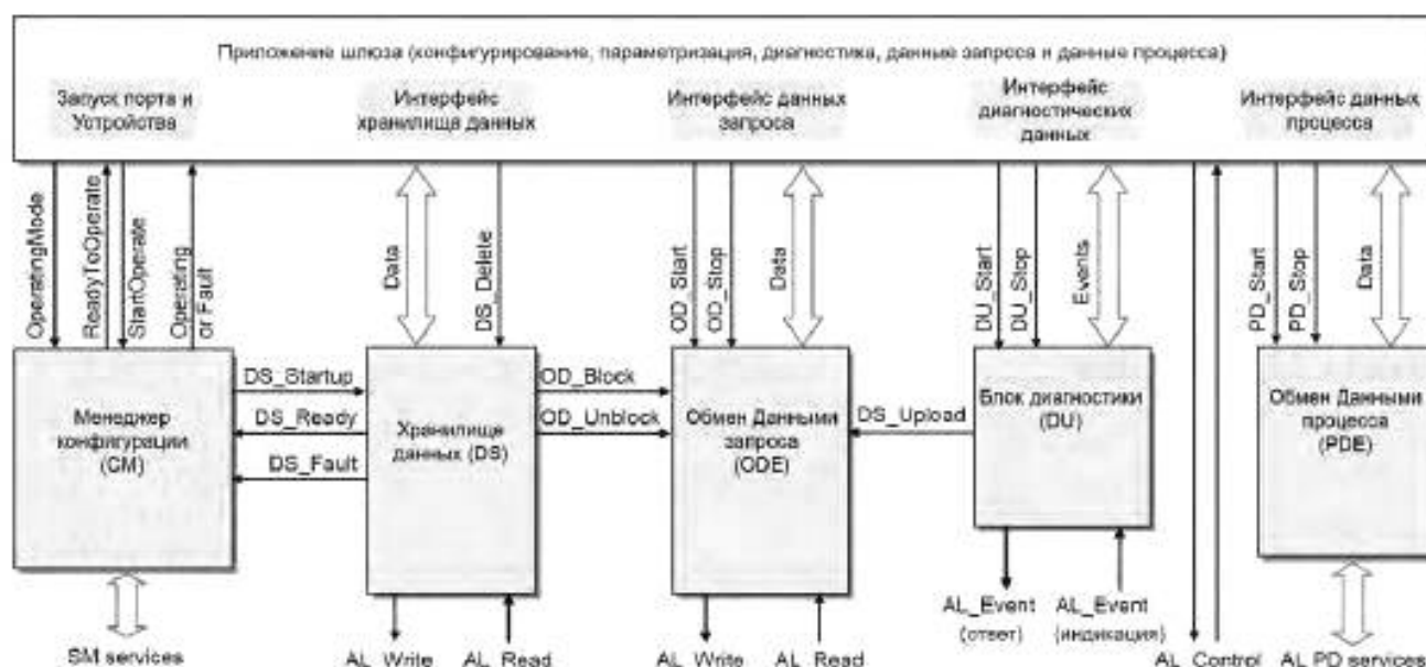
Рисунок 95 — Взаимоотношения общих приложений Ведущего узла
