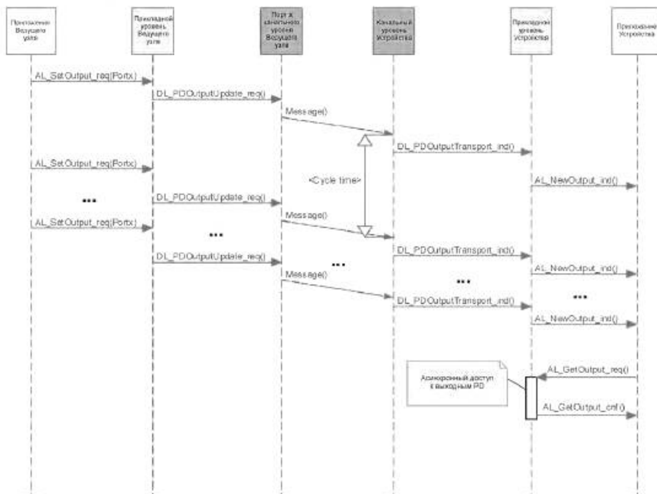
Рисунок 65 — Диаграмма последовательностей для выходных PD
