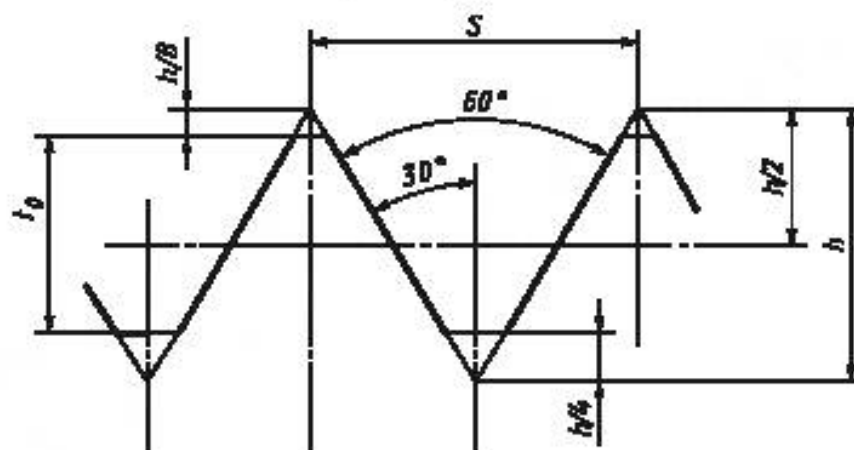
Метрическая резьба ИСО
