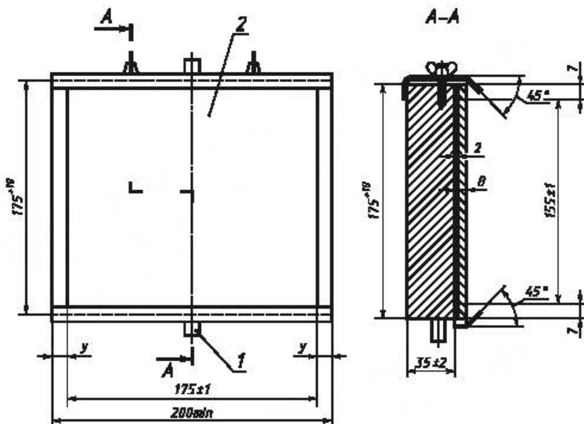
Рисунок 16 — Монтажная опора
