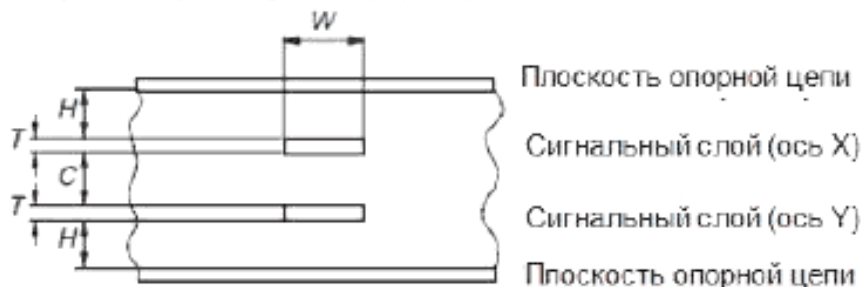
Рисунок 7 – Двойная (асимметричная) полосковая линия
