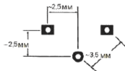
Единый тест-купон волнового сопротивления Схема образца 1В
