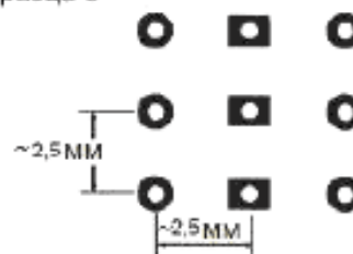
Единый тест-купон волнового сопротивления Схема образца 3
