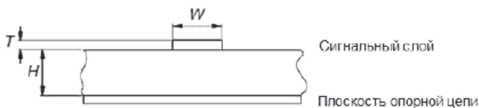
Рисунок 4 – Поверхностная микрополосковая линия
