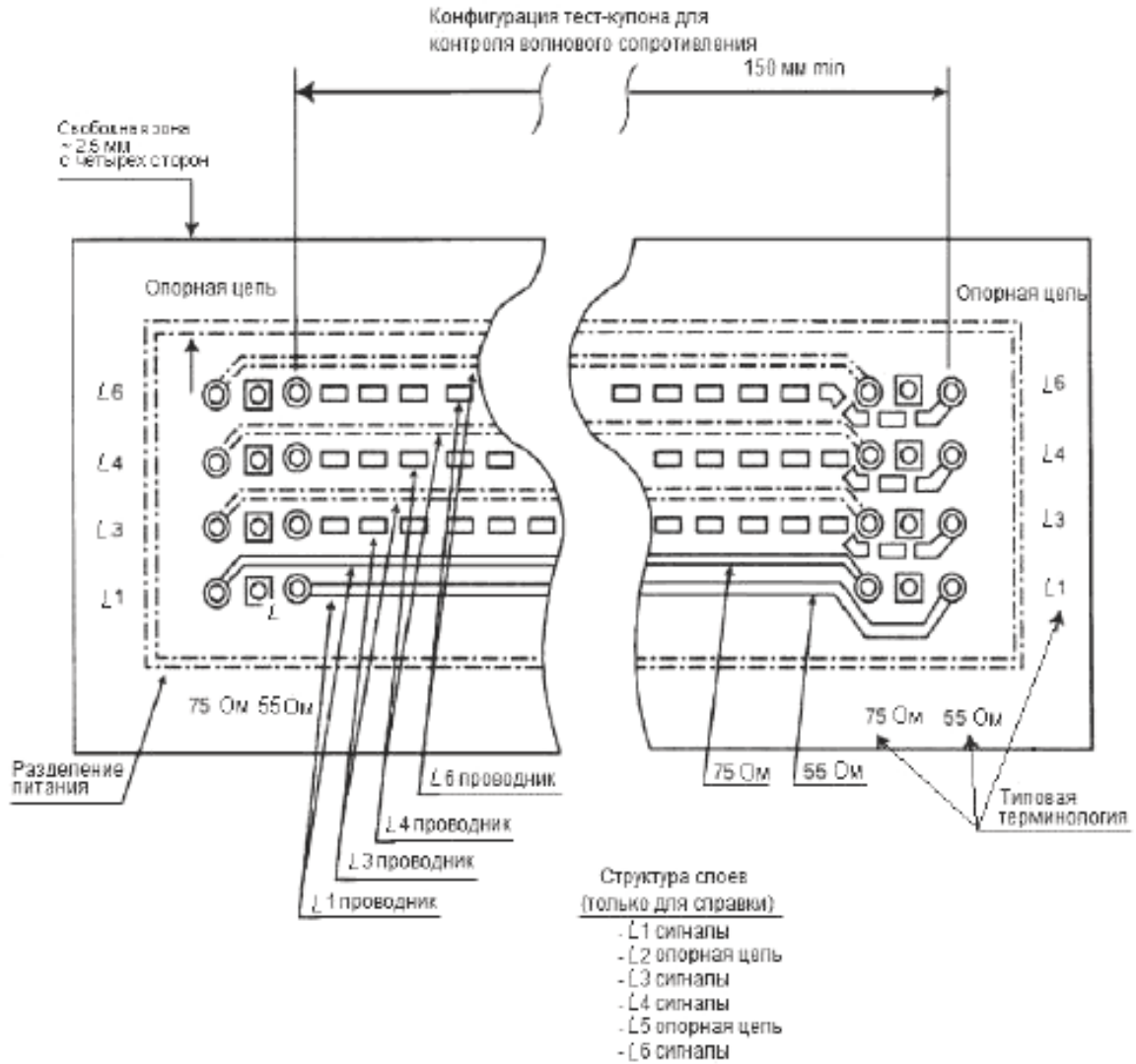
Рисунок 10 – Тест-кулон контролируемого волнового сопротивления
