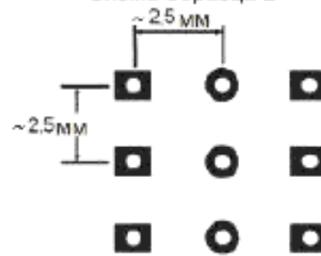
Единый тест-купон волнового сопротивления Схема образца 2
