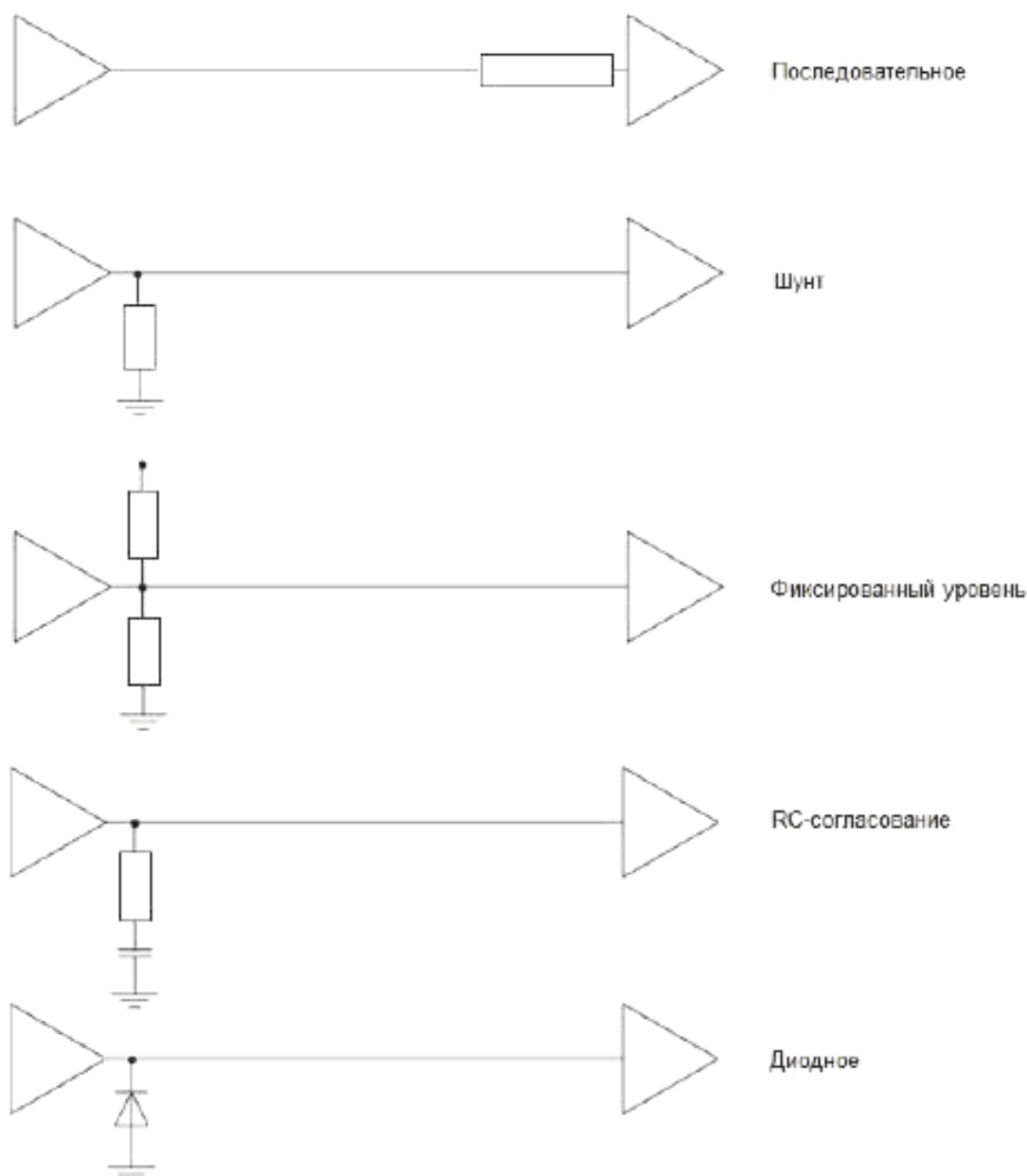
Рисунок 3 – Согласование нагрузок
