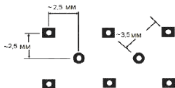
Единый тест-купон волнового сопротивления Схема образца 1А
