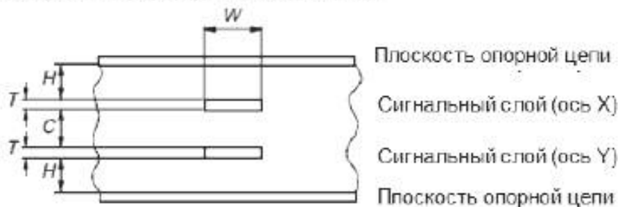
Рисунок 7 – Двойная (асимметричная) полосковая линия
