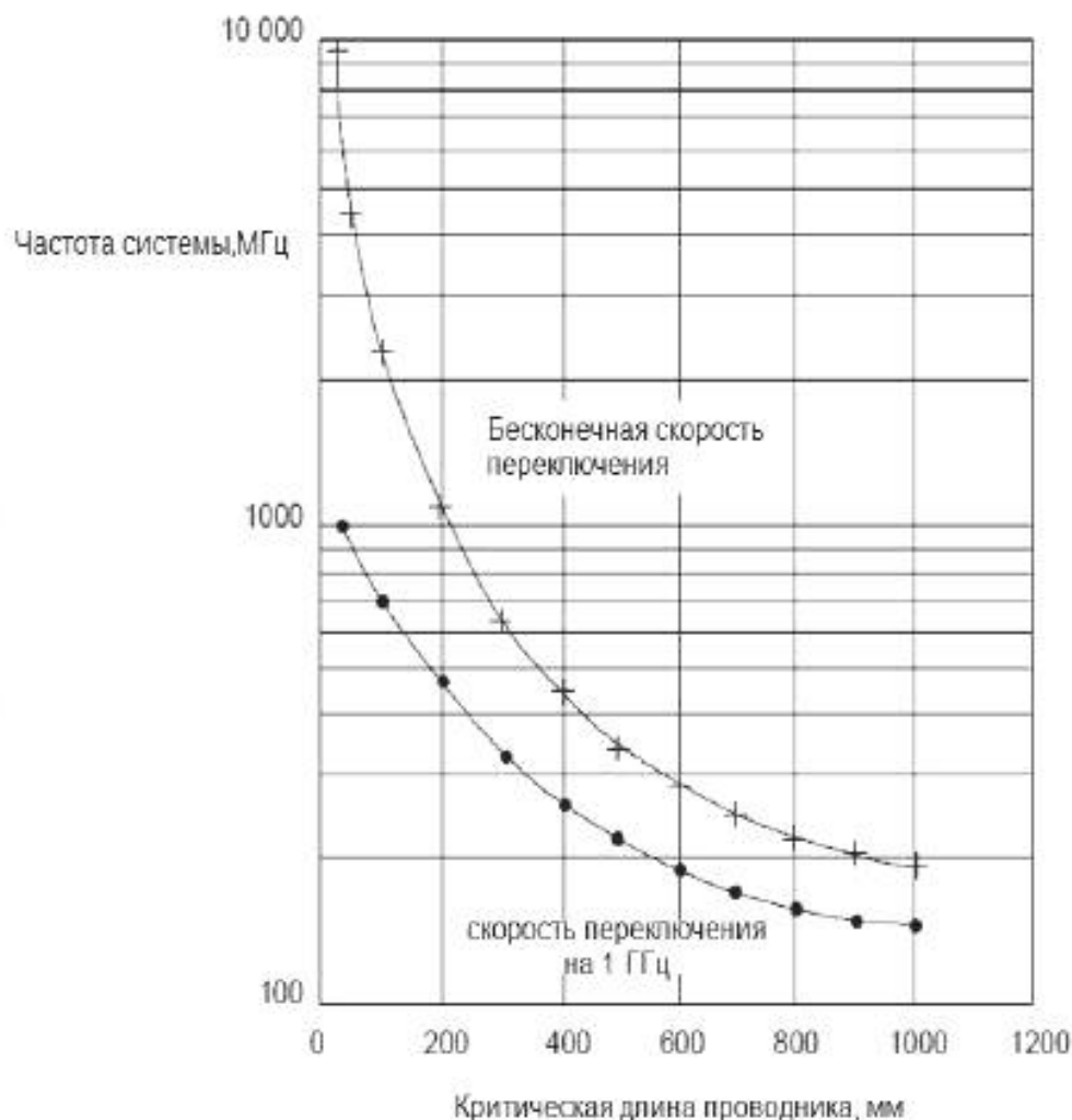
Рисунок 1 – Зависимость скорости переключения от временной задержки
