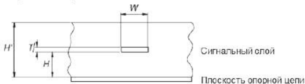
Рисунок 5 – Встроенная микрополосковая линия
