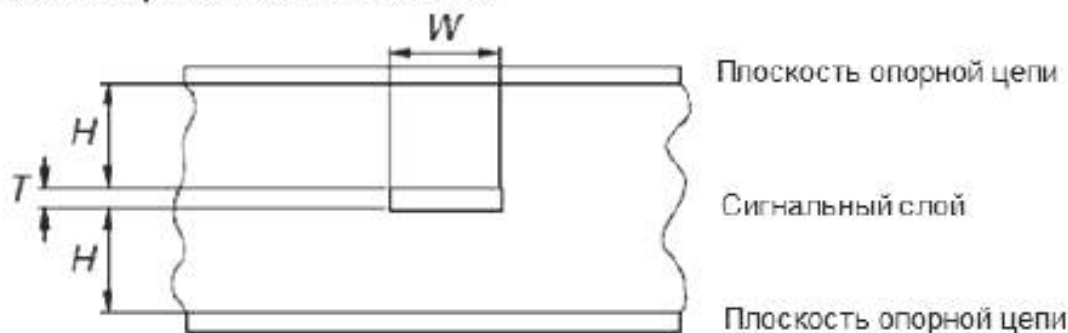
Рисунок 6 – Симметричная полосковая линия
