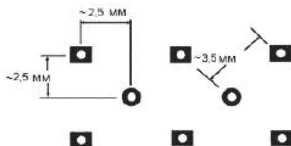
Единичный тест-купон волнового сопротивления Схема образца 1А
