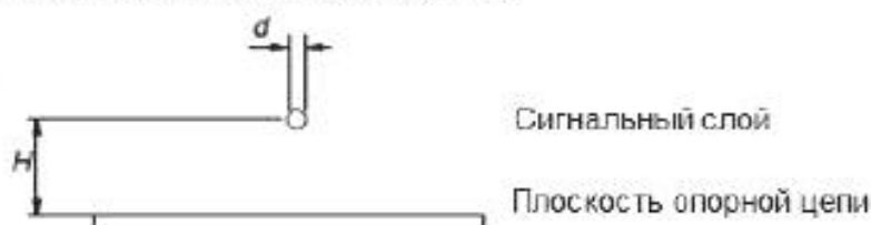
Рисунок 9 – Микрополосковая проводная линия
