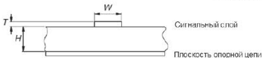
Рисунок 4 – Поверхностная микрополосковая линия
