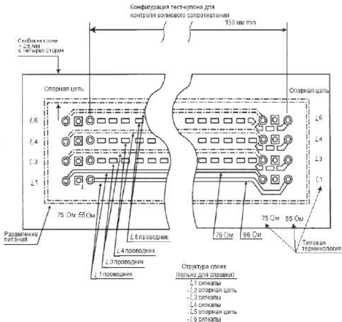
Рисунок 10 – Тест-кулон контролируемого волнового сопротивления
