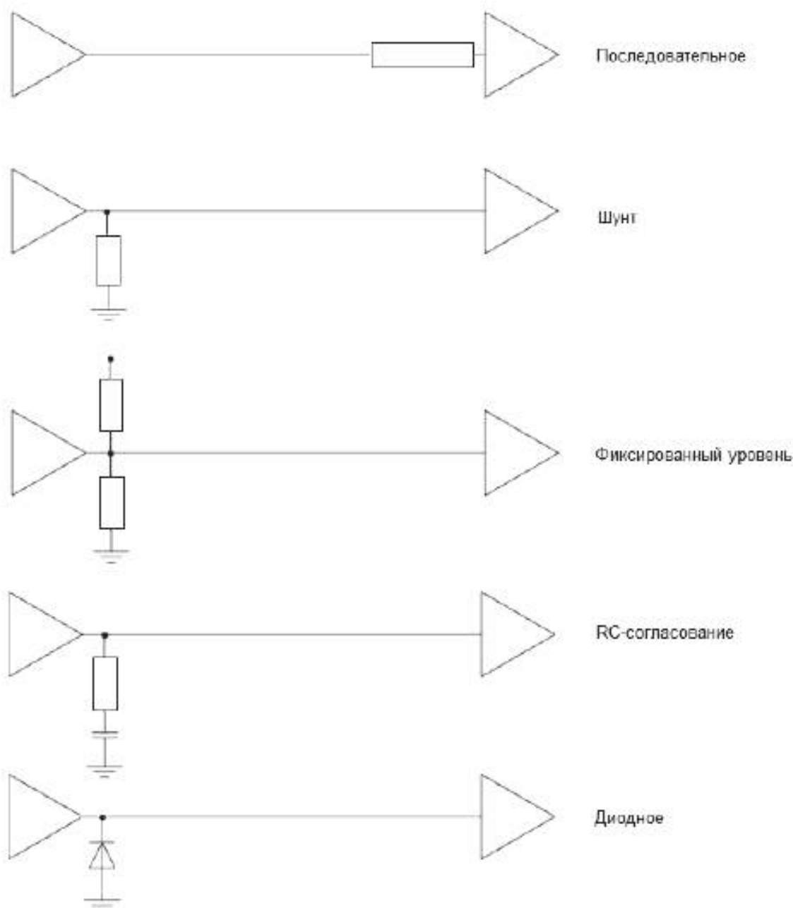
Рисунок 3 – Согласование нагрузок
