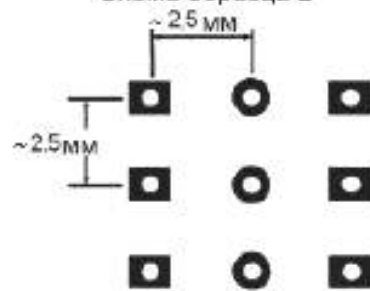
Единичный тест-купон волнового сопротивления Схема образца 2
