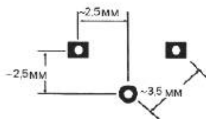
Единичный тест-купон волнового сопротивления Схема образца 1В
