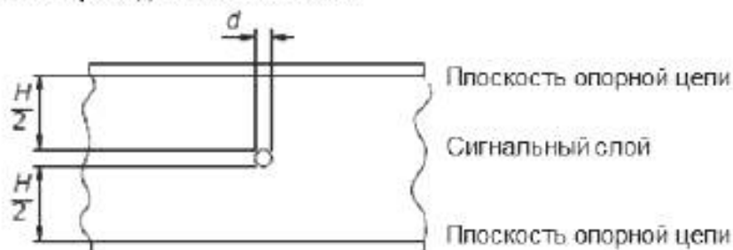
Рисунок 8 – Полосковая проводная линия
