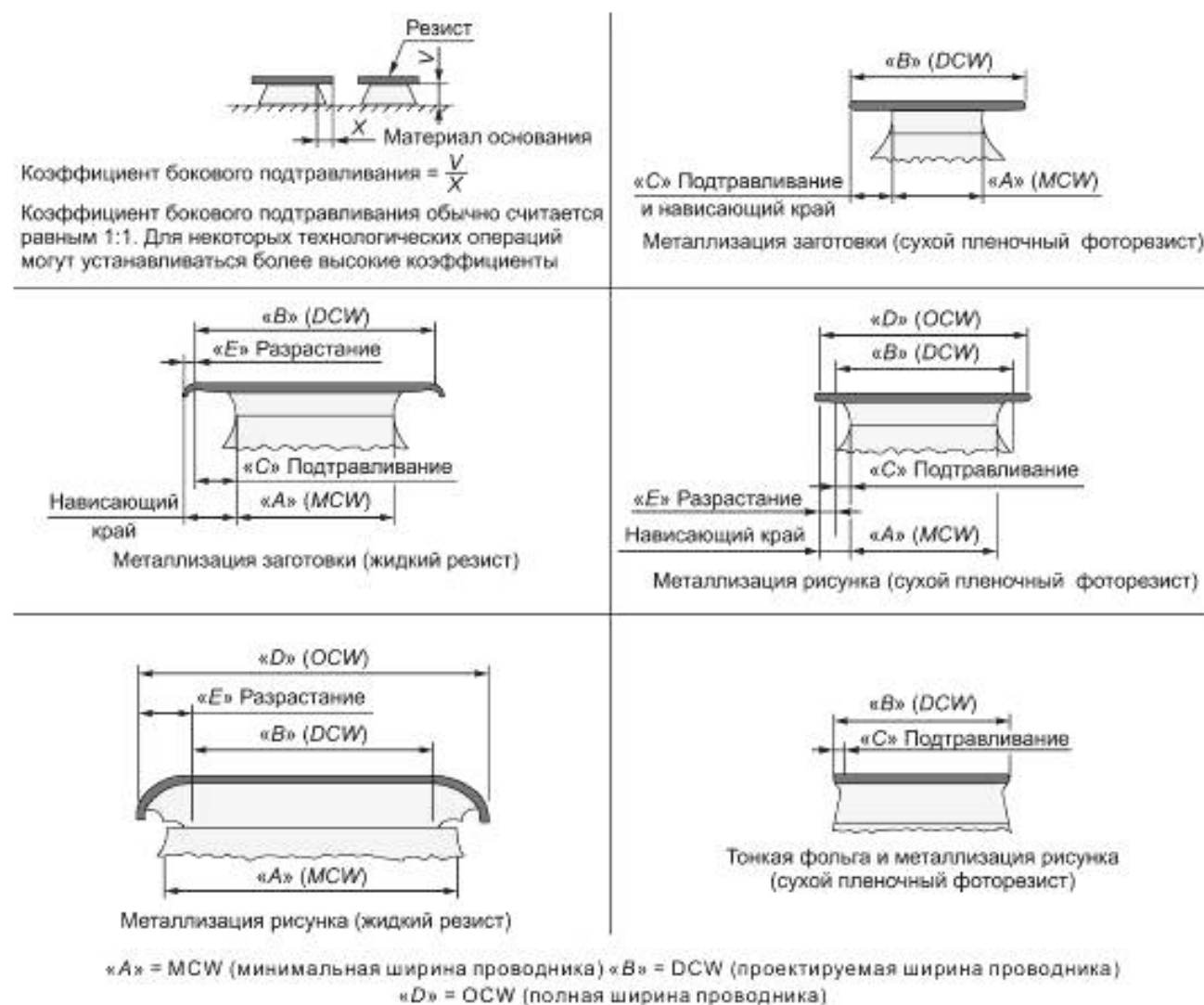
Рисунок 16 — Характеристика проводника
