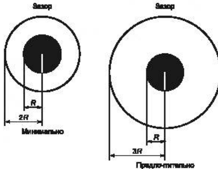
Рисунок 11 — Требования к зазору вокруг реперного знака
