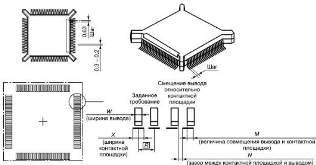
Рисунок 4 — Шаг для многвыводных компонентов
