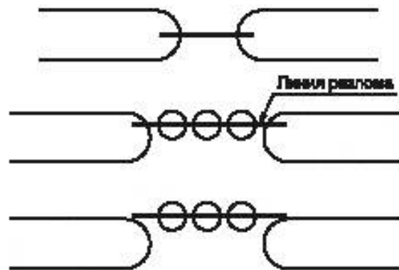
Рисунок 21 — Фрезерованные щели
