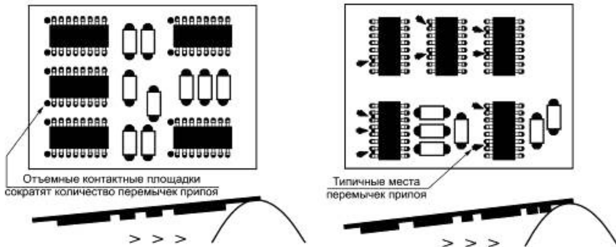
Рисунок 6 — Ориентация компонента для применения пайки волной
