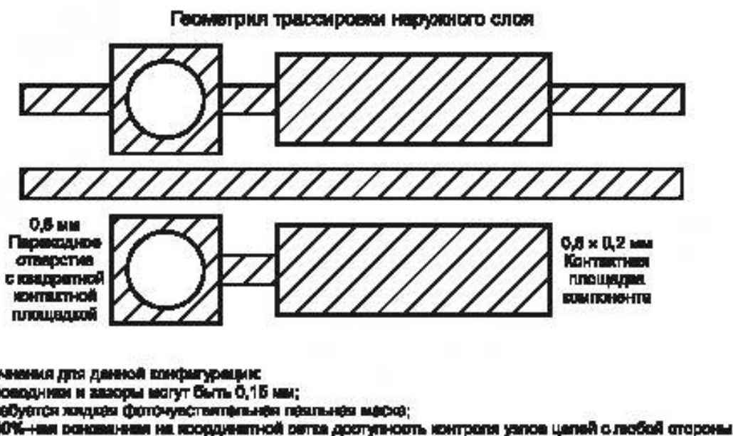
Рисунок 12 — Конфигурации поверхностного монтажа
