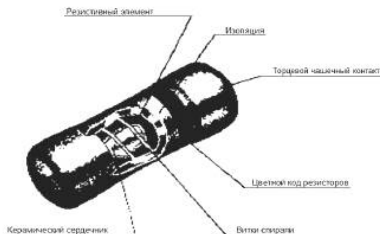
Рисунок 6 – Конструкция безвыводного цилиндрического резистора
