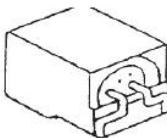
Рисунок 22 – Конструкция безвыводного алюминиевого электролитического конденсатора (горизонтальное исполнение)
