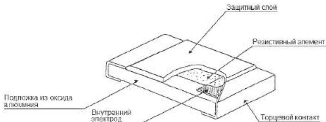
Рисунок 2 – Конструкция прямоугольного безвыводного резистора
