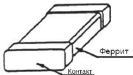
Рисунок 30 – Конструкция безвыводного дросселя
