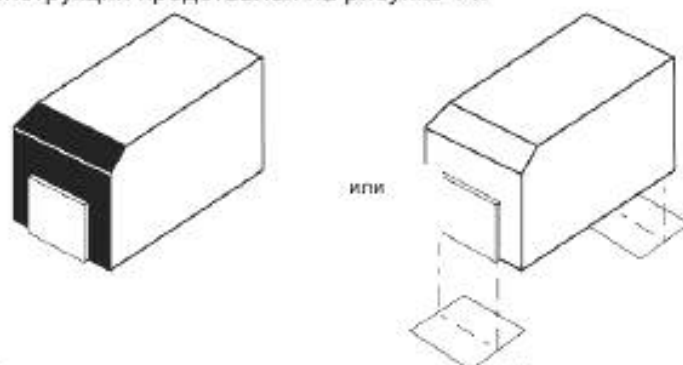
Рисунок 14 – Конструкция постоянного танталового безвыводного конденсатора
