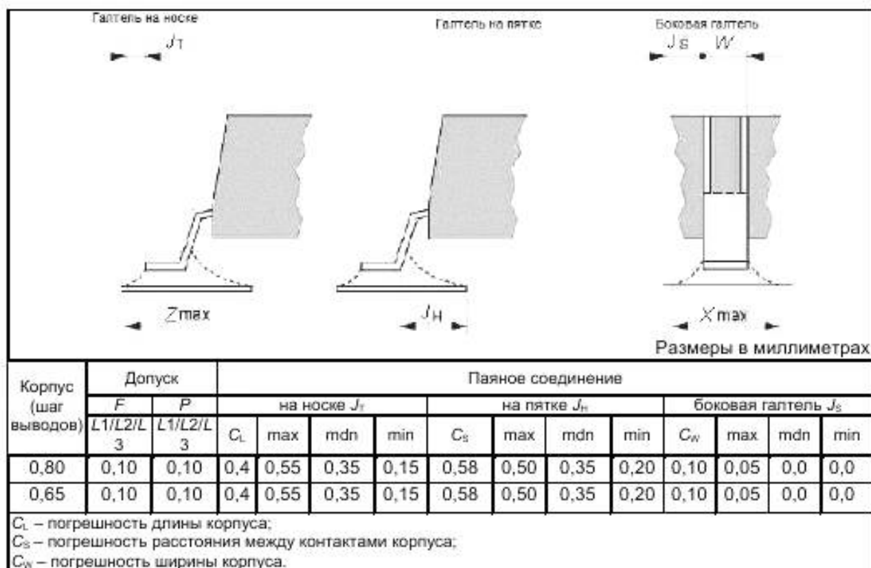
Рисунок 15 – Выступ паяного соединения (см. IEC 61188-5-1, таблицы 2 и 3)
