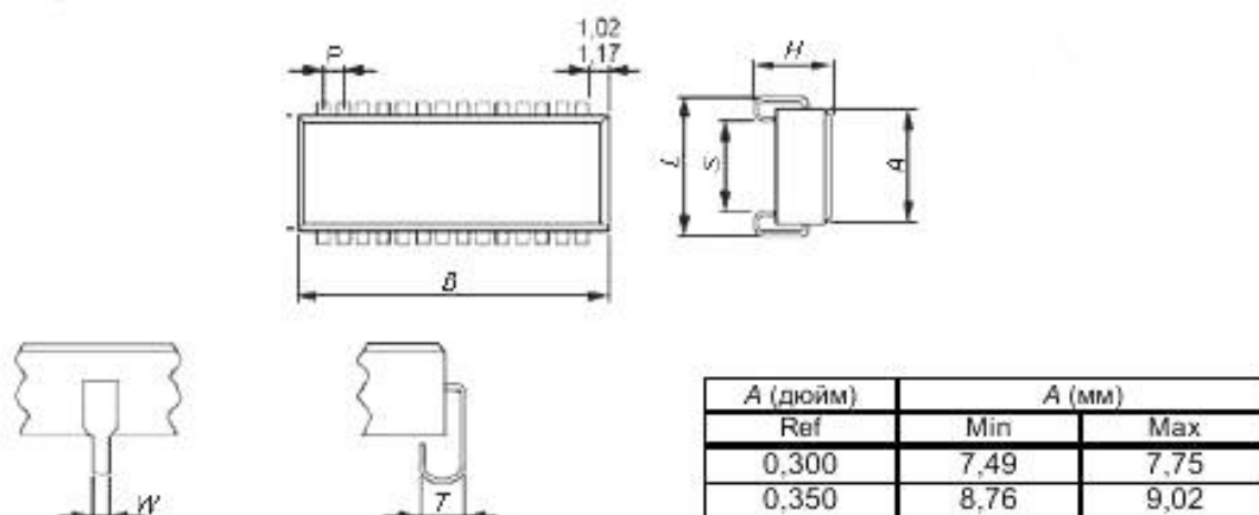
Рисунок 2 – Размеры корпуса SOJ, лист 1
