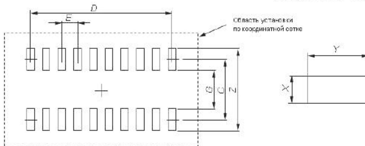
Рисунок 4 – Размеры посадочного места корпуса SOJ, лист 1
