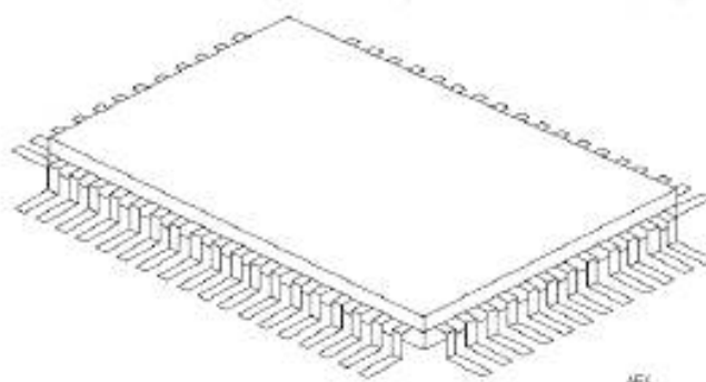
Рисунок 5 — Конструкция корпуса типа PQFP (прямоугольный)
