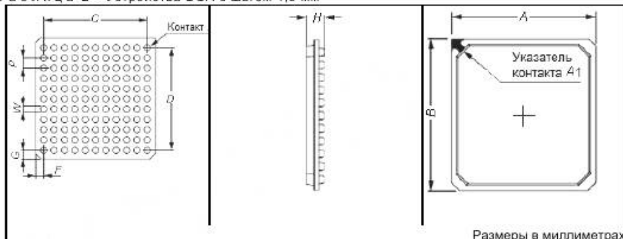
Т а б л и ц а 2 – Устройства BGA с шагом 1,5 мм
