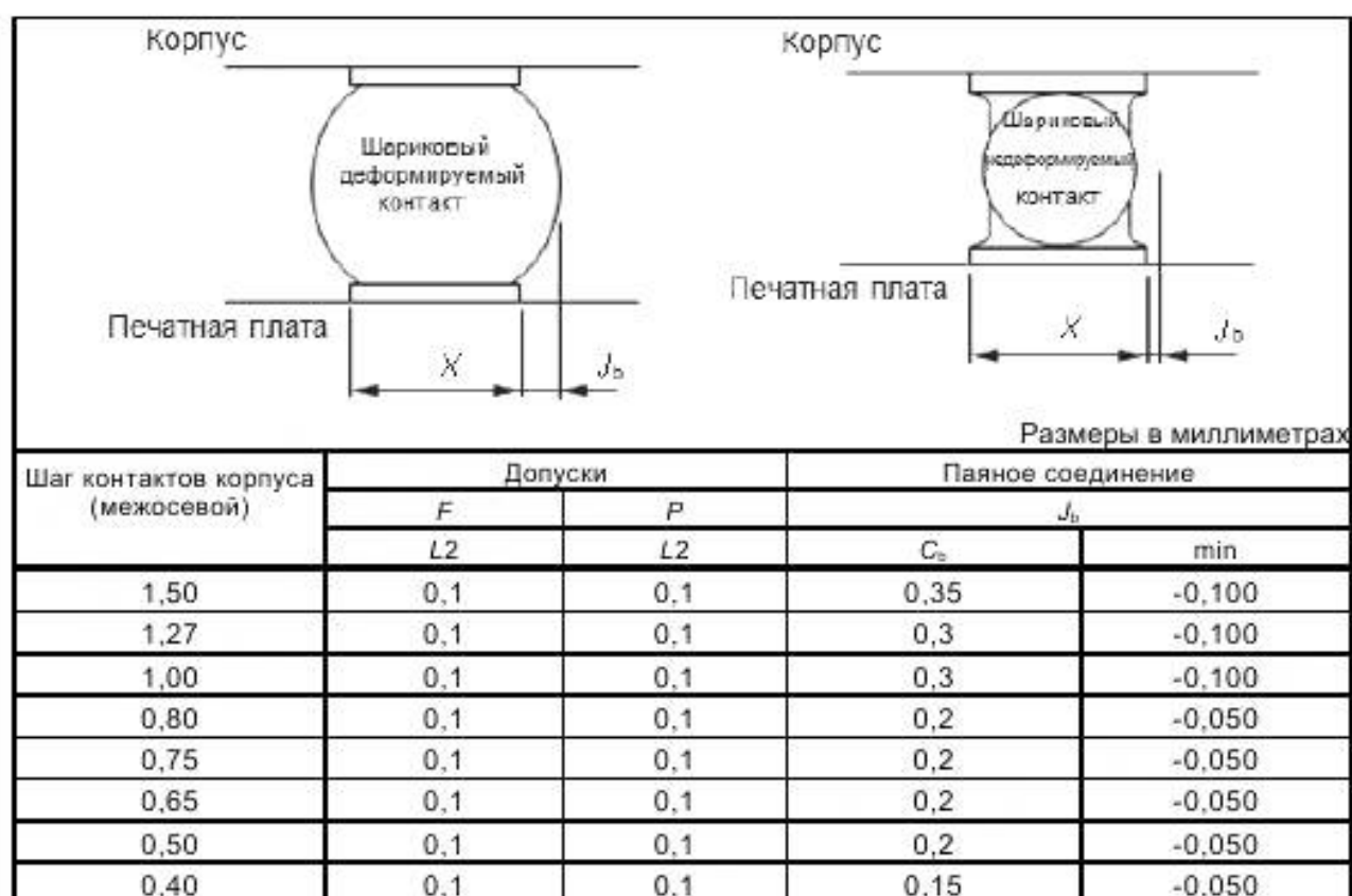
Рисунок 6 – Анализ формы паяного соединения
