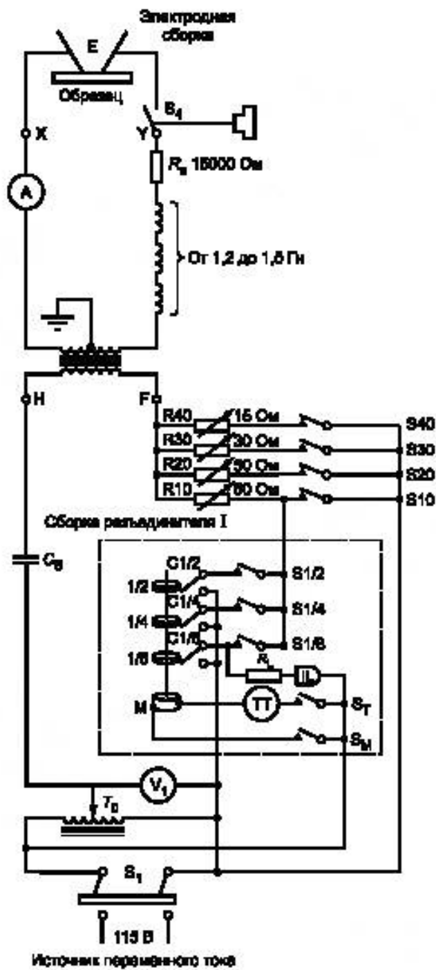
Рисунок 33 — Схема испытания на дугостойкость
