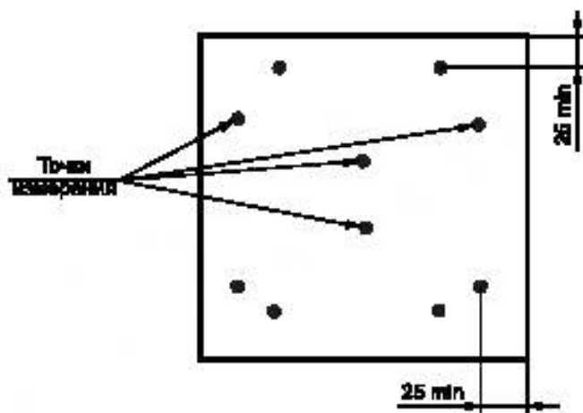
Рисунок 1 — Точки измерения толщины
