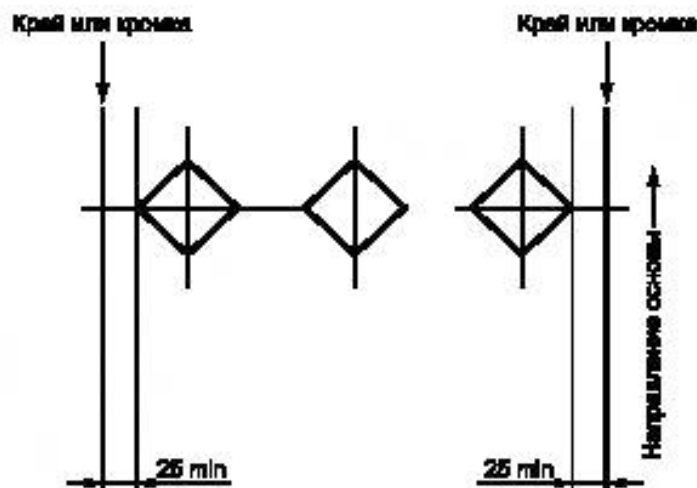
Рисунок 2 — Места вырезки образцов
