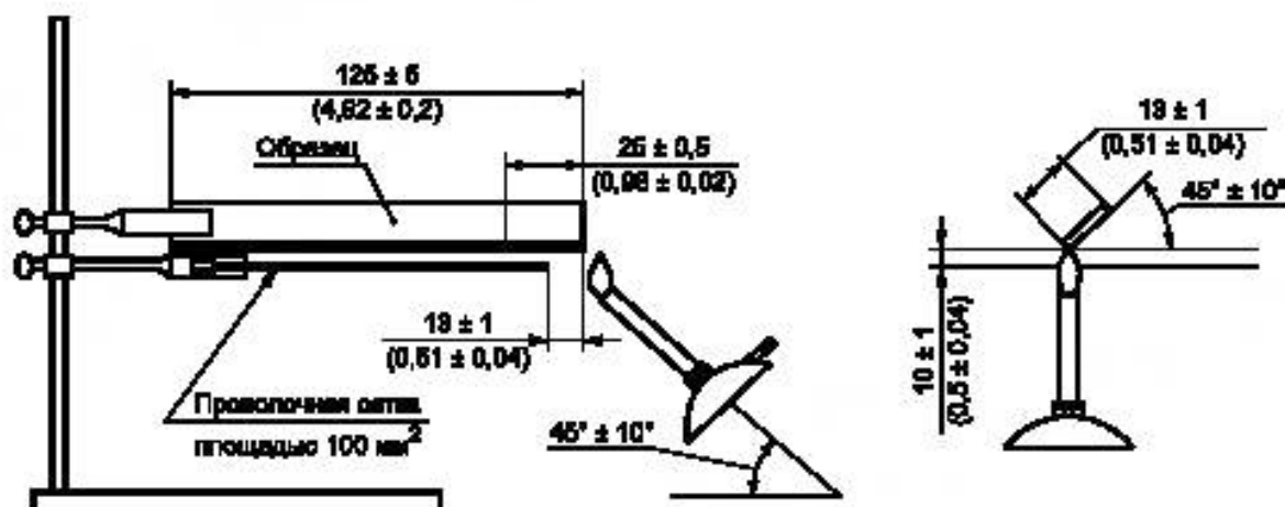
Рисунок 4 — Стенд для испытаний
