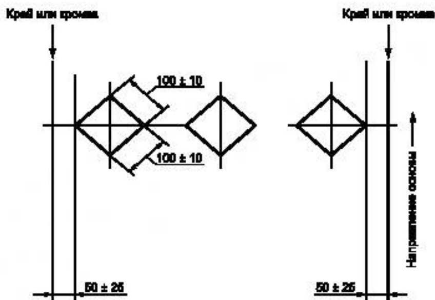
Рисунок 8 — Места вырезки образцов при определении содержания смолы
