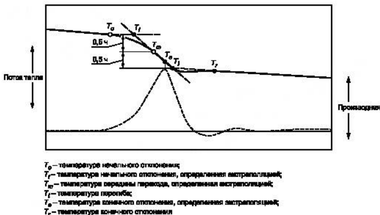
Рисунок 12 — Дифференциальная сканирующая калориметрия (характерные точки перехода состояния, связанные со стеклованием)
