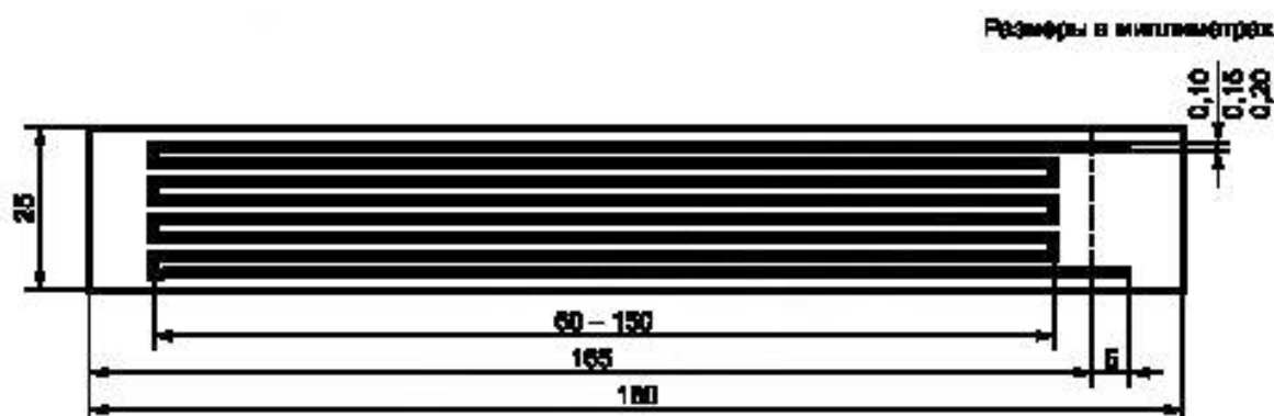
Рисунок 14 — Рисунок образца для испытаний
