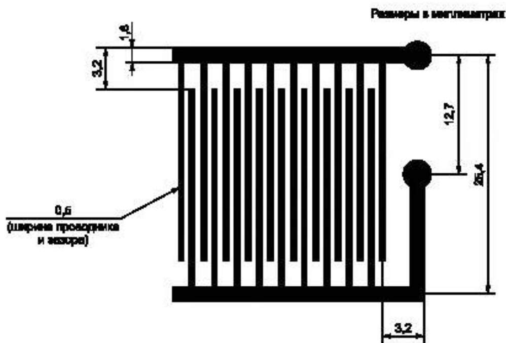
Рисунок 28 — Рисунок электродов гребенчатой формы
