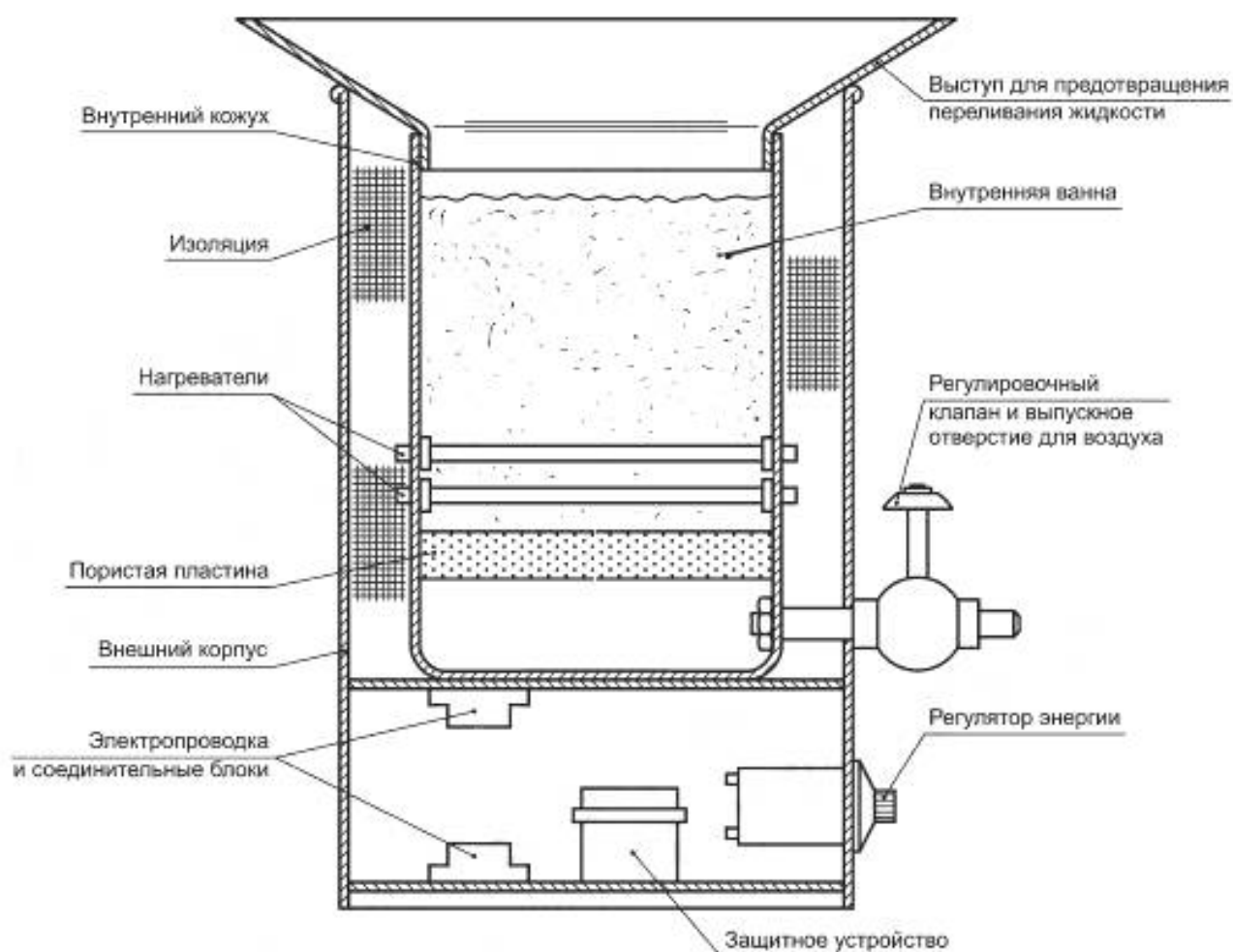
Рисунок 3 — Флюидизированная песочная баня. Принципы работы
