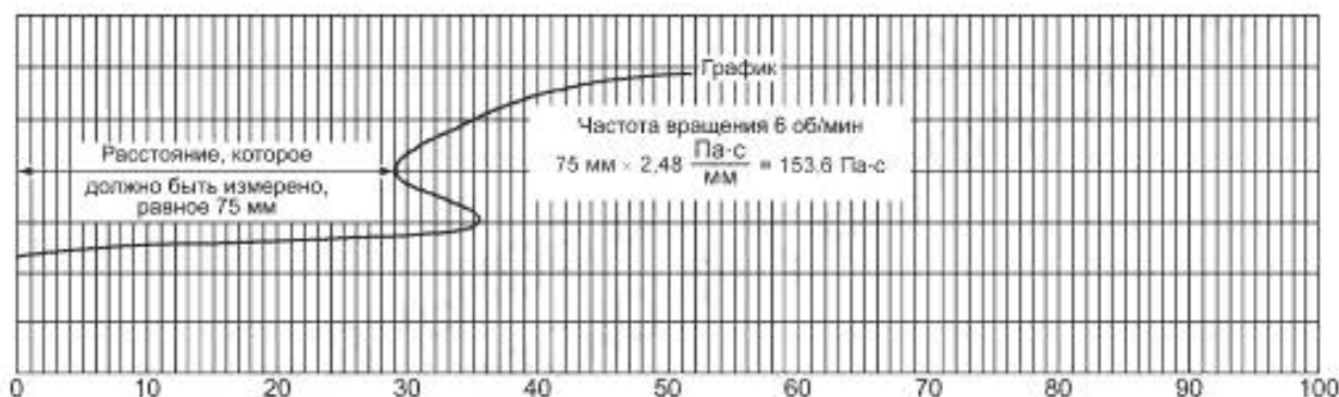
Рисунок 7 — Пример определения вязкости расплава связующего препрега
