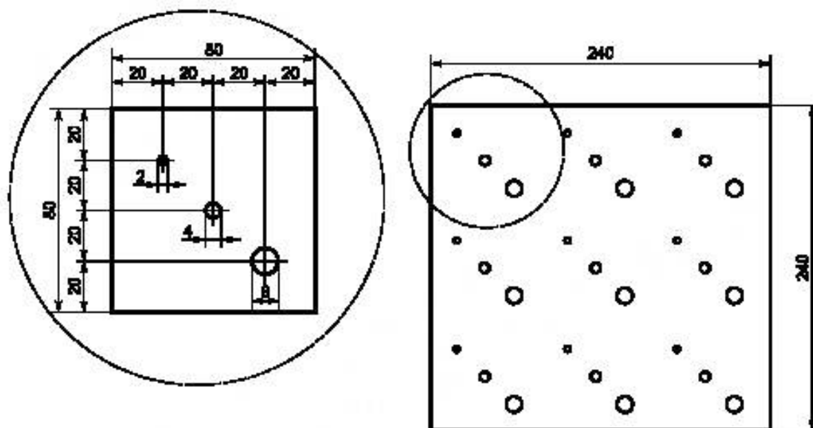
Рисунок 19 — Перфорированный тестовый рисунок для метода выдавливания
