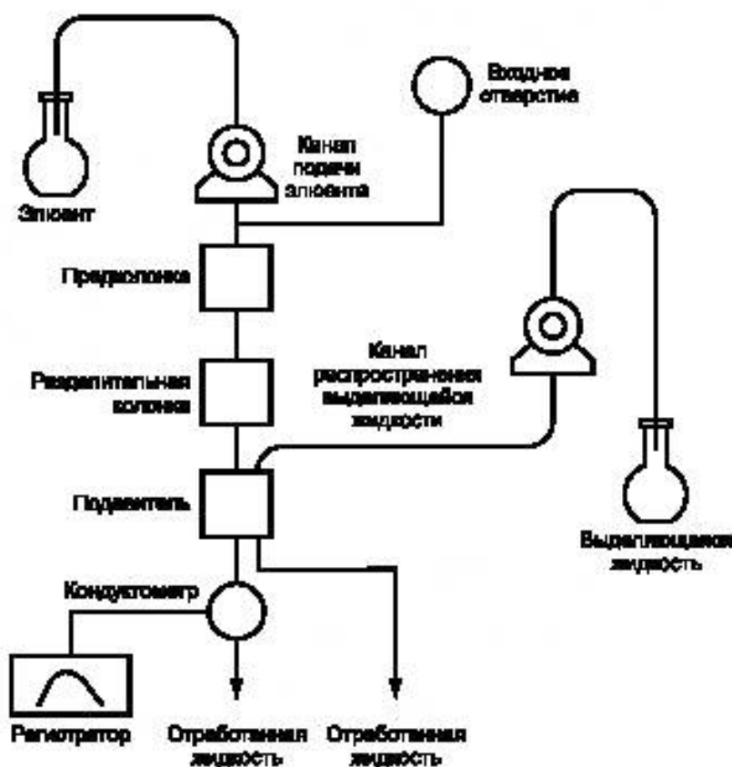
Рисунок 10 — Структура хроматографа с системой ионного обмена
