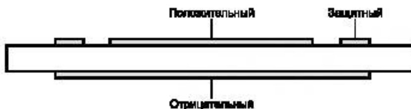
Рисунок 22 — Измерение объемного сопротивления
