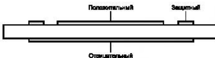
Рисунок 25 — Подсоединения электродов для измерения объемного сопротивления
