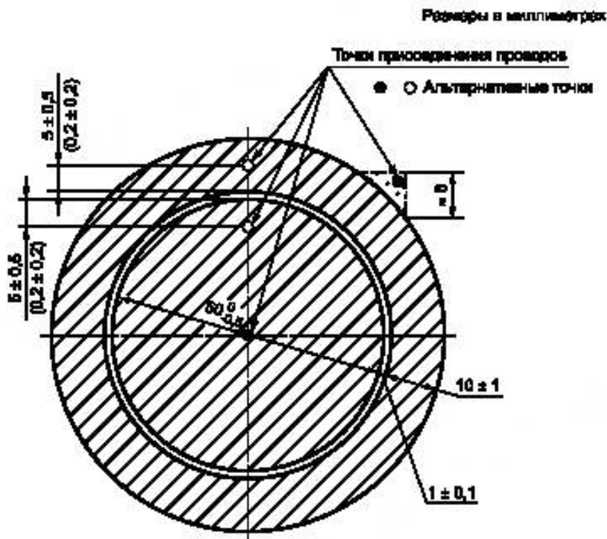
Рисунок 27 — Рисунок электродов круглой формы
