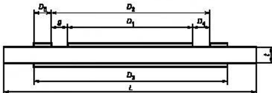
Рисунок 22а — Размеры тестового рисунка (см. таблицу 6)
