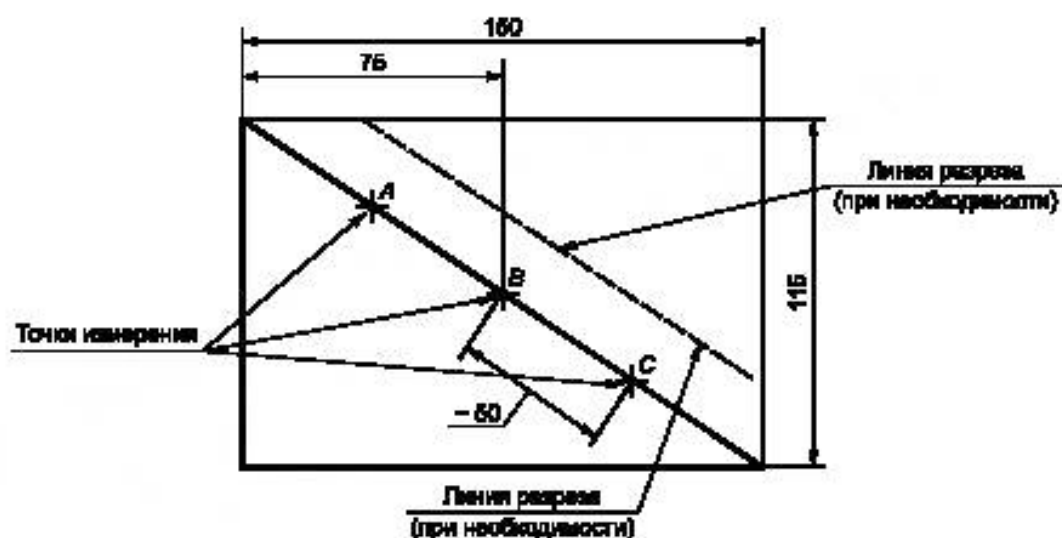
Рисунок 17 — Схема расположения точек измерения на образце
