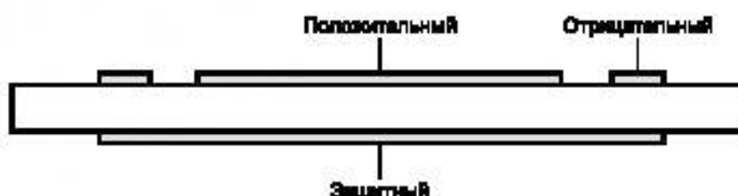
Рисунок 26 — Подсоединения электродов для измерения поверхностного сопротивления
