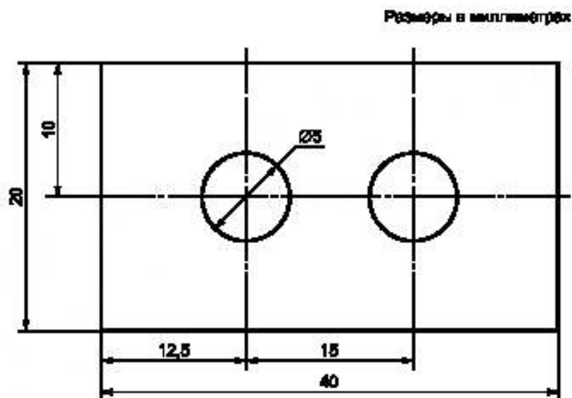
Рисунок 35 — Образец для проведения испытаний на сопротивление изоляции
