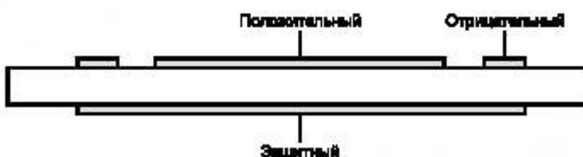
Рисунок 23 — Измерение поверхностного сопротивления
