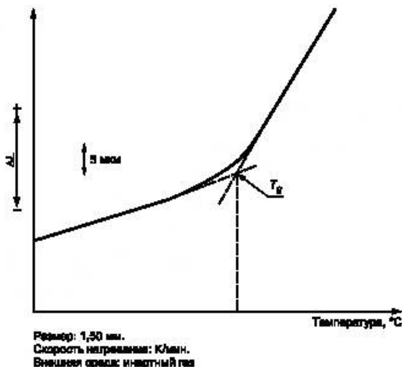
Рисунок 13 — Термомеханический анализ (в режиме расширения)
