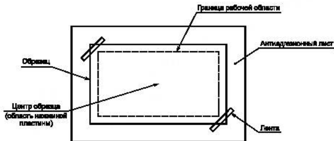
Рисунок 16 — Схема расположения образца перед прессованием
