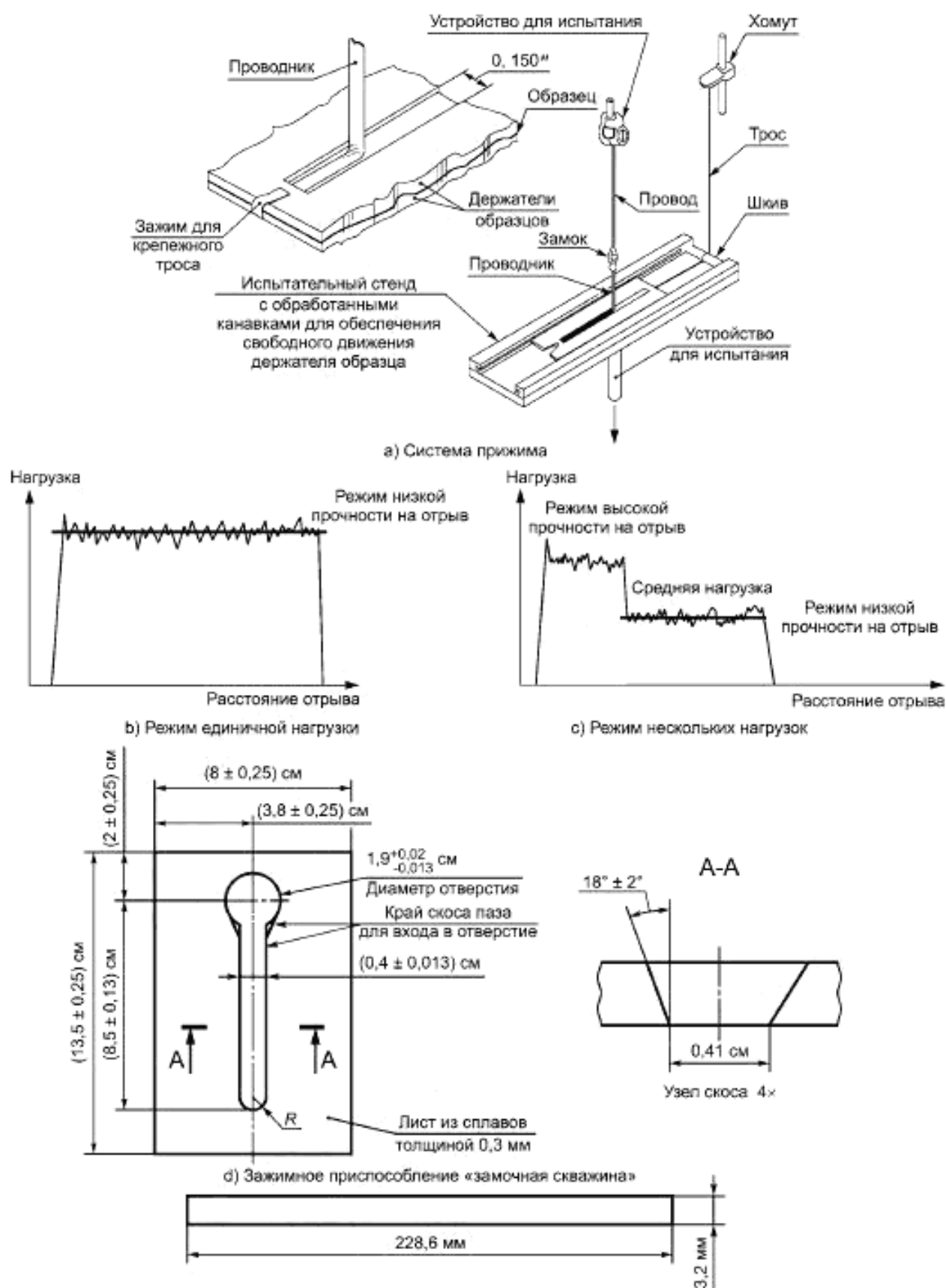
Рисунок 5 — Медная фольга для испытания на отрыв
