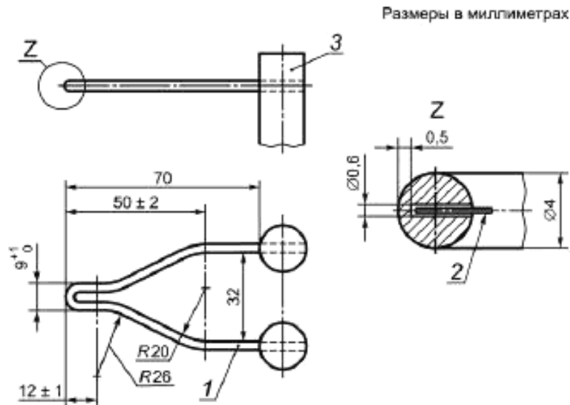
Ключ: 1 — проволока, паяная твердым припоем на позиции 3; 2 — термопара; 3 — штырь.
