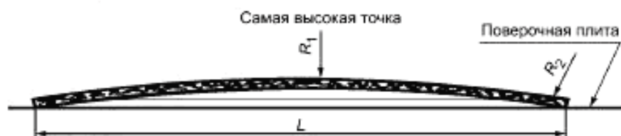
Рисунок 8 — Схема проведения измерения изгиба
