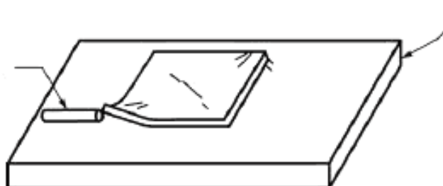
Рисунок 12 — Измерение скручивания
