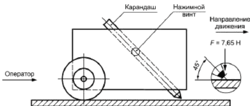
Рисунок 14 — Держатель карандашей
