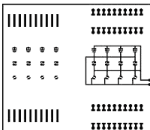
Рисунок 24 — Рисунки кнопочной панели
