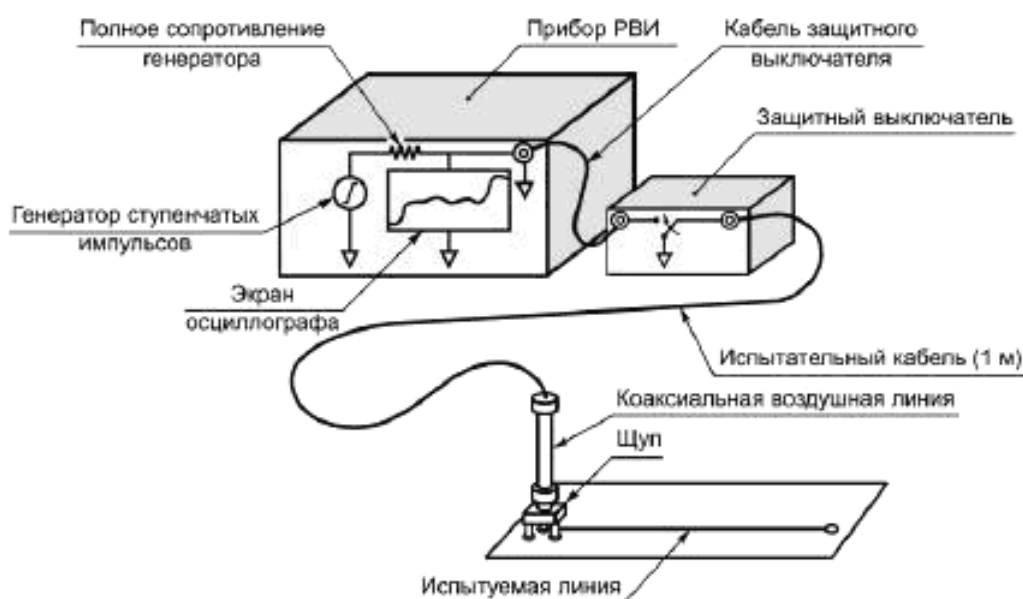
Рисунок 18 — Вариант схемы испытания
