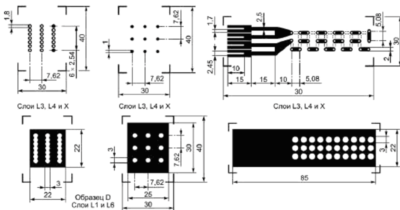
b) Расположение образцов для испытания
