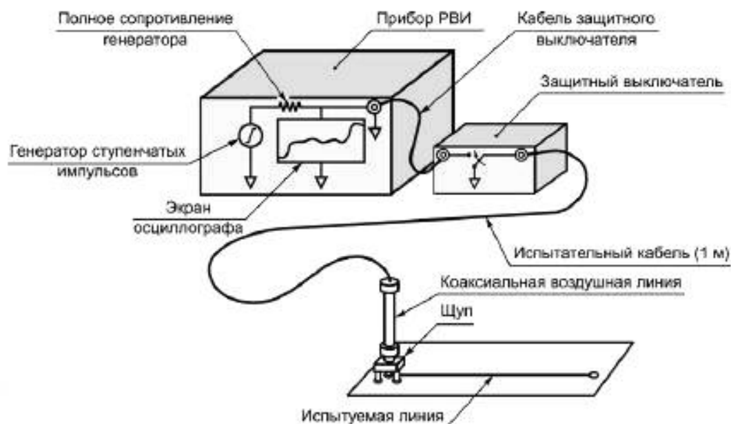
Рисунок 18 — Вариант схемы испытания
