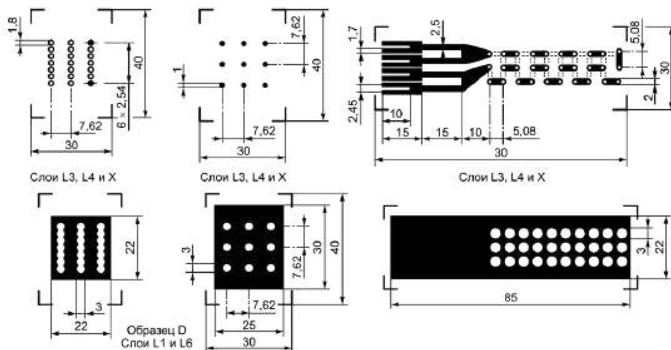
b) Расположение образцов для испытания
