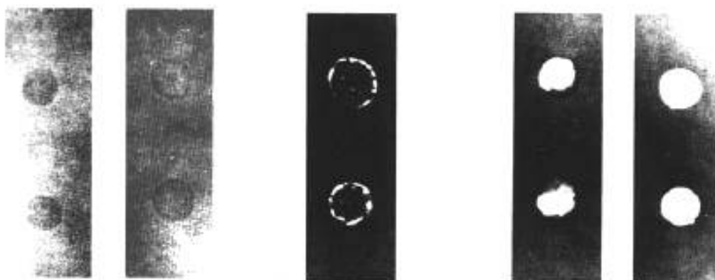
Рисунок 4 — Классификация типов флюса по результатам испытания «медное зеркало»
