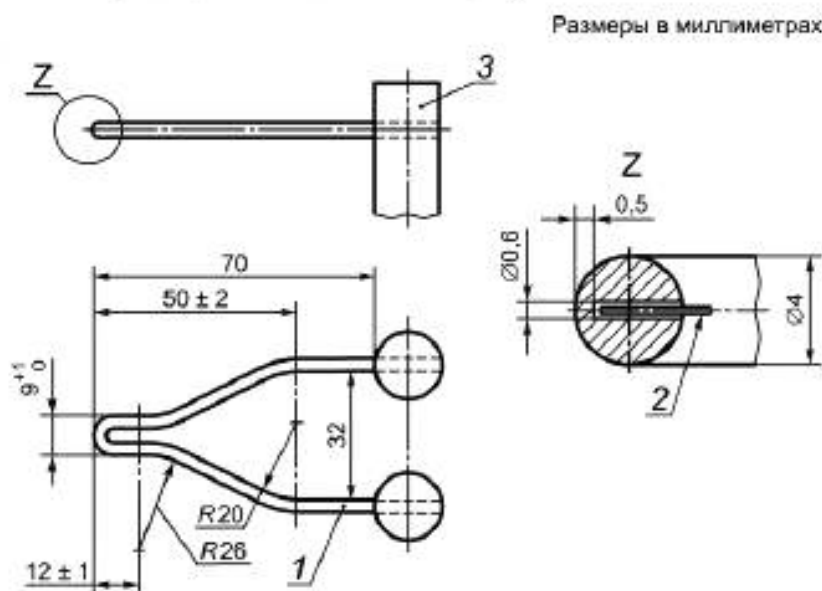
Рисунок 1 — Раскаленная проволока
