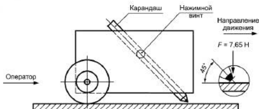
Рисунок 14 — Держатель карандашей
