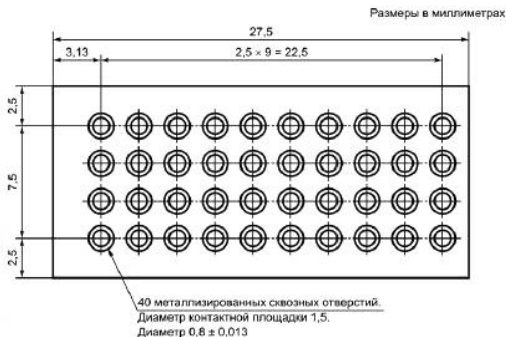
Рисунок 30 – Рекомендуемый образец для испытания металлизированных сквозных отверстий
