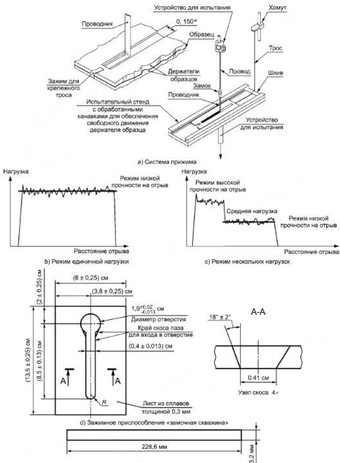
Рисунок 5 — Медная фольга для испытания на отрыв
