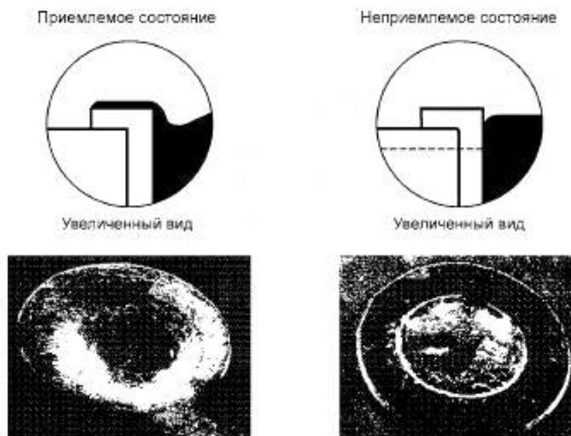
Рисунок 32 — Качество смачивания металлизированных сквозных отверстий припоем
