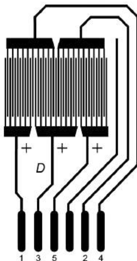
Рисунок 28 — Типовой рисунок «Гребенка»
